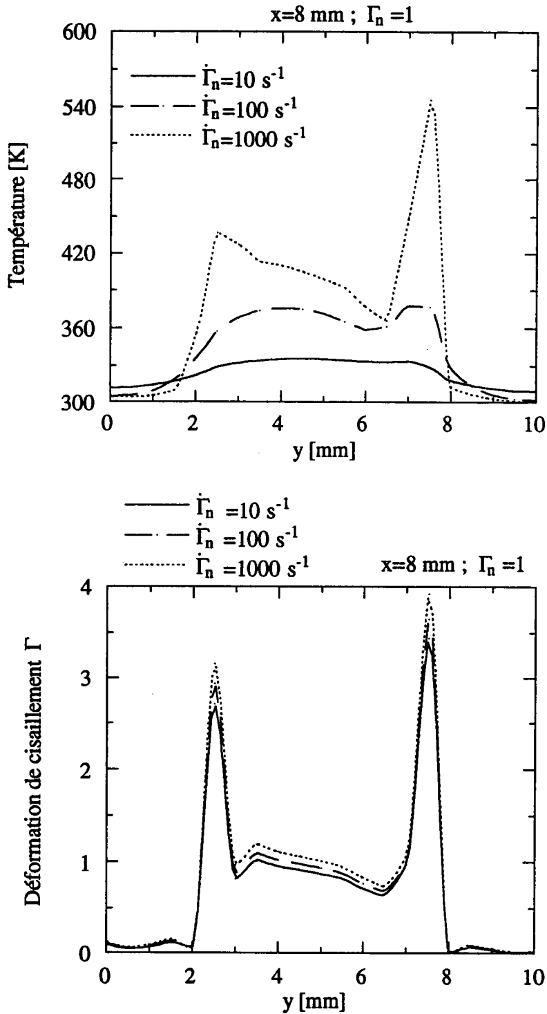
Figure IV-8. Évolution de la température et de la déformation de cisaillement le long de l'axe y d'abscisse x=8\text{ mm} pour une éprouvette en acier pour différentes vitesses de déformation nominales .
