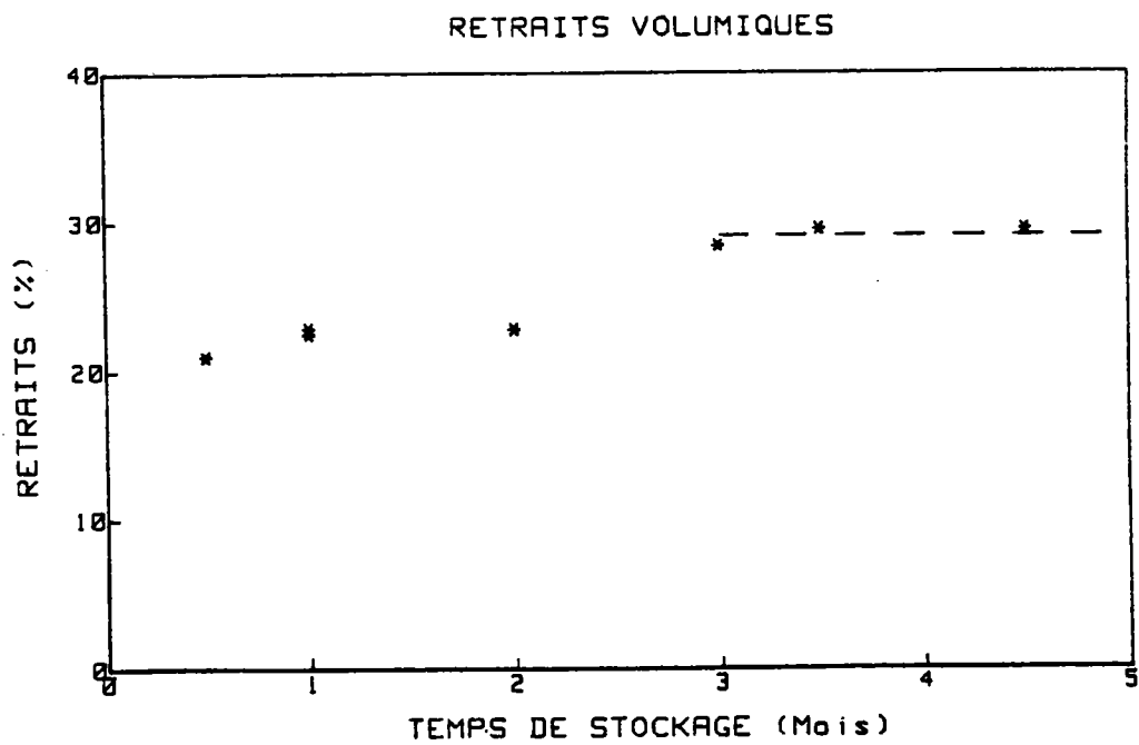
Figure 38 : Retraits volumiques des éprouvettes de flexion en colle+ fibre.
