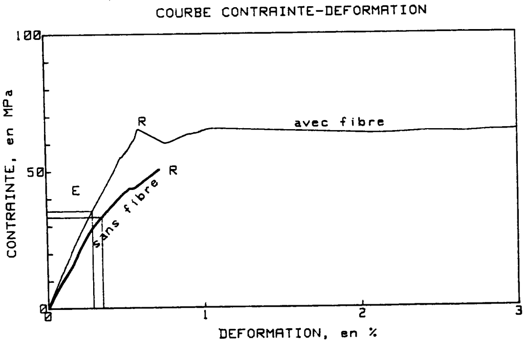
Figure 46 : Courbes contrainte-déformation d'un L.C.R. 2 couches et d'un lamellé-collé traditionnel.
