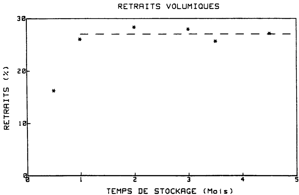
Figure 25 : Retraits volumiques des éprouvettes de traction en colle + fibre en fonction du temps de stockage.
