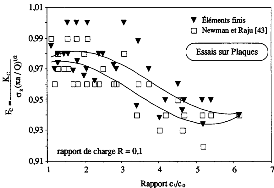
Figure III.21. Variation du facteur de correction de géométrie F_C en surface en fonction du rapport c_i/c_0 , pour un rapport de charge R = 0,1 et dans le cas d'une plaque.
