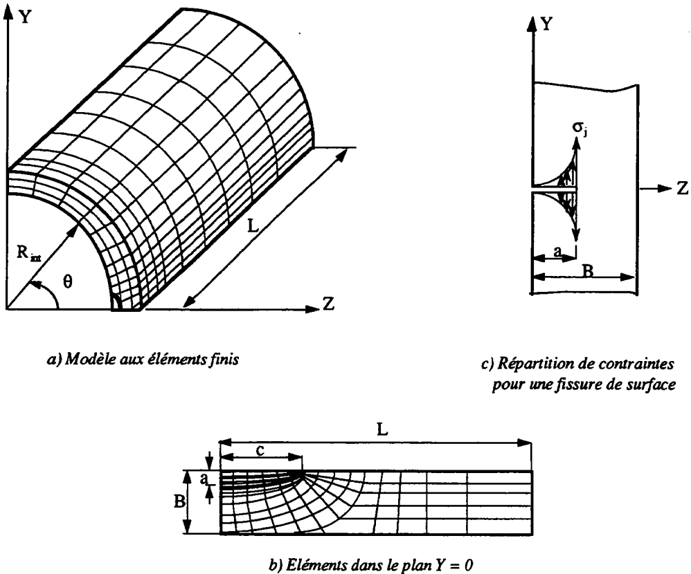
Figure I.9. Schéma représentatif d'une modélisation aux éléments finis d'un quart de tube soumis à une pression interne [31 et 32].
