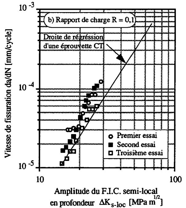
Figures (III.10a - b). Courbes de vitesse de fissuration sur plaques, rapport de charge R = 0,1 .
