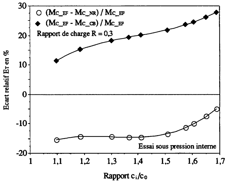
Figure III.27. Variation de l'écart relatif E_T % sur la valeur des facteurs de correction de géométrie M_C en profondeur en fonction de c_i/c_0 , pour rapport de charge R = 0,3 résultats sur un tube.
