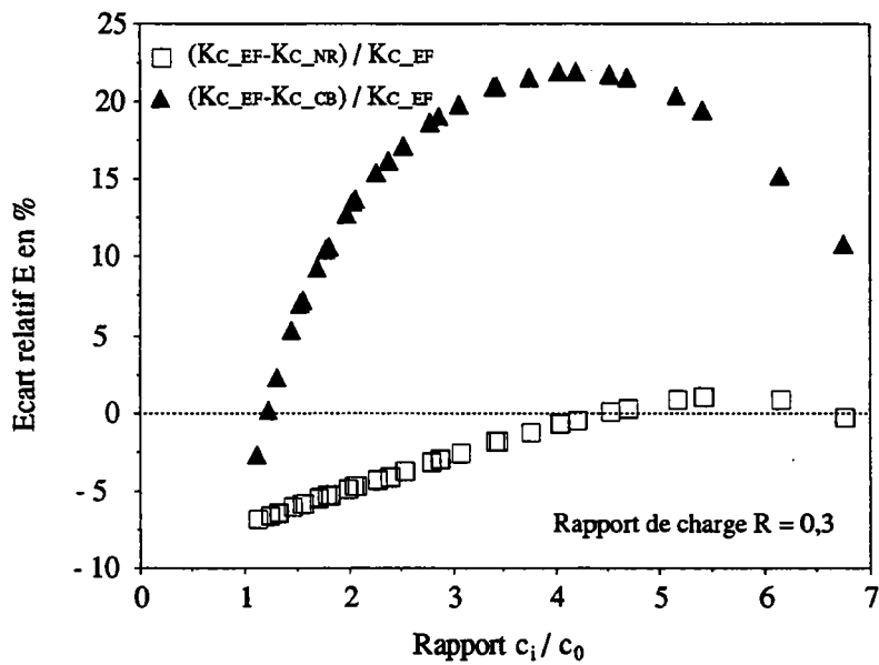
Figure III.7d. Variation de l'écart relatif sur la valeur du facteur d'intensité de contraintes en surface en fonction du rapport c_i/c_0 , pour un rapport de charge R = 0,3 .
