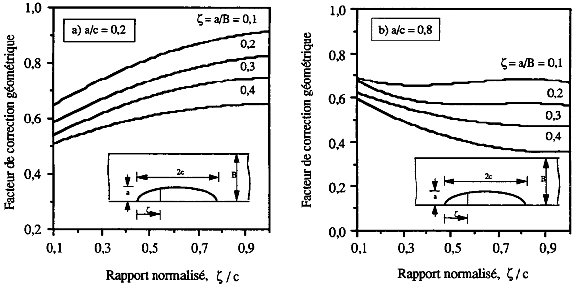
Figures (I.26a et b). Facteur de forme géométrique en fonction du rapport normalisé \xi/c pour un chargement de flexion selon [42].
