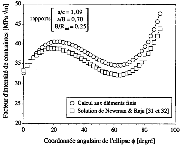
Figure III.16c. Comparaison du facteur d'intensité de contraintes local obtenu par la solution de Newman & Raju et par la méthode aux éléments finis, pour les conditions de géométrie a/c = 1,09 ; a/B = 0,70 et B/R_{int} = 0,25 .
