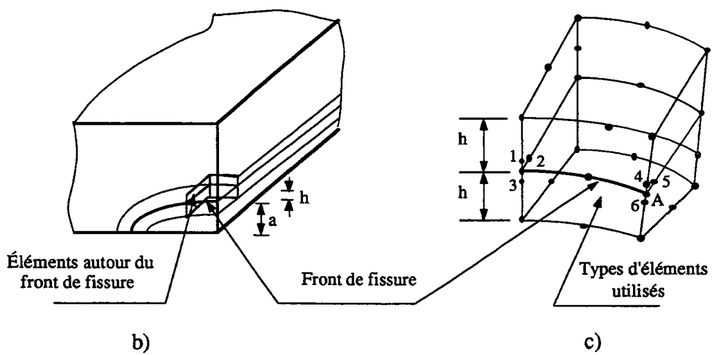
Figure II.12. (b) Éléments autour du front de fissure ; (c) les nœuds centraux situés à une position d'un 1/4 de la maille du front de fissure (nœuds 1 à 6) et appartiennent à deux éléments du front de fissure.
