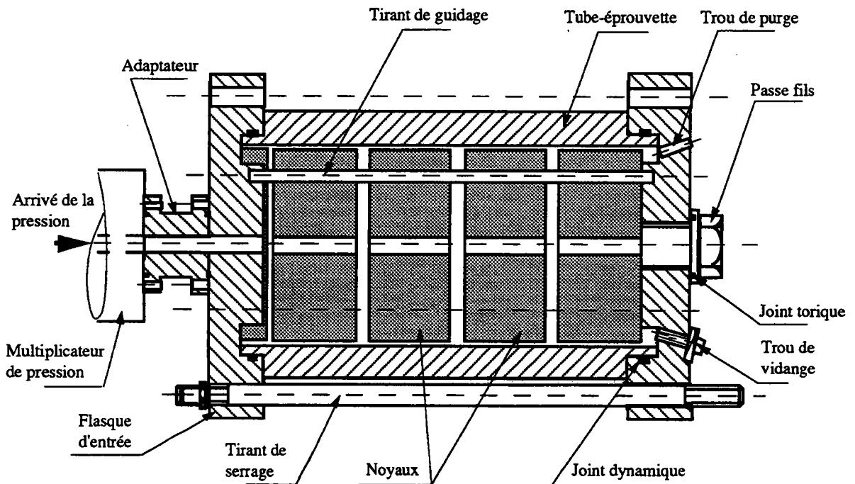
Figure II.7. Schéma du montage tube-épreuve.
