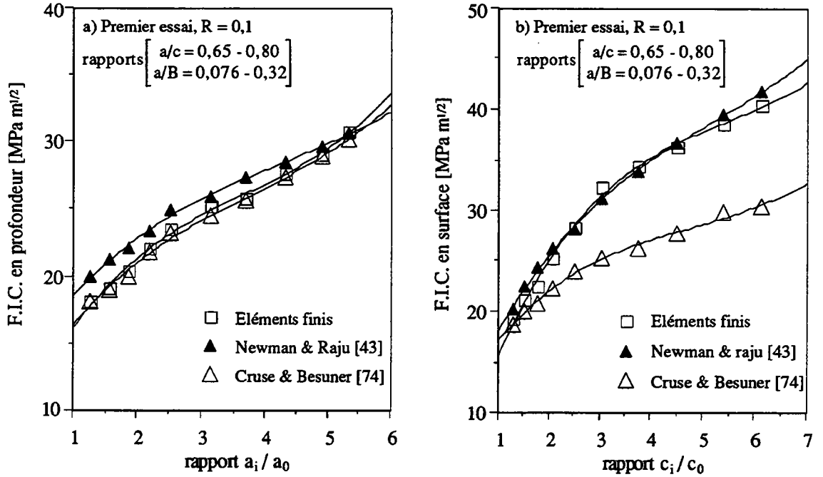
Figure III.5a. Variation du facteur d'intensité de contraintes local et semi-local a) en profondeur en fonction du rapport a_i/a_0 , b) en surface en fonction du rapport c_i/c_0 pour un rapport de charge R = 0,1 .
