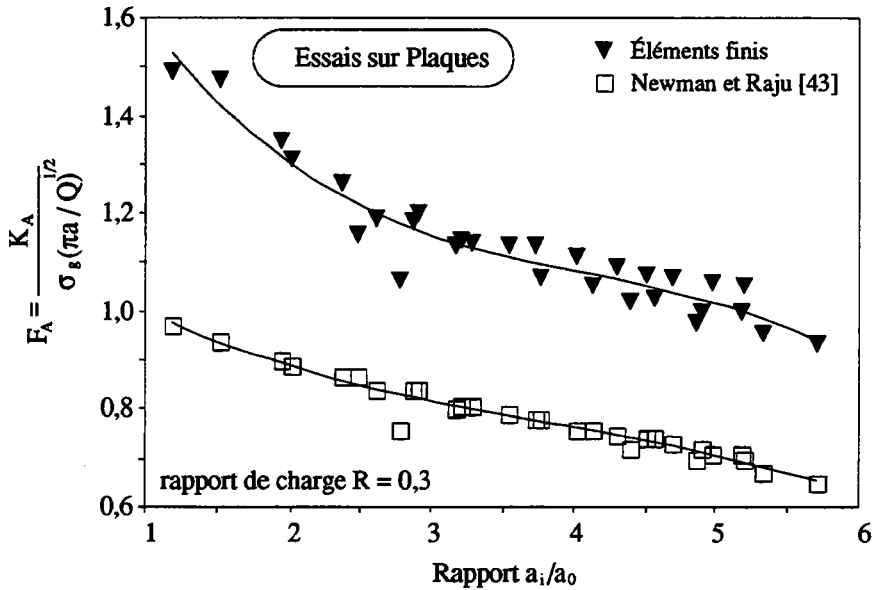
Figure III.22. Variation du facteur de correction de géométrie F_A en profondeur en fonction du rapport c_i/c_0 , pour un rapport de charge R = 0,3 et dans le cas d'une plaque.
