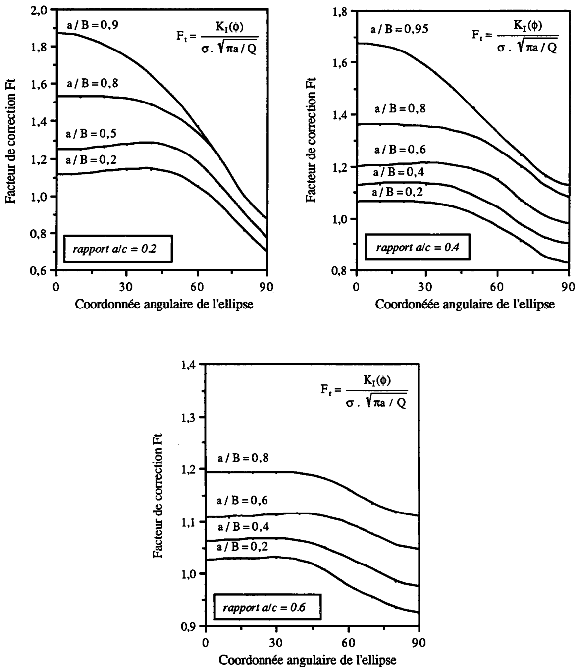
Figure I.15. Résultats de Smith & Sorensen pour un défaut de forme semi-elliptique dans une plaque soumise à une traction simple [51].
