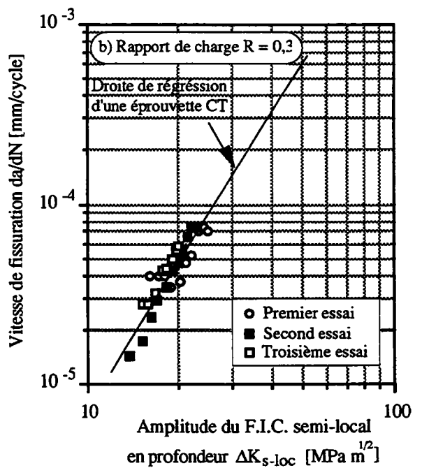
Figures (III.11a - b). Courbes de vitesse de fissuration sur plaques, rapport de charge R = 0,3 .
