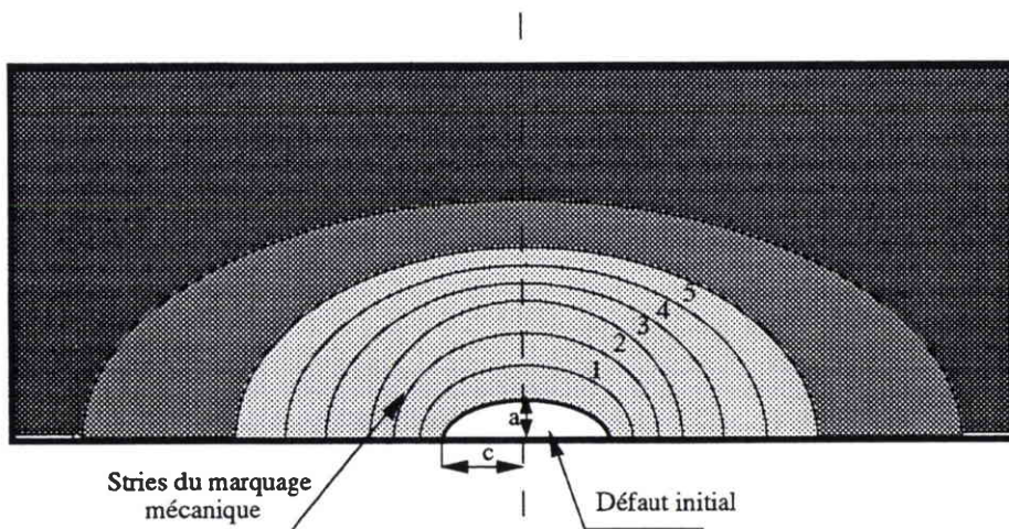
Figure III.2. Schéma représentatif du faciès de rupture après marquage sur plaques.
