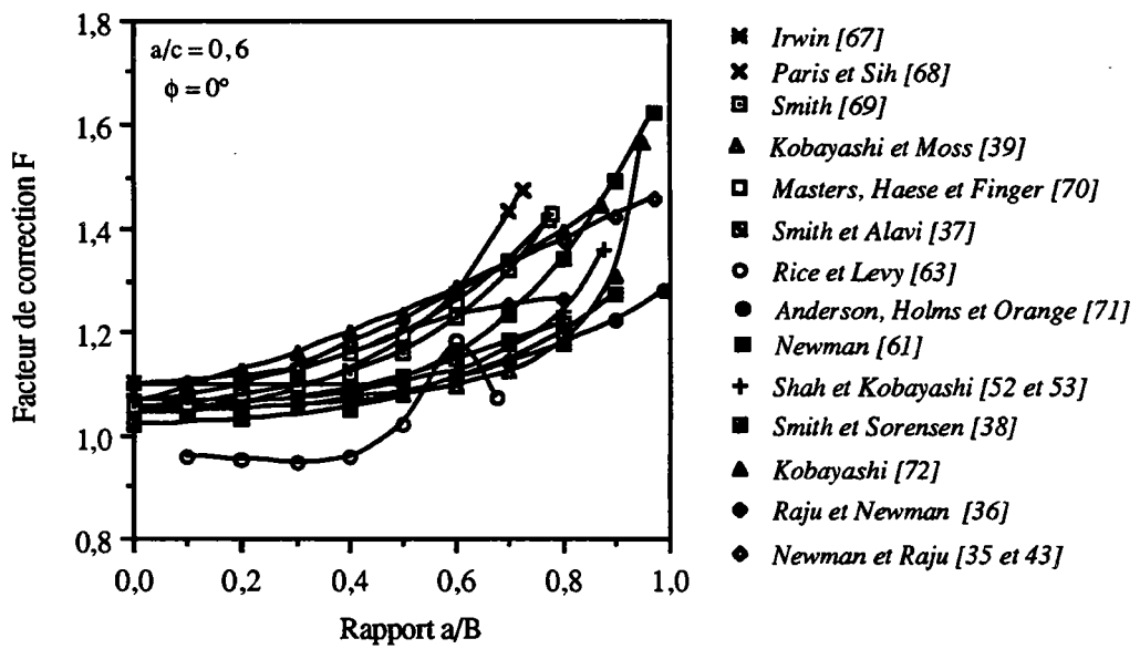
Figure I.22. Comparaison de la variation du facteur de correction F présentée par différents auteurs au point le plus profond \phi = 0^\circ et pour le rapport a/c = 0,6 [62].
