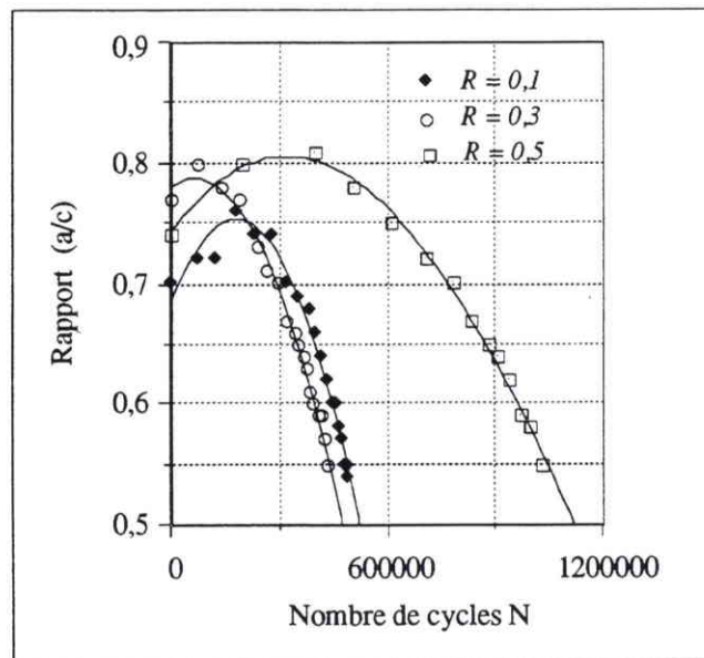
Figure III.1. Évolution du rapport (a/c) en fonction du nombre de cycles N pour trois rapports de charge R , dans le cas des plaques.
