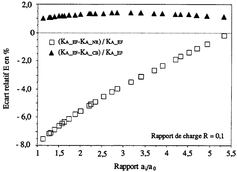
Figure III.7a. Variation de l'écart relatif sur la valeur du facteur d'intensité de contraintes en profondeur en fonction du rapport a_i/a_0 , pour un rapport de charge R = 0,1 .
