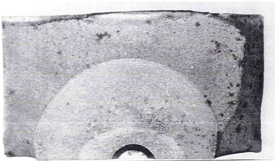
Photo III.3. Faciès de rupture d'un tube sollicité en pression interne.
