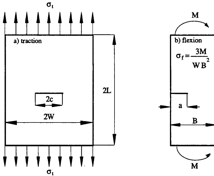
Figure I.13. Représentation schématique d'une plaque sollicitée en traction et en flexion.
