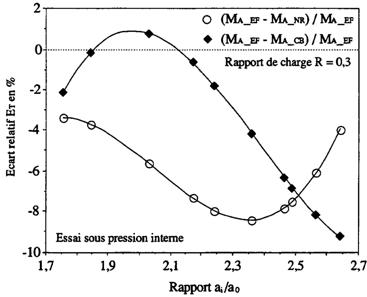
Figure III.26. Variation de l'écart relatif E_T % sur la valeur des facteurs de correction de géométrie M_A en profondeur en fonction de a_i/a_0 , pour rapport de charge R = 0,3 résultats sur un tube.
