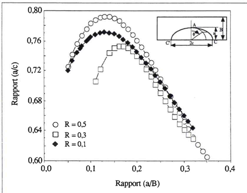
Figure III.3. Évolution de la forme de fissure dans le cas des plaques.
