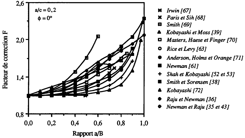
Figure I.21. Comparaison de la variation du facteur de correction F présentée par différents auteurs au point le plus profond \phi = 0^\circ et pour le rapport a/c = 0,2 [62].
