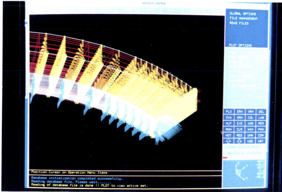
Figure A3. Maillage du tube sous pression interne
