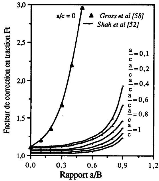
Figure I.18. Comparaison des résultats de Shah & Kobayashi avec ceux de Gross & Srawley & Brown en traction simple [23].
