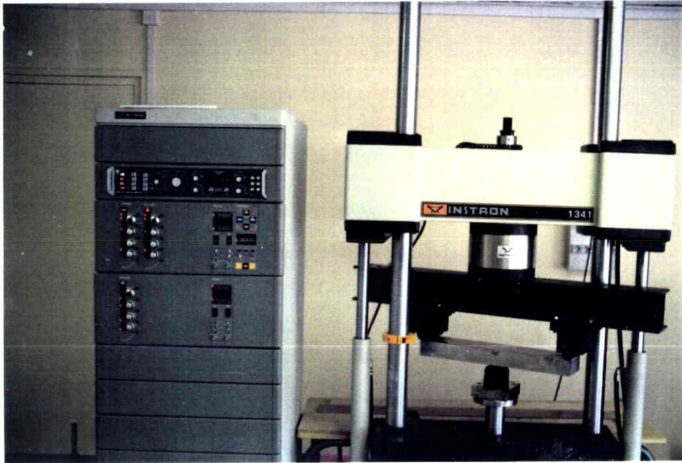
Photo II.1. Machine d'essai et dispositif de fissuration sur plaques.
