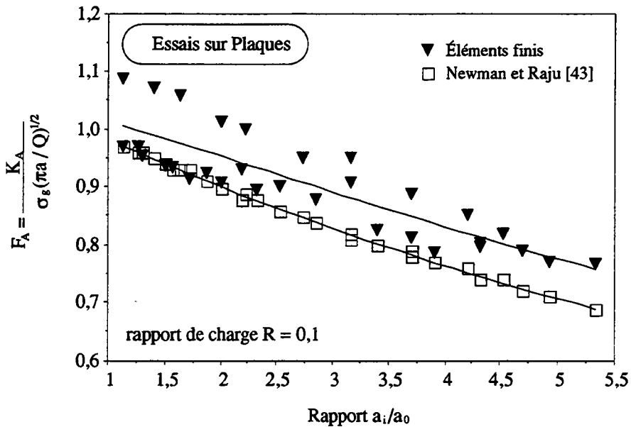
Figure III.20. Variation du facteur de correction de géométrie F_A en profondeur en fonction du rapport a_i/a_0 , pour un rapport de charge R = 0,1 et dans le cas d'une plaque.
