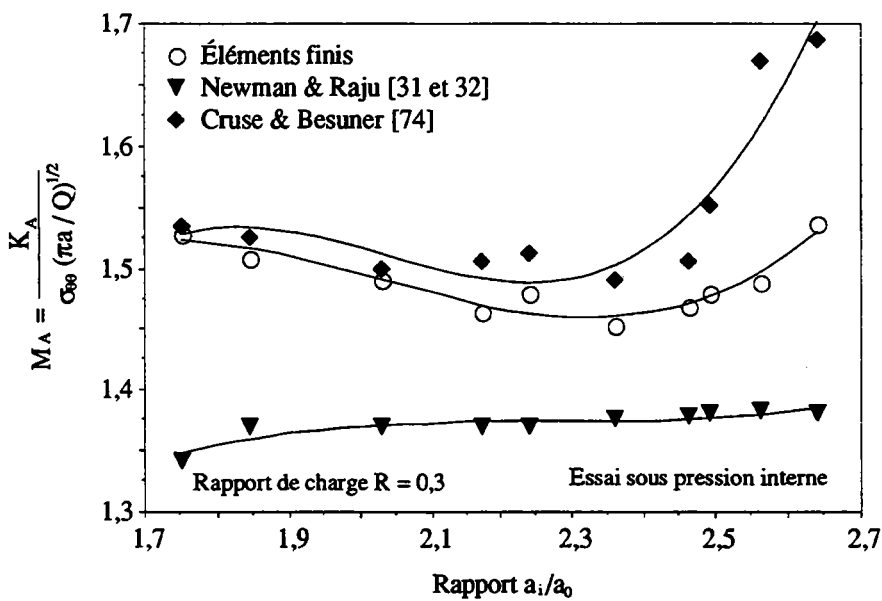
Figure III.24. Variation des facteurs de correction de géométrie M_A en profondeur en fonction de a_i/a_0 , pour un rapport de charge R = 0,3 résultats sur un tube.
