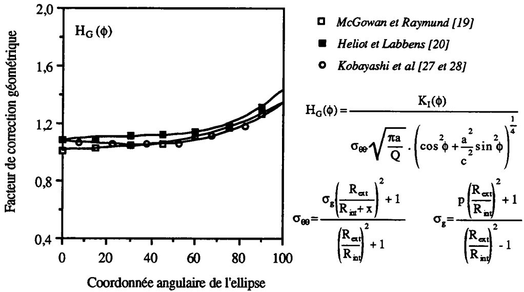
Figure I.8a. Courbes des facteurs de correction géométrique données par différents auteurs, pour les rapports a/B = 0,25 , a/c = 1/3 et B/R_{int} = 0,1 [19].
