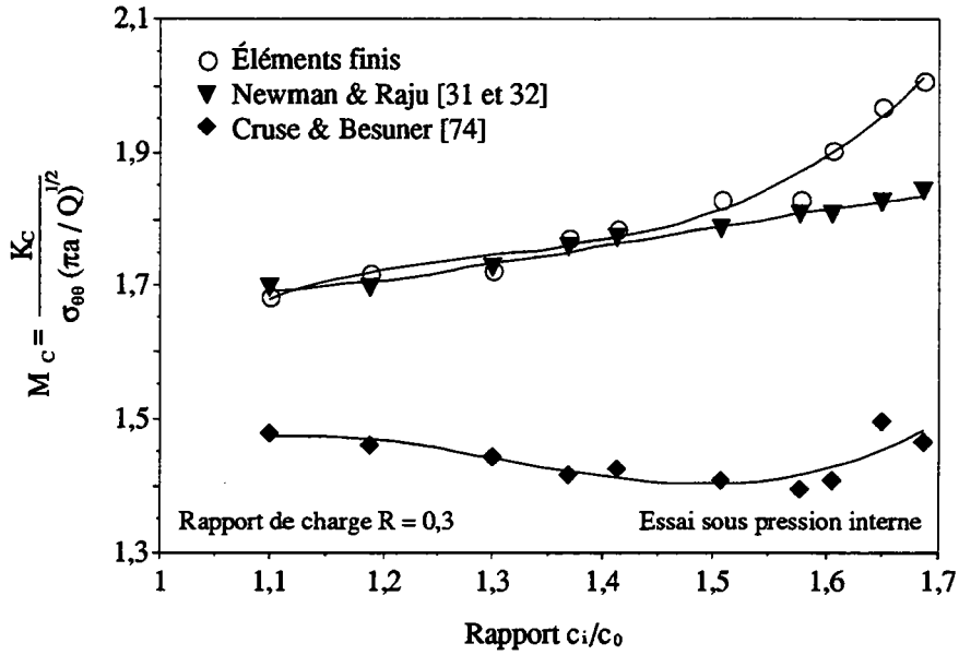
Figure III.25. Variation des facteurs de correction de géométrie M_C en surface en fonction de c_i/c_0 , pour un rapport de charge R = 0,3 résultats sur un tube.
