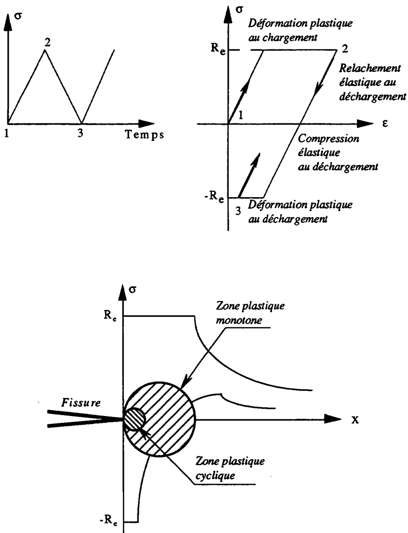
Figure 1.3. Mécanisme de la plastification cyclique à fond de fissure de fatigue selon Rice [5].
