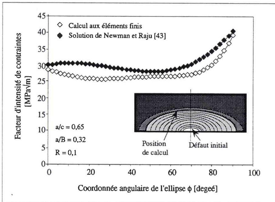
Figure III.4d. Comparaison du F.I.C. local obtenu par la solution de Newman & Raju et par la méthode aux éléments finis pour a/c = 0,65 et a/B = 0,32 .
