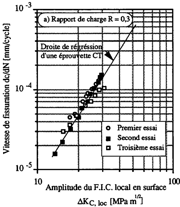
Figures (III.9a et b). Courbes de vitesse de fissuration sur plaques, rapport de charge R = 0,3 .
