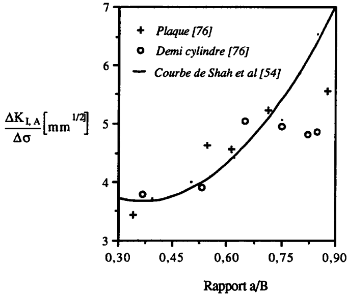
Figure I.29. Comparaison entre les résultats expérimentaux de Sommer & Ratwani [76] et les résultats théoriques de Shah et Kobayashi [54].
