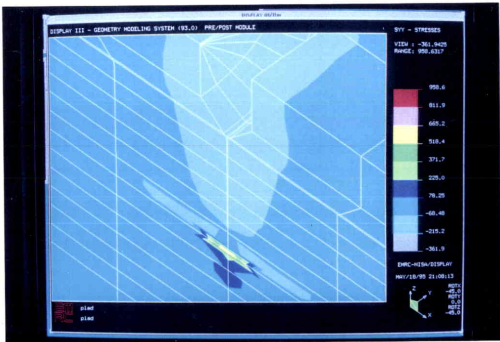
Figure A6. Concentration de contraintes au point le plus profond dans une plaque en flexion trois points
