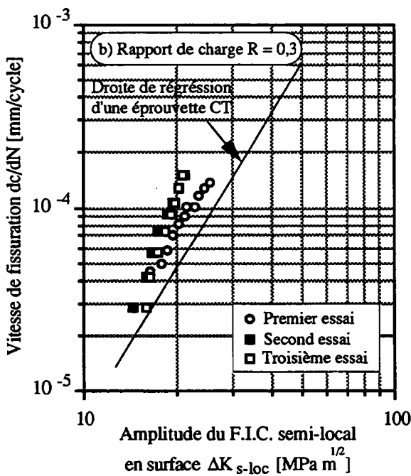
Figures (III.11a - b). Courbes de vitesse de fissuration sur plaques, rapport de charge R = 0,3 .
