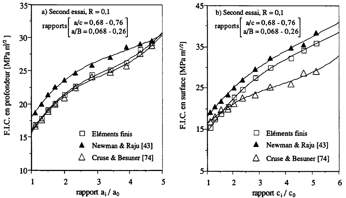
Figure III.5b. Variation du facteur d'intensité de contraintes local et semi-local a) en profondeur en fonction du rapport a_i/a_0 , b) en surface en fonction du rapport c_i/c_0 pour un rapport de charge R = 0,1 .
