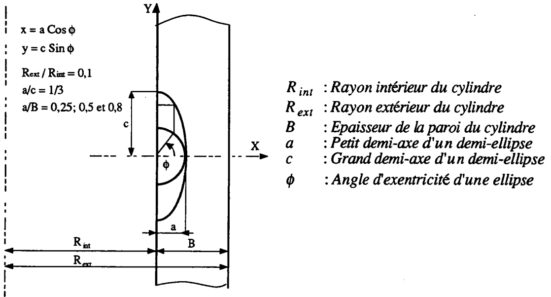
Figure I.4. Défaut semi-elliptique dans un cylindre pressurisé [27 et 28].
