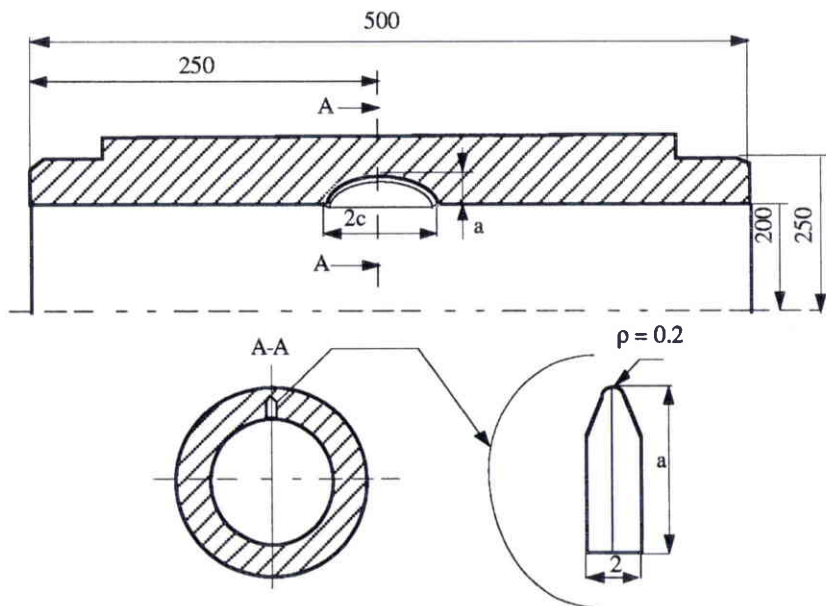
Figure II.9. Dimensions du tube-éprouvette.
