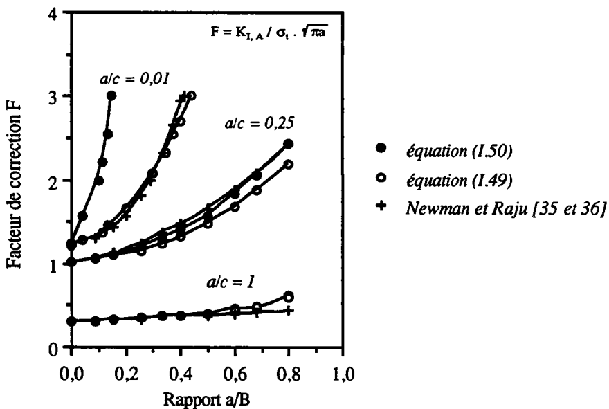
Figure I.20. Comparaison de différentes solutions du facteur de correction F en traction, valeurs données en référence [60].
