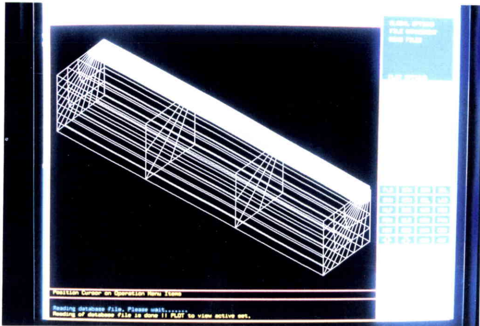
Figure A5. Modélisation d'un quart d'une plaque en flexion trois points
