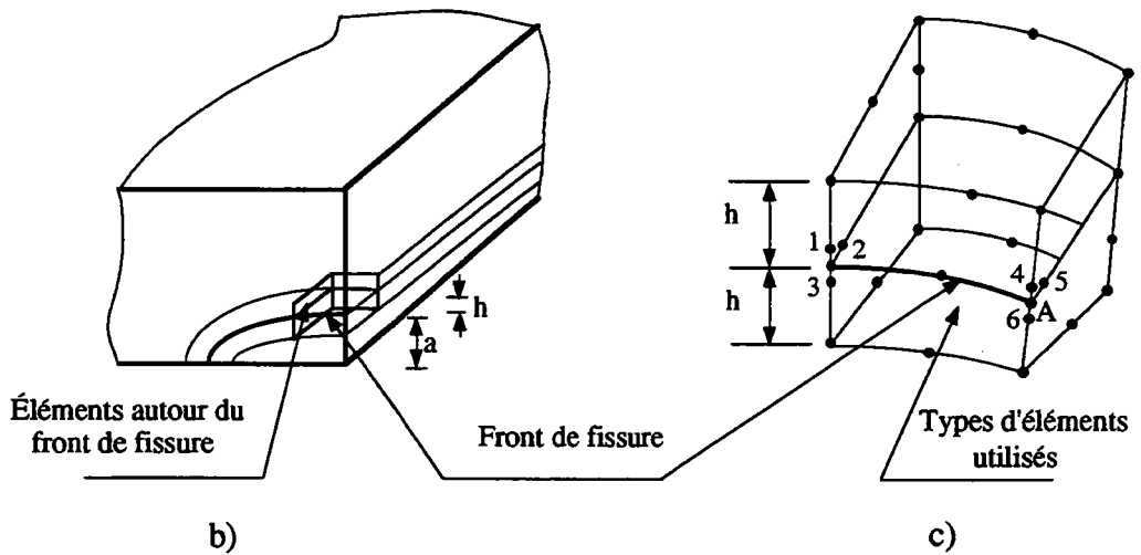
Figure II.11 (b) Éléments autour du front de fissure ; (c) les nœuds centraux situés à une position d'un 1/4 de la maille du front de fissure (nœuds 1 à 6) et appartiennent à deux éléments du front de fissure.
