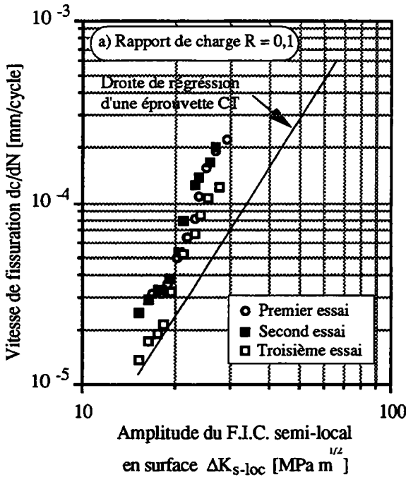
Figures (III.10a - b). Courbes de vitesse de fissuration sur plaques, rapport de charge R = 0,1 .
