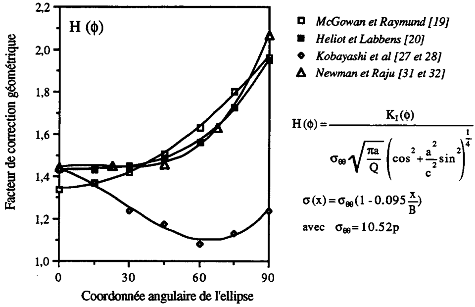
Figure I.11. Courbes du facteur de correction H(\phi) données par différents auteurs, pour les rapports a/B = 0,8 , a/c = 1/3 et B/R_{int} = 0,1 .
