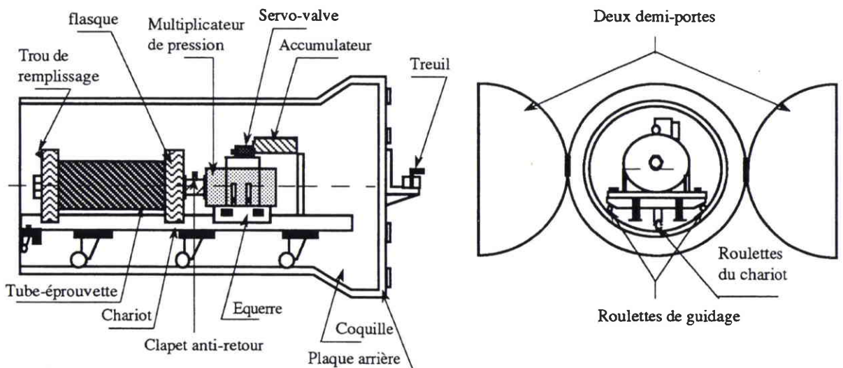
Figure II.8. Schéma de l'ensemble du dispositif de fissuration et de la coquille de protection.
