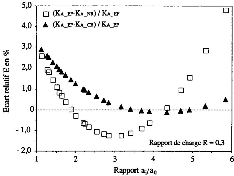
Figure III.7c. Variation de l'écart relatif sur la valeur du facteur d'intensité de contraintes en profondeur en fonction du rapport a_i/a_0 , pour un rapport de charge R = 0,3 .
