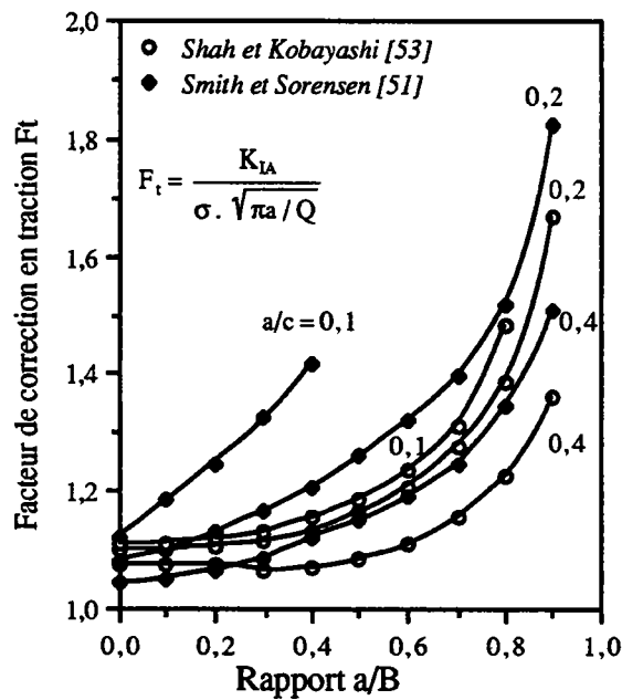
Figure I.19. Comparaison entre les résultats de Shah & Kobayashi et ceux de Smith & Sorensen [51].
