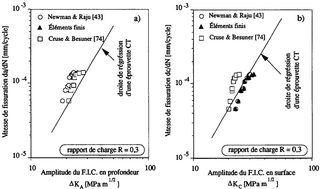
Figure III.19. Courbes de vitesse fissuration locale et semi-locale, a) au point le plus profond, b) en surface, pour un rapport de charge R = 0,3 .
