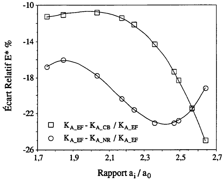
Figure III.18a. Variation de l'écart relatif E^* % sur la valeur du facteur d'intensité de contraintes en profondeur en fonction du rapport a_i/a_0 .
