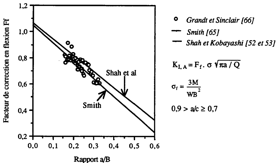
Figure I.23. Comparaison des résultats expérimentaux de Grandt & Sinclair [66] avec les résultats numériques de Smith [65] et Shah & Kobayashi [52 et 53].
