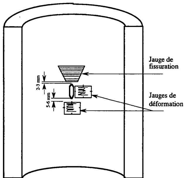
Photo II.10. Position de collage des jauges pour détecter l'amorçage et l'évolution de la propagation de la fissure de fatigue sur tube.
