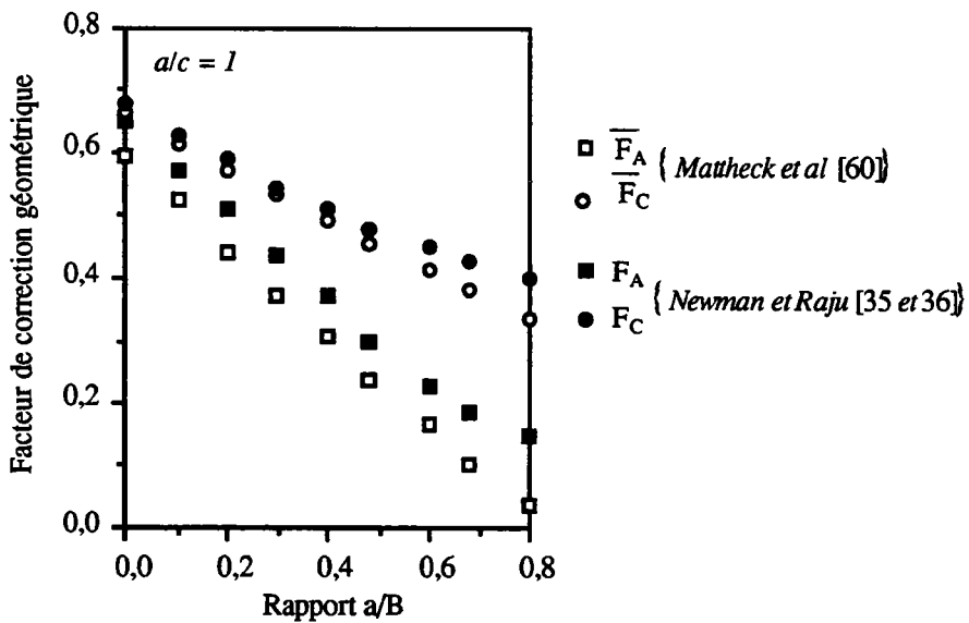
Figure (I.28a). Comparaison de différentes valeurs de F données par Mattheck & al [60] et celles de Newman & Raju [35 et 36] pour une flexion pure (rapport a/c = 1 ).
