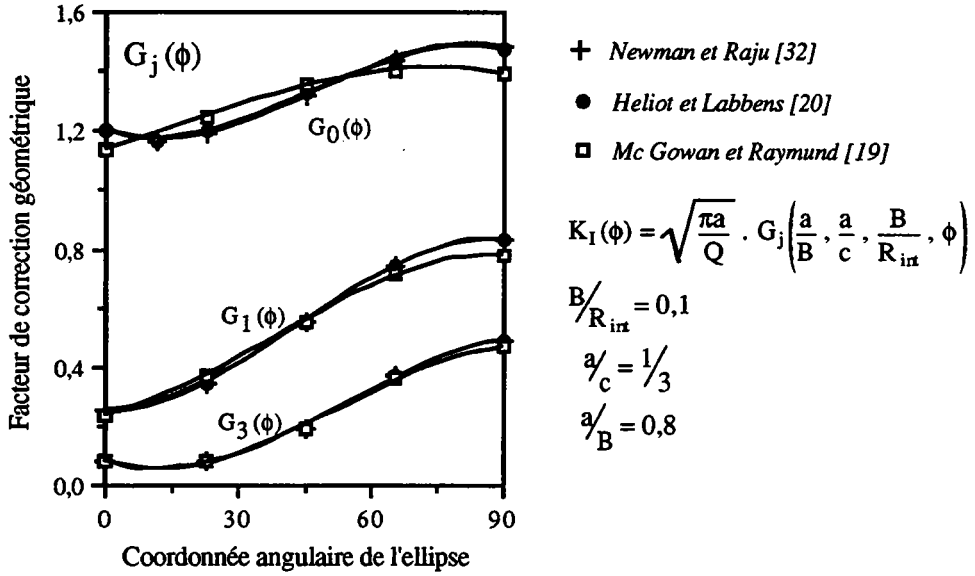
Figure I.10. Comparaison des résultats de Heliot & Labbens et McGowan & Raymund avec ceux de Raju & Newman [32].
