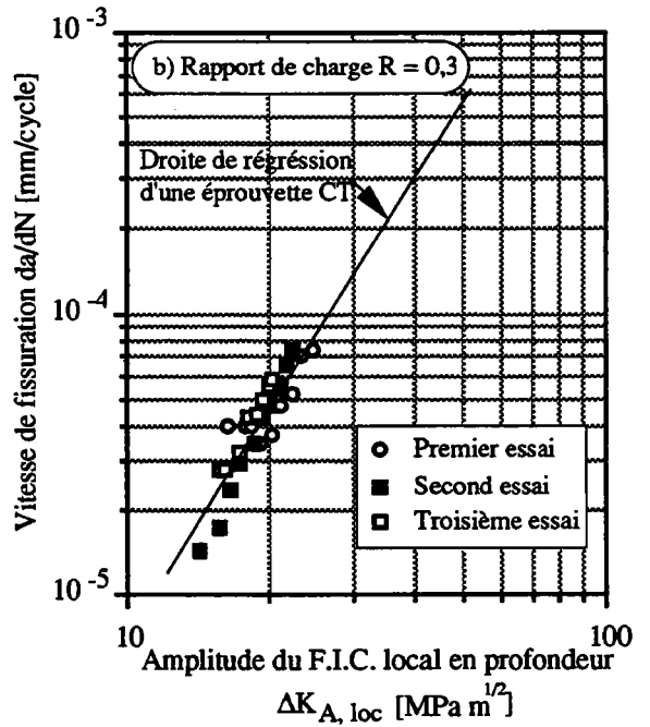
Figures (III.9a et b). Courbes de vitesse de fissuration sur plaques, rapport de charge R = 0,3 .
