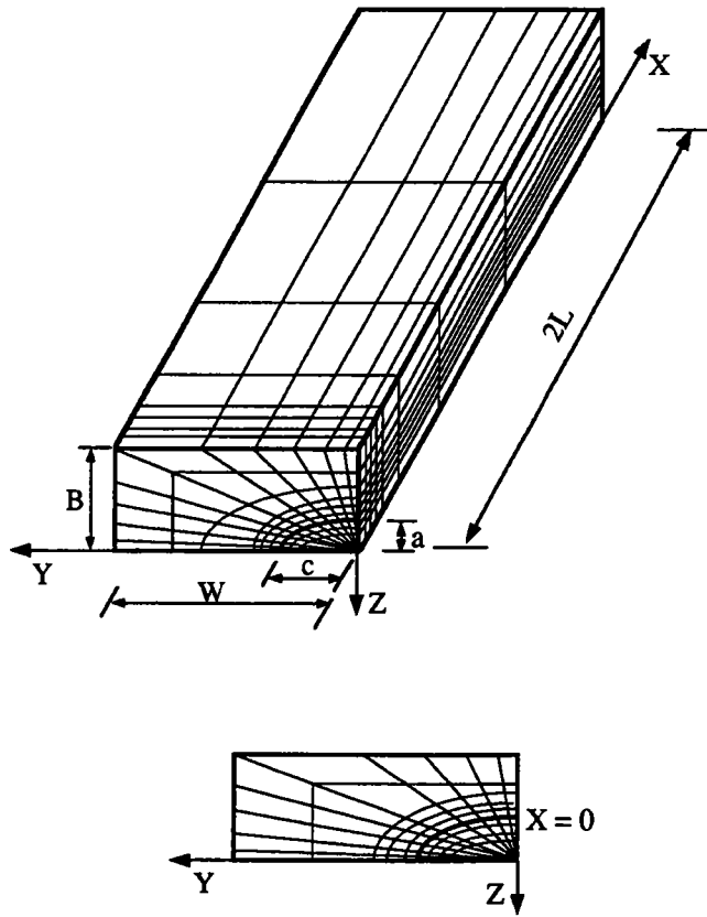
Figure II.11a. Maillage par éléments finis de la géométrie plaque.
