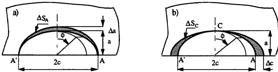
Figure I.27. Extension de la fissure pour le calcul du facteur d'intensité de contraintes moyen [60].
