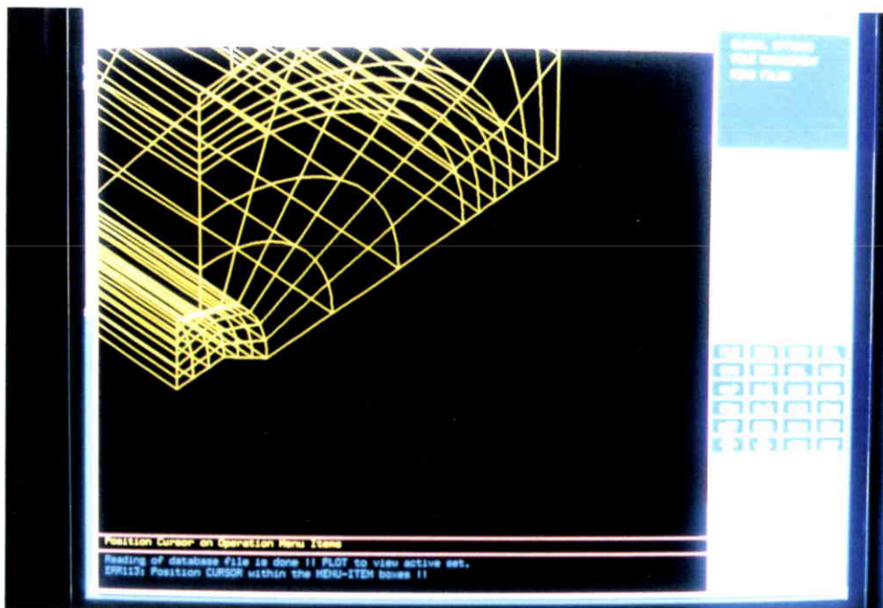
Photo III.4. Modélisation d'un tube sous pression interne.
