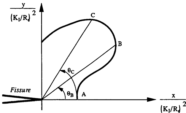
Figure I.2. Définitions des valeurs particulières de \alpha selon Banks et al [3].
