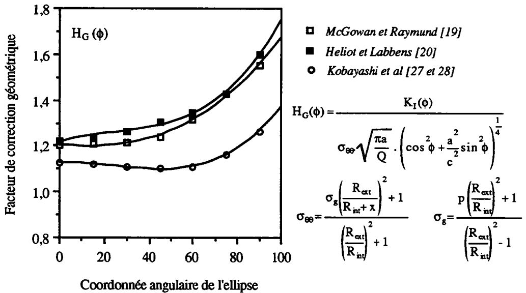
Figure I.8b. Courbes des facteurs de correction géométrique données par différents auteurs, pour les rapports a/B = 0,5 , a/c = 1/3 et B/R_{int} = 0,1 [19].
