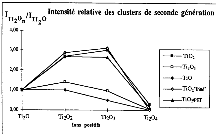
Figure 3.14 : Analyse LAMMA en mode positif - Empreintes spectrales d'une poudre de TiO 2 "frittée" et d'un film (échantillon 3) - Intensités relatives des ions rapportées à l'intensité de l'ion Ti 2 O +
