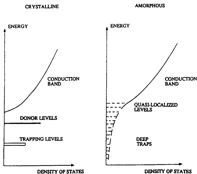
Figure 3.18 : Comparaison schématique des structures de bandes de diélectriques cristallins et amorphes d'après [163]
