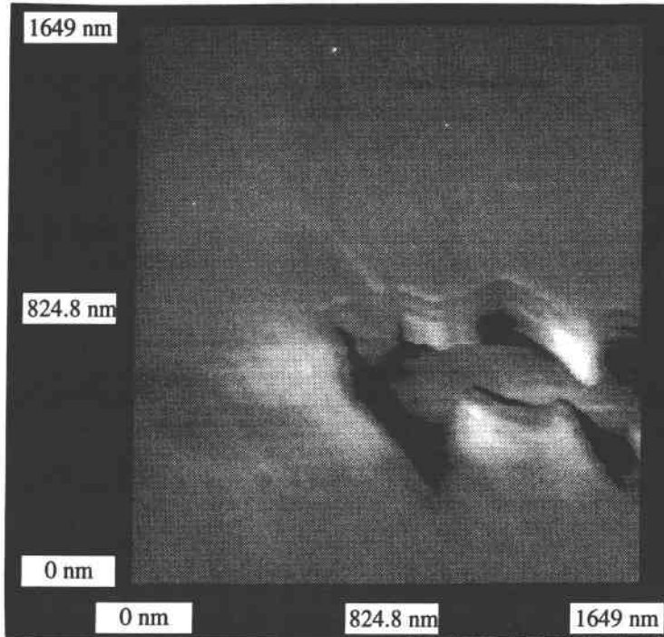
Cliché 3.10 : Cliché AFM d'un film TiO 2 /PET (expérience 12) - Surface 1649×1649 nm
