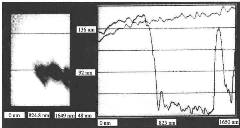
Cliché 3.11 : Profil AFM d'un film TiO 2 /PET (expérience 12) dans une zone présentant un trou - épaisseur du film : 1300Å
