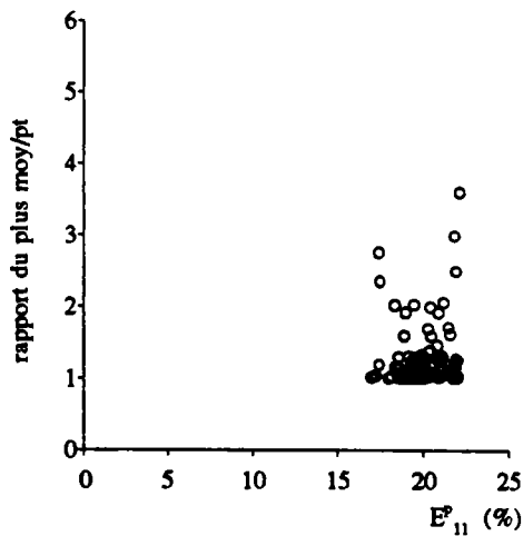
Fig.V.9.c : rapport du moyen sur le plus petit demi-axe pour une déformation plastique macroscopique de 20%
