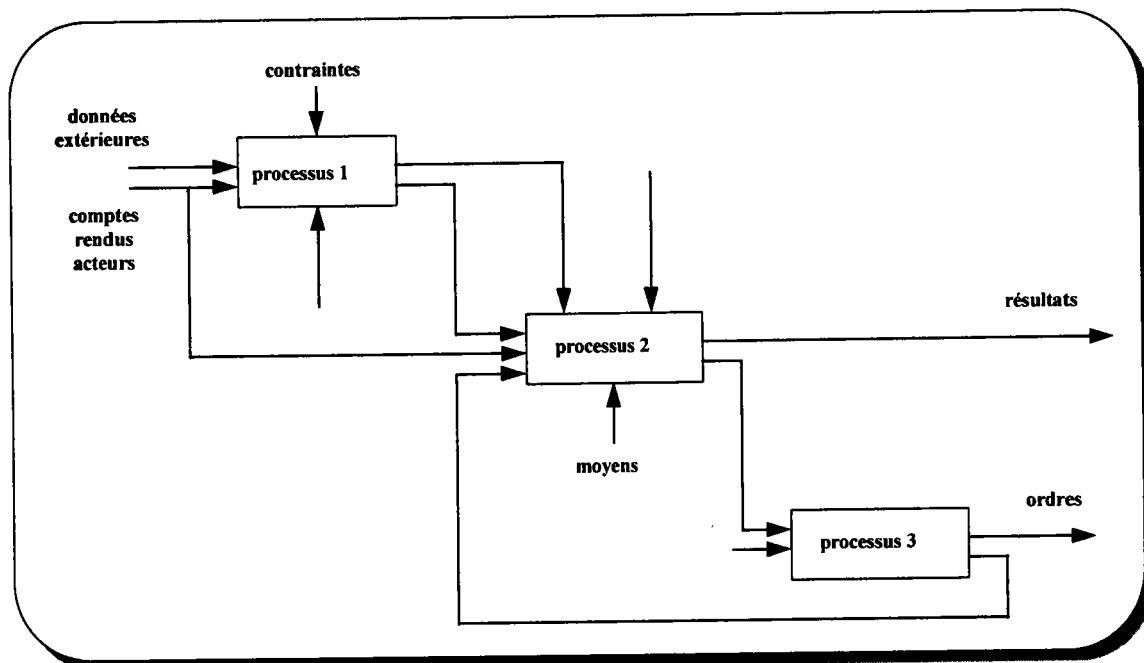
Fig.12 Modélisation du processus de production par SADT
