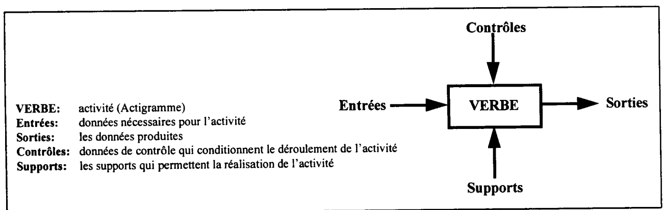
Fig. 18 Modèle SADT
