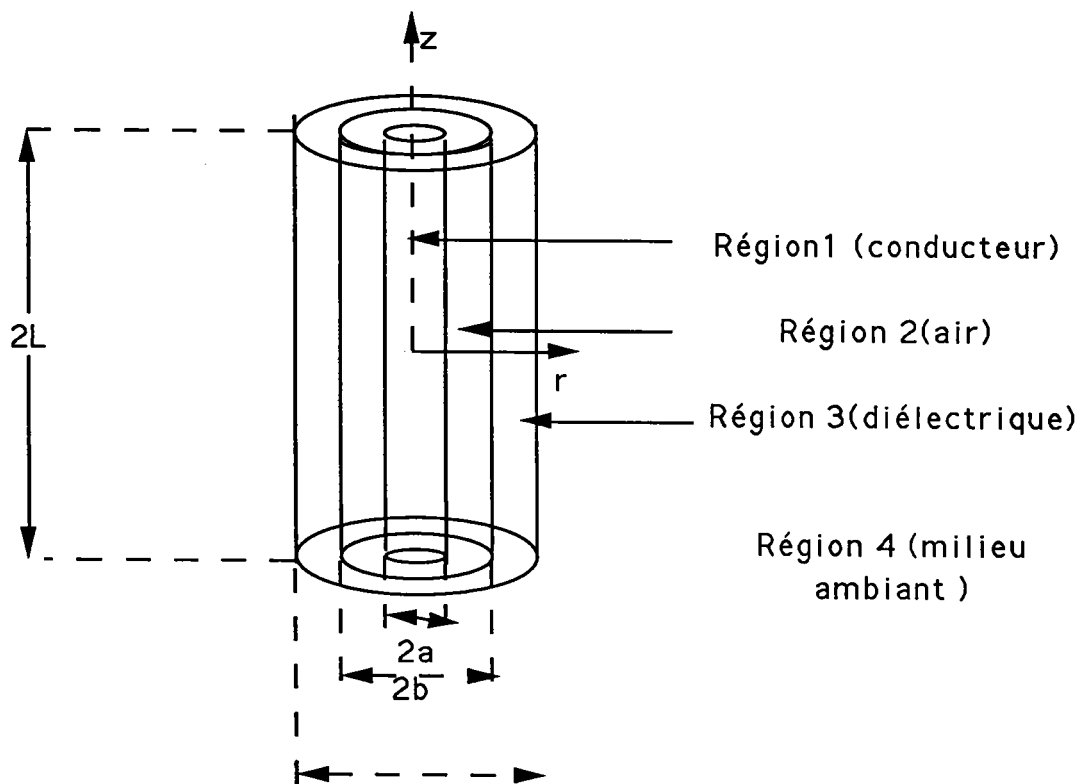
Figure 2.5. Antenne à gaine uniforme
