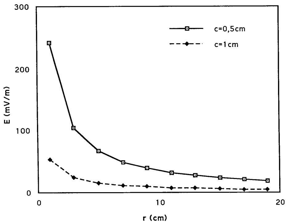
Figure 3.17. E = f(r) dans l'air, L=26\text{cm} , antennes à gaine uniforme
