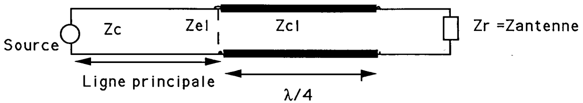
Figure 3.5. Adaptation par ligne \lambda/4
