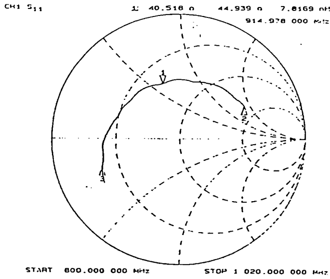
Figure 3.1. Impédance de l'antenne à gorge dans l'air
