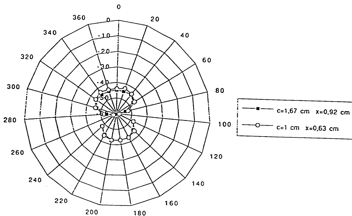
Diagramme de rayonnement - Polarisation horizontale
