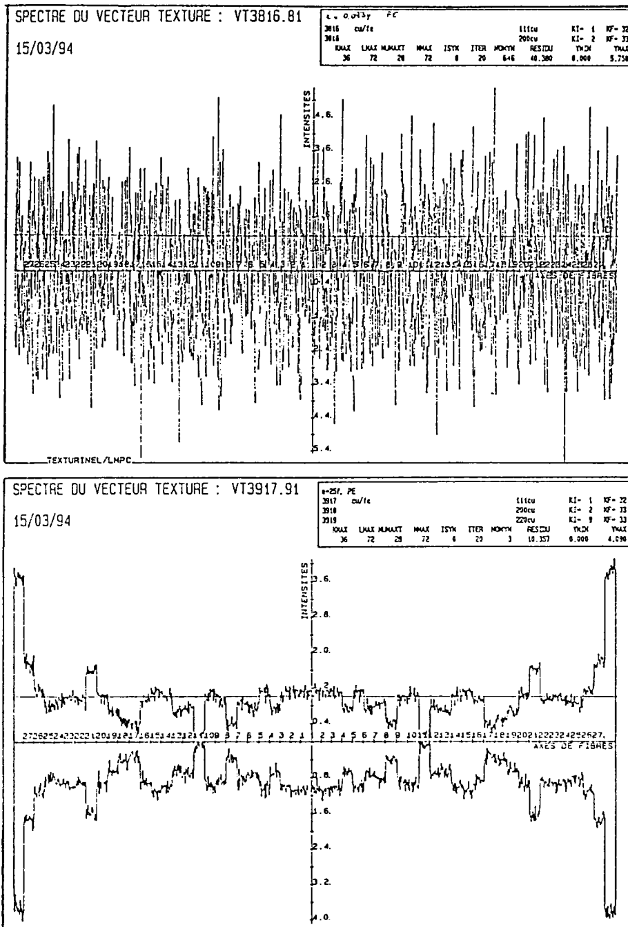
Figure II. 34: vecteur texture des échantillons à: (a) 0.083µm, (b) 25µm d'épaisseur.
