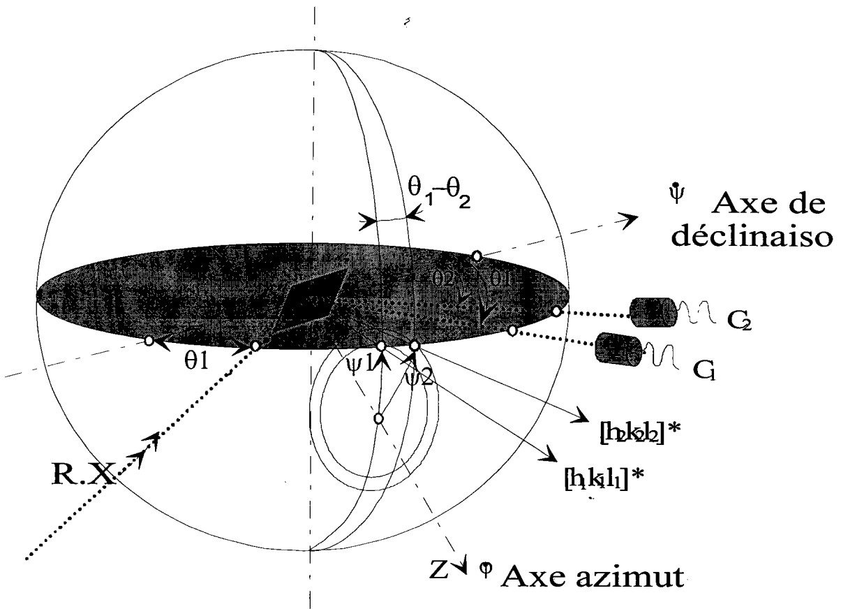
Figure I. 11: Géométrie de diffraction permettant l'obtention des figures de pôles.
