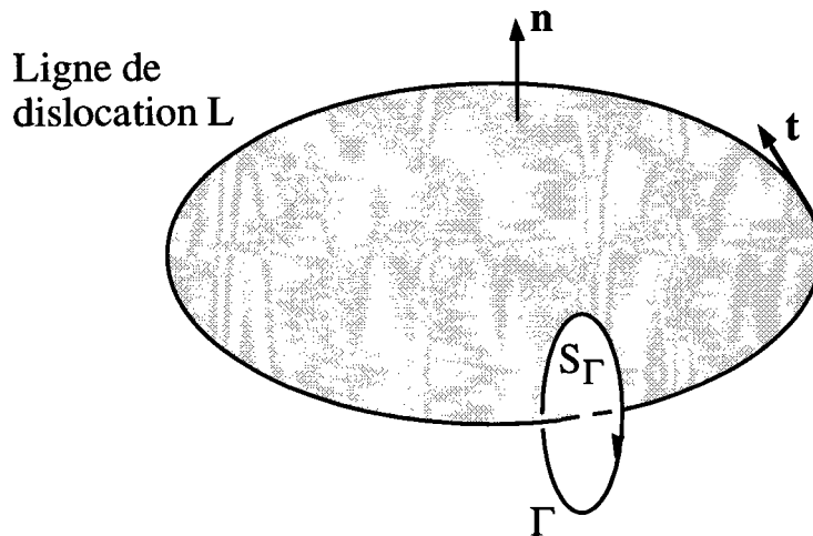
Figure II-4: Circuit et surface de Burgers d'une dislocation.
