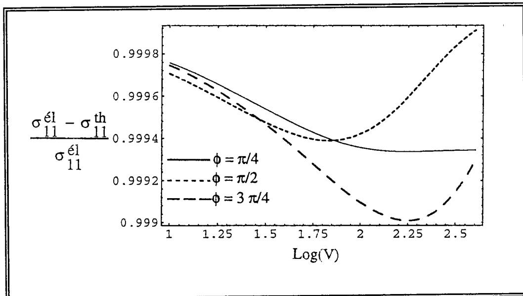
Figure B-2: Comparaison entre \sigma_{11}^{th} et \sigma_{11}^{él} pour r = 2 \mu\text{m} .
