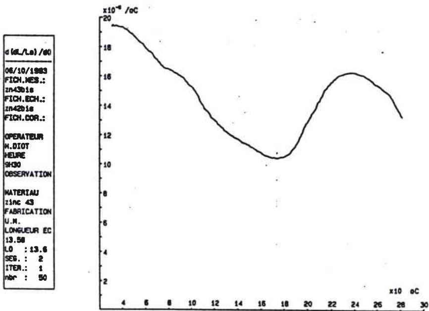
Courbe d(dL/L_0)/dT=f(T) : alliage 31043
