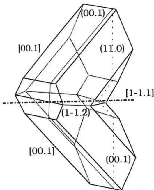
Le maclage (11.0)[1-1.1] du zinc
