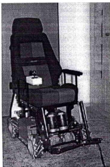
Figure II.11 : le projet OMNI et le système “Mecanum-Wheels”
