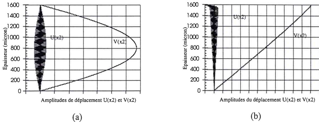
Figure A 35 : Amplitudes modales dans le cas d'un unidirectionnel. Chargement de compression, épaisseur du pli 1600 \mu\text{m} . Conditions aux limites : face inférieure bloquée, face supérieure (a) bloquée (b) libre.
