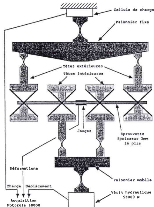
Figure A 12 : Montage de flexion 4 points (VITTECOQ 1991, ALLIX et al. 1988).
