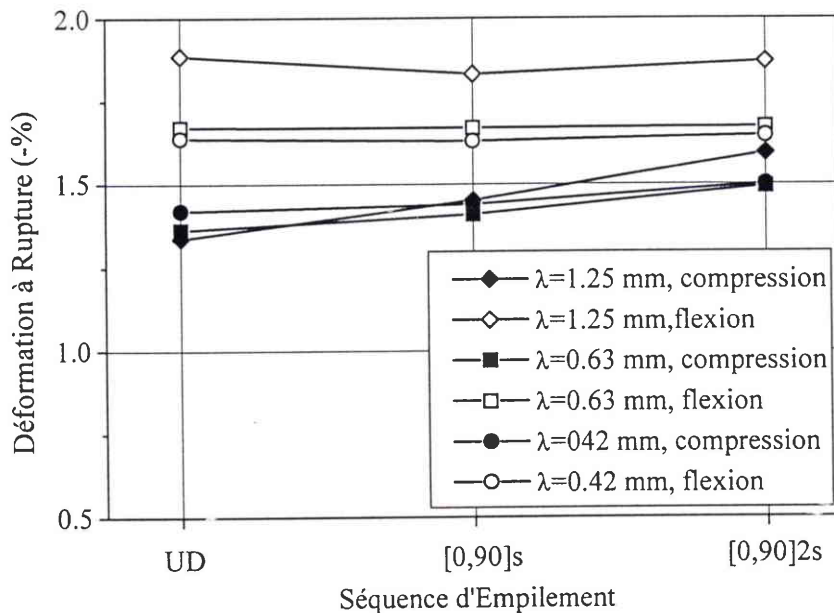
Figure D 64 : Influence de la longueur d'onde du défaut sur la résistance de stratifiés sous diverses sollicitations et pour différentes séquences d'empilement.
