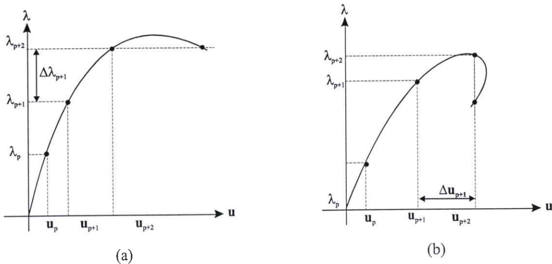
Figure C 3 : Pilotage (a) en chargement et (b) en déplacement.
