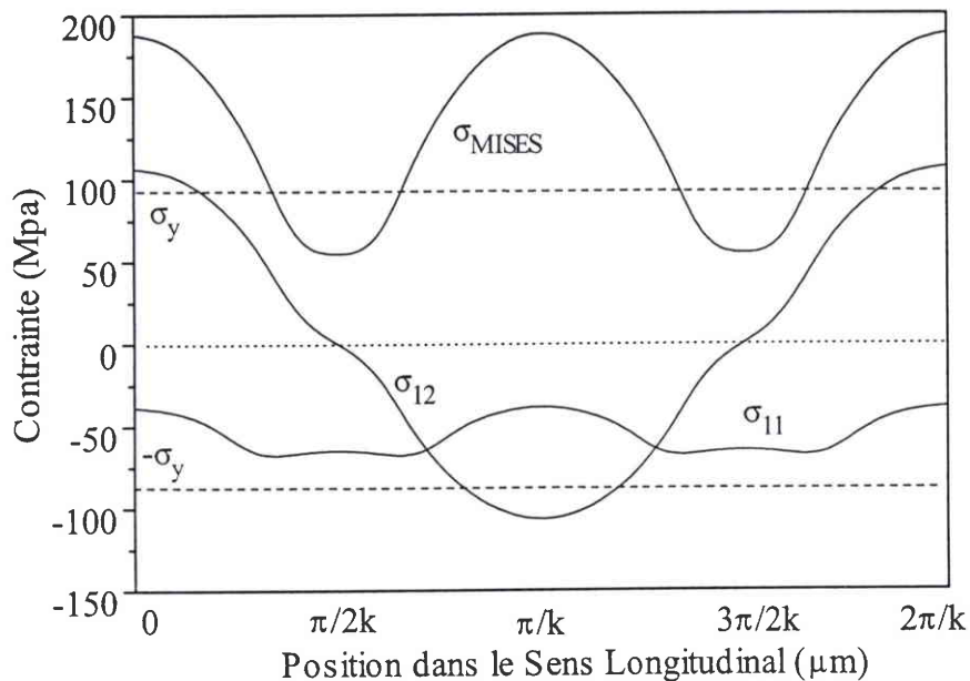
Figure D 11 : Profil des contraintes matrice dans la largeur du pli pour un chargement correspondant point de charge maximum (-1.40 %). Contraintes longitudinale, de cisaillement et de VON-MISES. Le défaut initial v_{01} est de 5 \mu\text{m} .
