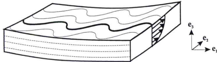
Figure A 29 : Gradient de déplacement v dans la hauteur du pli en flexion.
