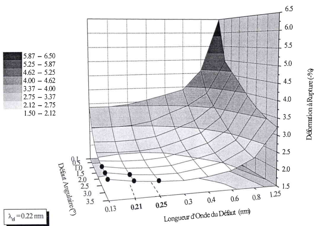
Figure D 39 : Évolution des déformations à rupture du pli, en fonction du défaut angulaire initial obtenu avec différentes longueurs d'onde. Pli de 1.6 mm en flexion-compression, bloqué-bloqué.
