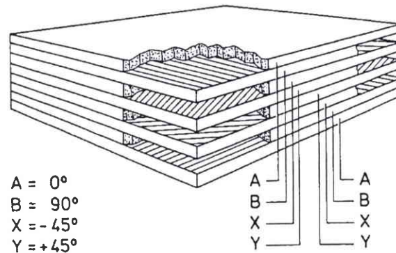
Figure A 5 : Stratifié symétrique [0,90,-45,+45]_s
