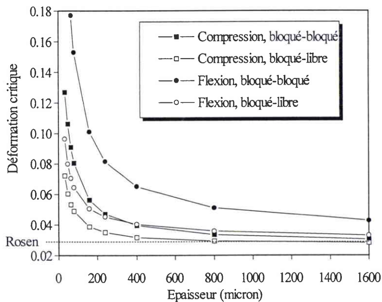
Figure A 36 : Déformations critiques en fonction de l'épaisseur du pli, du chargement et des conditions aux limites imposées sur ses faces inférieure et supérieure.
