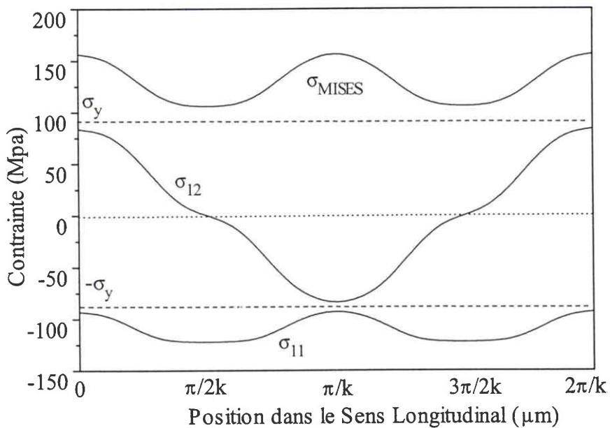
Figure D 9 : Profil des contraintes matrice dans la largeur du pli pour un chargement correspondant à l'apparition de l'instabilité (-2.37%). Contraintes longitudinale, de cisaillement et de VON-MISES. Le défaut initial v_{01} est de 1 \mu\text{m} .
