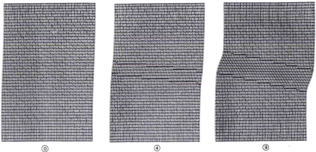
Figure A 27 : Maillages bidimensionnels d'une \frac{1}{2} longueur d'onde du pli UD. Étapes 0, 4 et 9 de la courbe obtenue par la modélisation ci-dessus. Les points noircis figurent les endroits où le moment de flexion dans les fibres est maximum (KYRIAKIDES et al., 1995).
