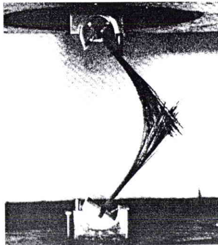
Figure A 13 : Rupture de la face en tension d'un UD XAS/913 sur un montage de flambage rotulé (WISNOM, 1992).
