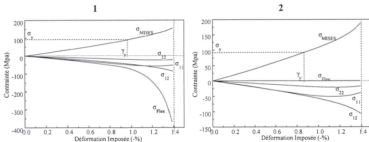
Figure D 10 : Évolution des contraintes aux pseudo-noeuds 1 et 2, le défaut initial v_{01} est de 5 \mu\text{m} .
