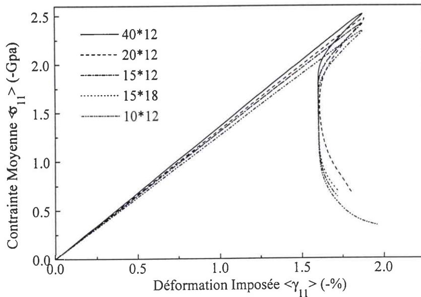
Figure D 2 : Réponses calculées pour différents maillages (nombre d'éléments selon e_2 * nombre de divisions sur e_1 ) d'un pli UD T300/914 de 3200 \mu\text{m} bloqué-libre en compression.
