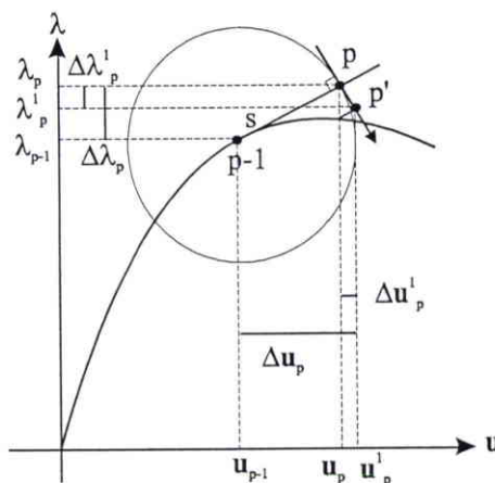
Figure C 4 : Convergence de la prédiction et de la correction pour la méthode de RAMM.
