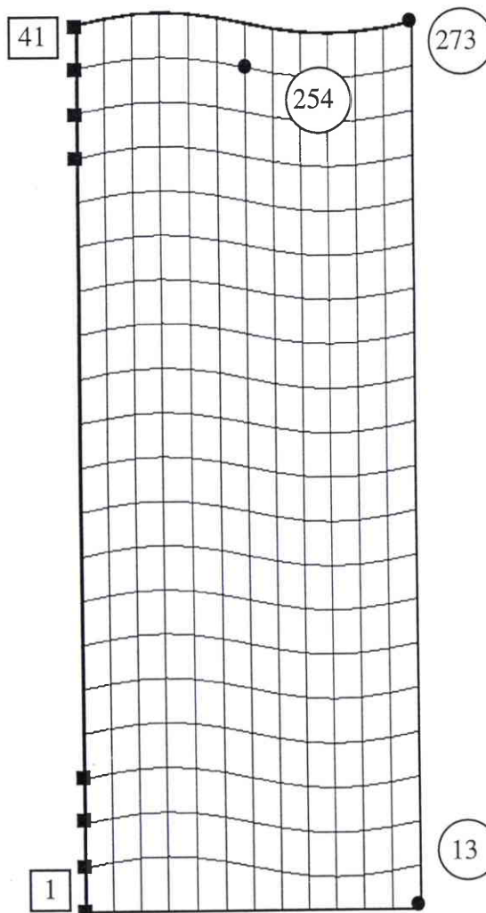
Figure D 3 : Maillage de 20 éléments et 12 divisions. Le défaut v_{01} de 1 \mu\text{m} constant dans l'épaisseur est amplifié par 10 pour être visible sur ce pli de 1600 \mu\text{m} bloqué-libre.
