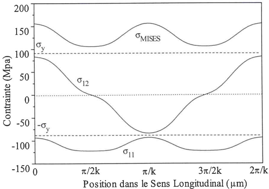
Figure D 9 : Profil des contraintes matrice dans la largeur du pli pour un chargement correspondant à l'apparition de l'instabilité (- 2.37 %). Contraintes longitudinale, de cisaillement et de VON-MISES. Le défaut initial v_{01} est de 1 \mu\text{m} .
