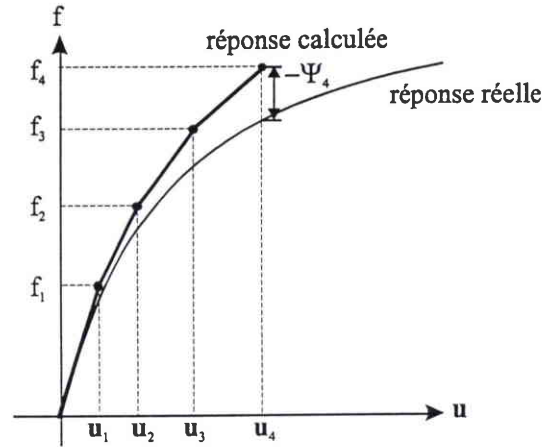
Figure C 1 : Résolution d'un problème non linéaire \Psi(\mathbf{u};\delta\mathbf{u}) = 0 par un schéma incrémental.
