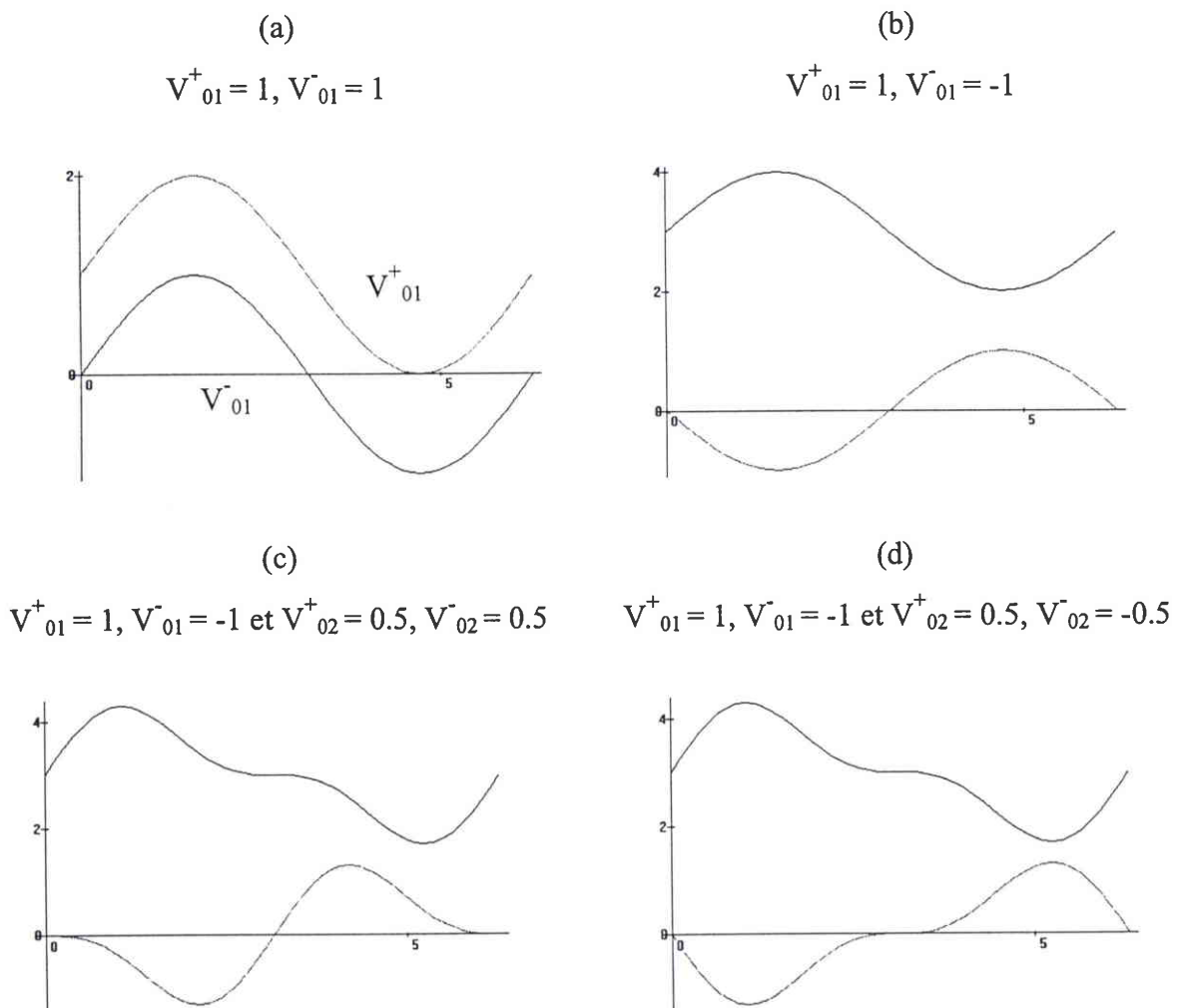
Figure D 15 : Formes du défaut initial, obtenues en combinant les amplitudes V_{01} et V_{02} (en \mu\text{m} ).
