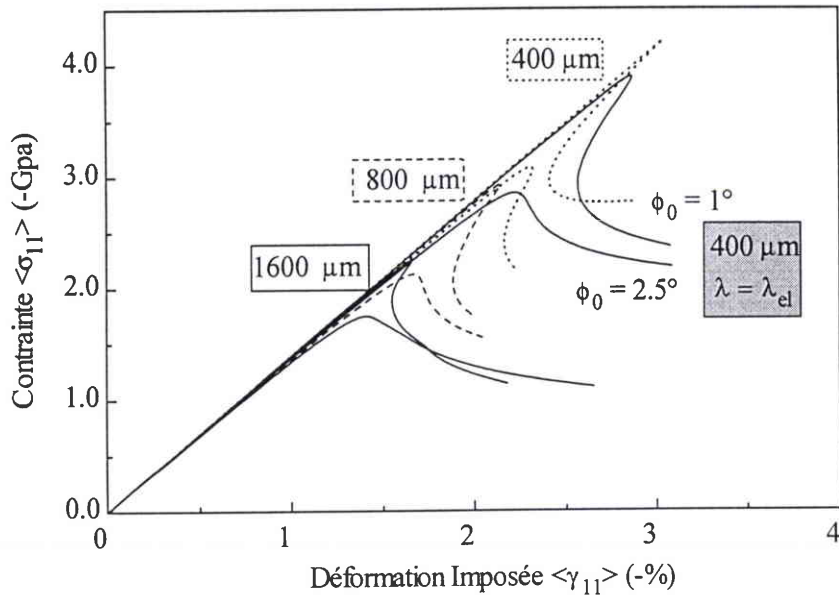
Figure D 46 : Réponse d'un pli UD en compression, bloqué-bloqué, pour différentes épaisseurs et 2 défauts angulaires de longueur d'onde 0.63 mm (si non indiquée).
