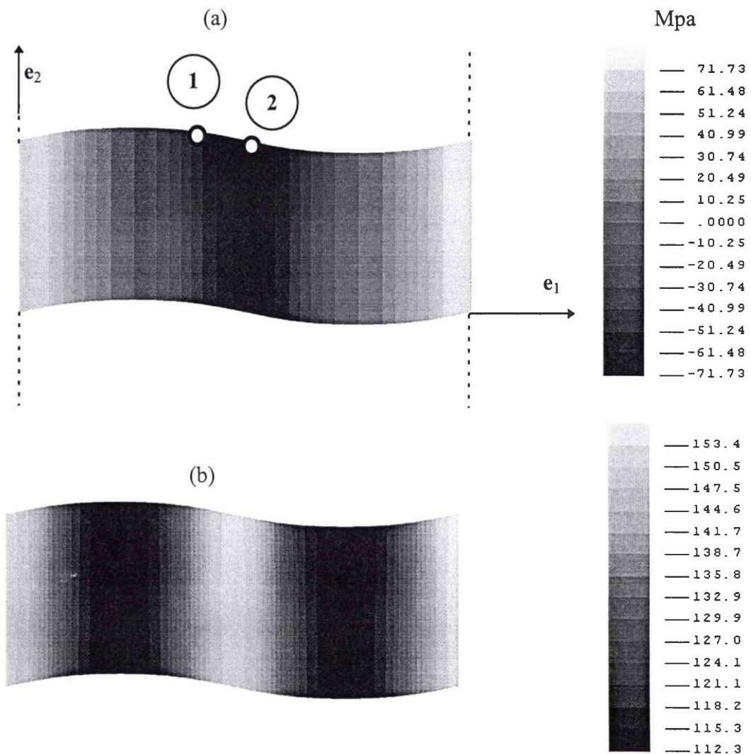
Figure D 7: Distribution des contraintes dans la matrice à mi-hauteur du pli affecté d'un défaut v_{01} = 1 \mu\text{m} , pour un chargement correspondant à la charge maximum (-1.89 % soit -2463 Mpa) :
