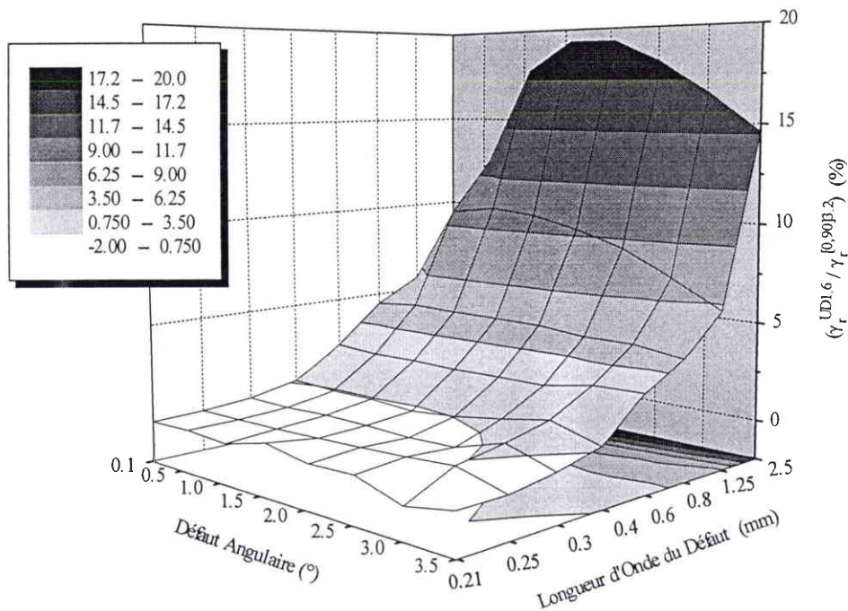
Figure D 56 : Évolution de la différence relative entre les déformations à rupture correspondant à un pli UD de 1.6 mm bloqué-bloqué et un stratifié [0,90] bloqué-libre de 3.2 mm, en fonction du défaut initial obtenu avec différentes longueurs d'onde.
