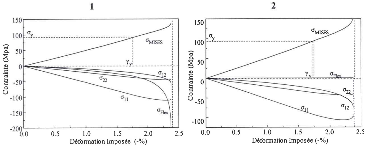
Figure D 8 : Évolution des contraintes aux pseudo-noeuds 1 et 2 jusqu'à l'instabilité : contraintes longitudinales ( \sigma_{11} ), de cisaillement ( \sigma_{12} ), transverse ( \sigma_{22} ), de MISES ( \sigma_{Mises} ) dans la matrice et de flexion ( \sigma_{Flex} ) dans la fibre. Le défaut initial v_{01} est de 1 \mu\text{m} .
