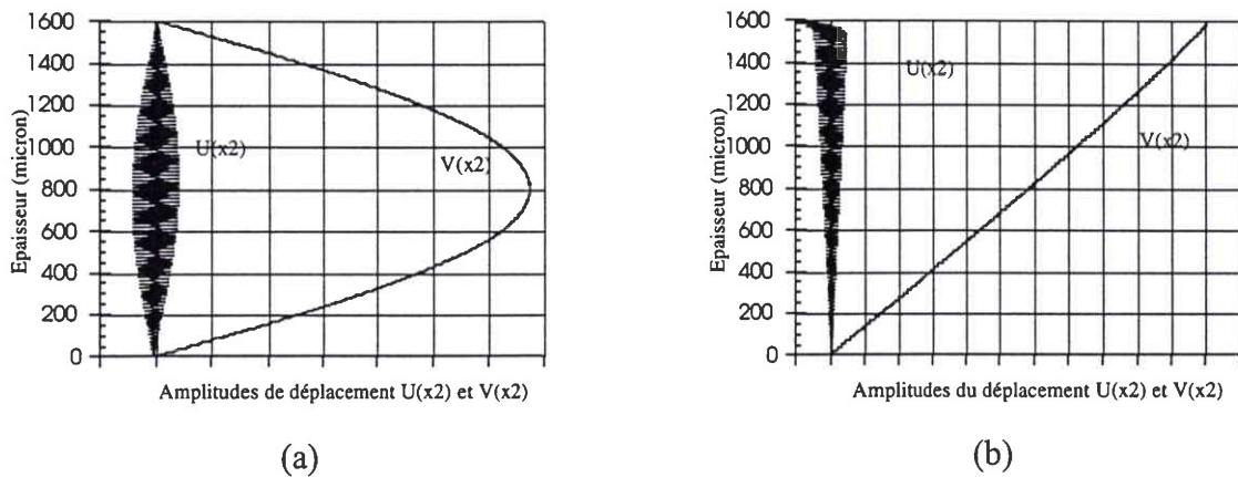
Figure A 35 : Amplitudes modales dans le cas d'un unidirectionnel. Chargement de compression, épaisseur du pli 1600µm. Conditions aux limites : face inférieure bloquée, face supérieure (a) bloquée (b) libre.
