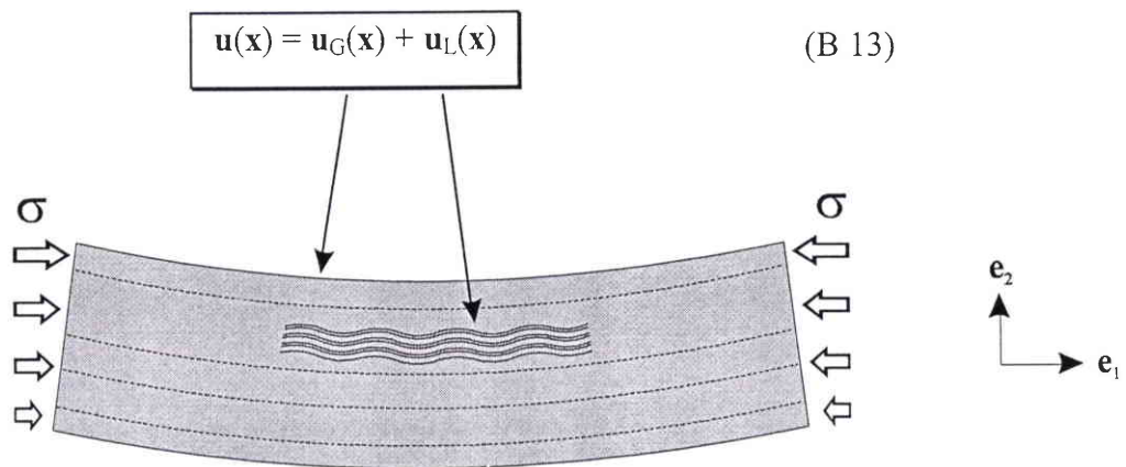
Figure B 3: Schématisation du microflambage dans un UD en flexion, et champ de déplacement associé.
