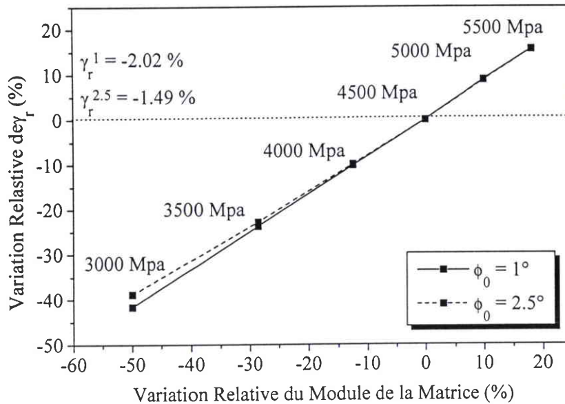
Figure D 29 : Influence de la variation du module de la matrice sur la déformation à rupture du pli.
