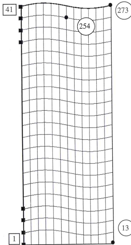
Figure D 3 : Maillage de 20 éléments et 12 divisions. Le défaut v_{01} de 1 \mu\text{m} constant dans l'épaisseur est amplifié par 10 pour être visible sur ce pli de 1600 \mu\text{m} bloqué-libre.
