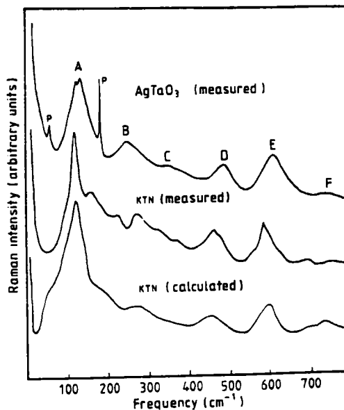
Figure II.11: Spectres Raman expérimentaux et calculés pour KTN ( x=0.008 ) (300 K), AgTaO_3 (775 K) dans la phase cubique. (Hafid, 1985)
