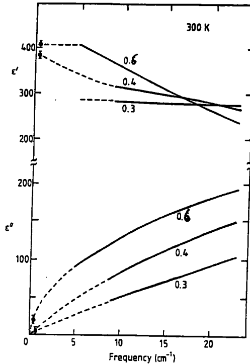
Spectre submillimétrique de ATN pour x=0.3 , 0.4 et 0.6 , à température ambiante. Les lignes pointillées sont des extrapolations.
