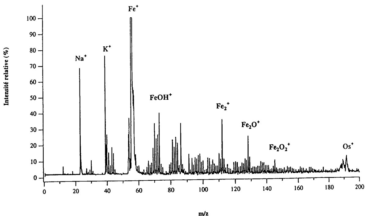
Figure IV-5. Spectre LAMMA en mode RELAI ( \lambda=293,7 \text{ nm} I = 10^7 \text{ W/cm}^2 ) d'une cellule L 132 incubée en présence de \text{Fe}_3\text{O}_4 .
