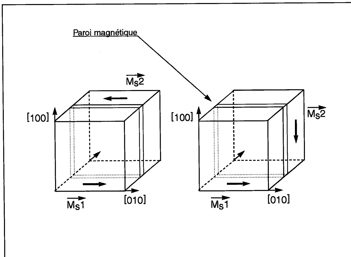
Fig. 2.2 : Domaines magnétiques d'aimantation antiparallèle (g) et orthogonale (d)
