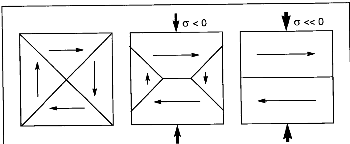
Fig. 4.9 : Effet de la contrainte de compression sur la distribution des domaines
