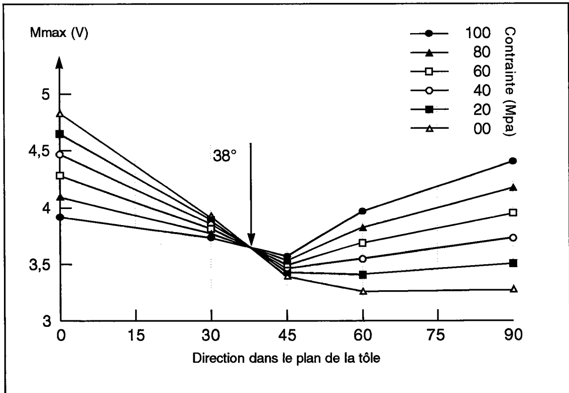
Fig. 6.12 : Tôle T5 / Variation de l'activité Barkhausen M_{max} en fonction de la direction de mesure pour différentes valeurs de la contraite transverse.
