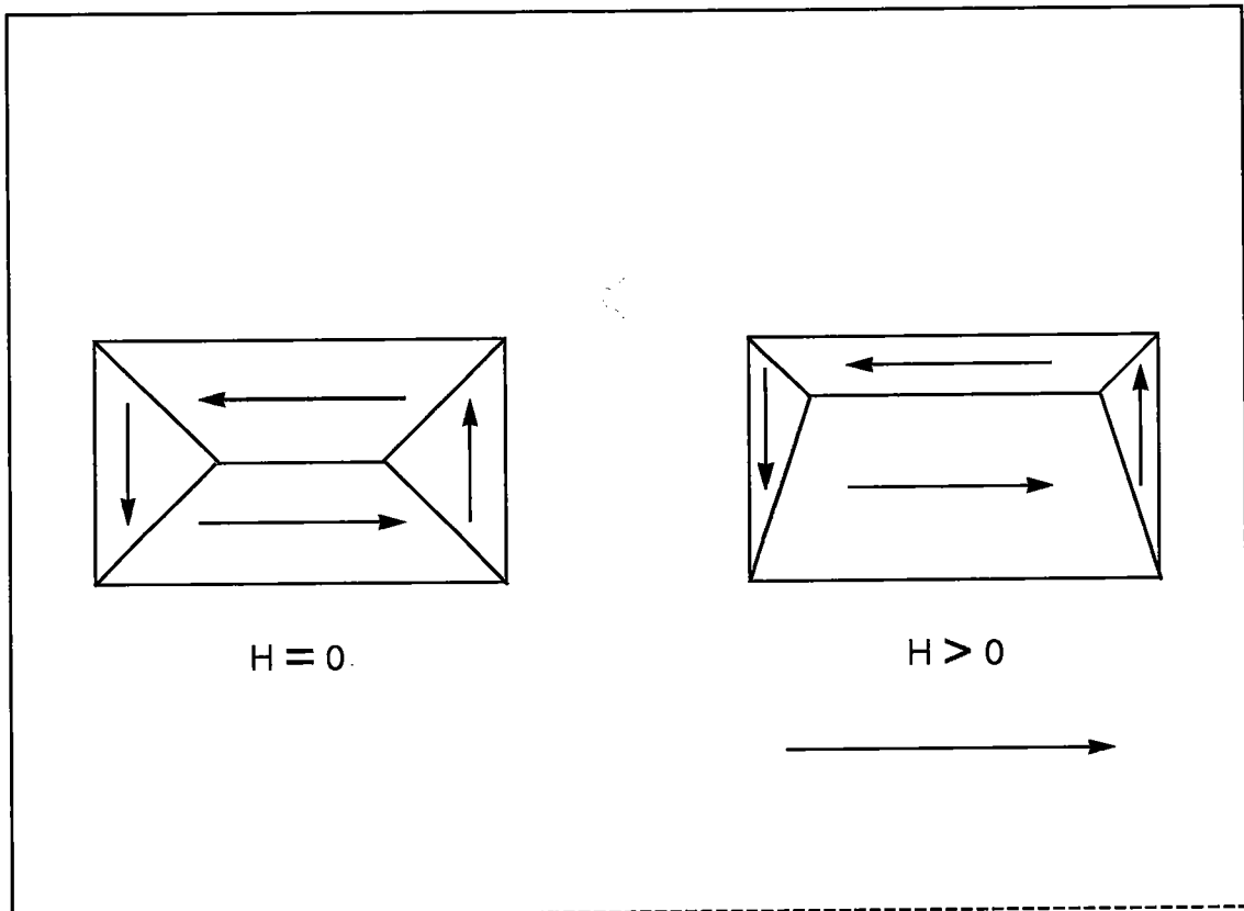
Fig. 2.8 : Redistribution des domaines sous l'effet du champ magnétique
