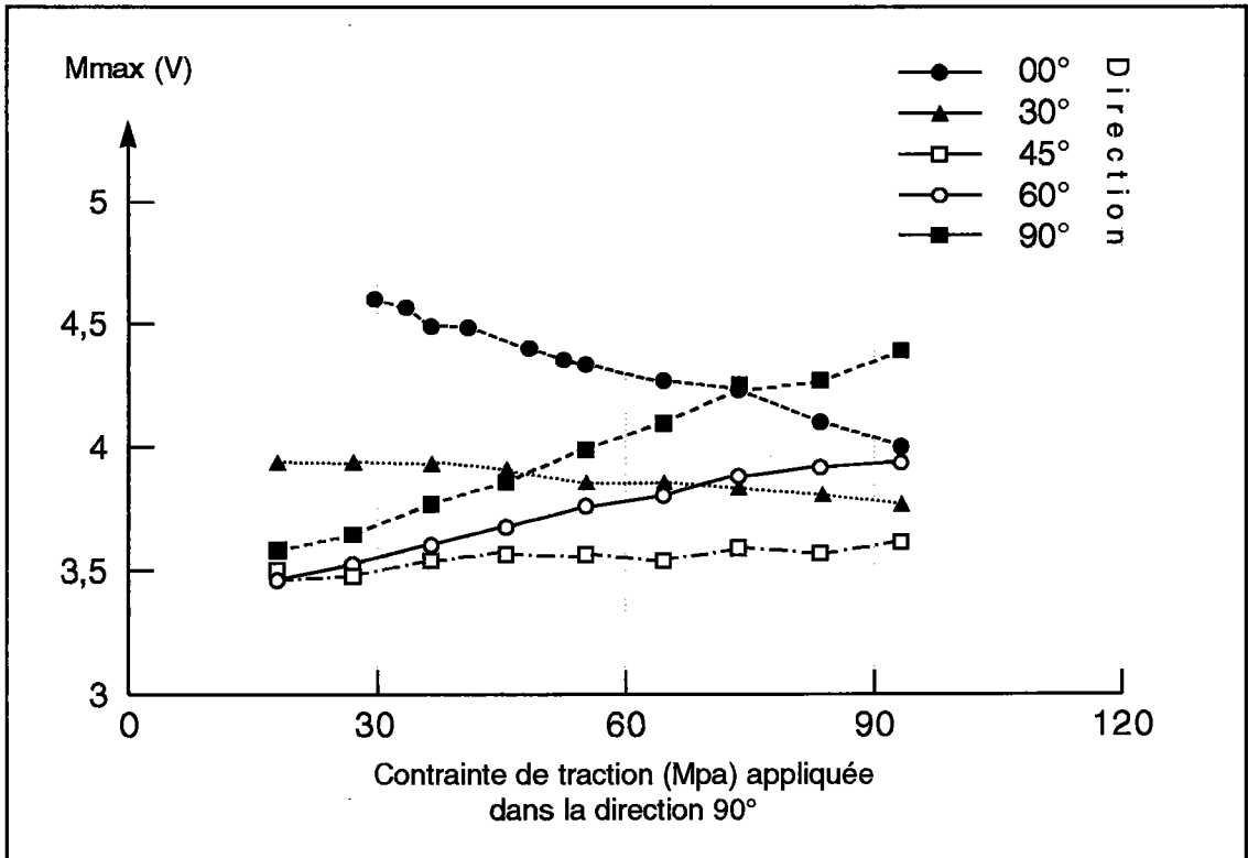
Fig. 6.11 : Tôle T5 / Variation de l'activité Barkhausen M_{max} en fonction de la contraite transverse pour les directions 00°, 30°, 45°, 60° et 90°.
