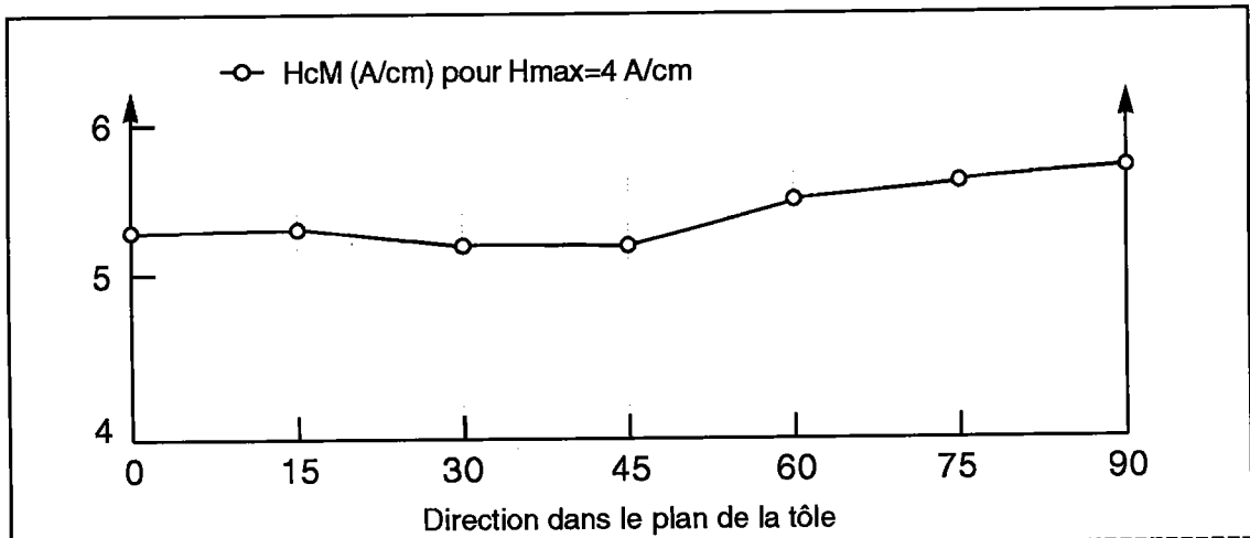
Fig. 6.23 : Tôle T6 / Champ coercitif H_{cM} en fonction de la direction de mesure pour une intensité de magnétisation de 4 A/cm.
