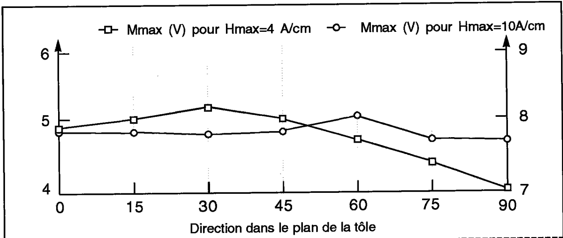
Fig. 6.22 : Tôle T6 / Activité Barkhausen M_{max} en fonction de la direction de mesure pour des intensités de magnétisation de 4 et 10 A/cm.
