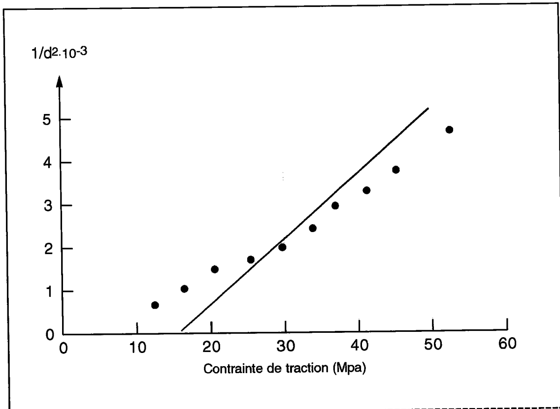
Fig. 5.11 : Variation de la largeur d des domaines longitudinaux en fonction de la conainte (relation théorique et mesures expérimentales) Réf.[5.4]
