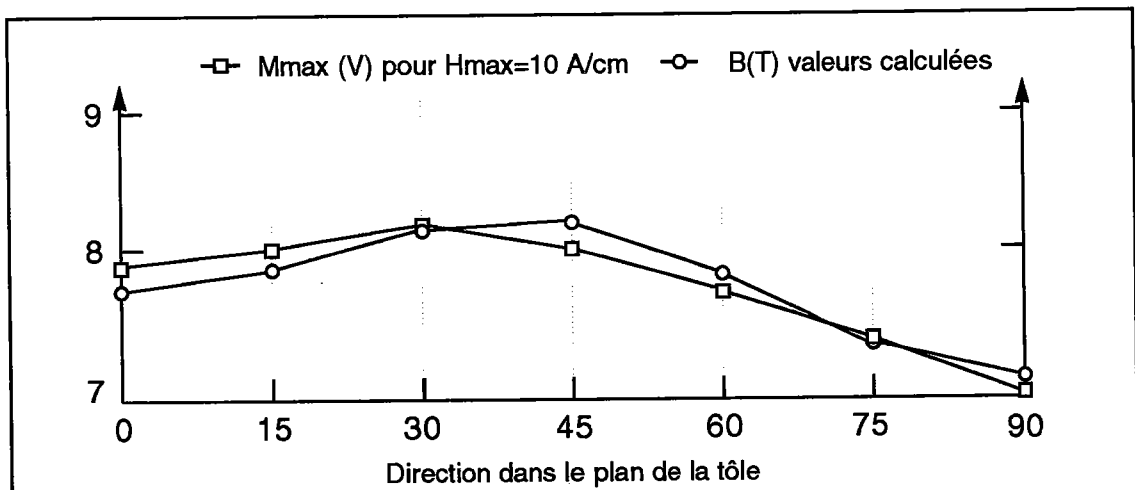
Fig. 6.24 : Tôle T6 / Activité Barkhausen M_{max} mesurée et induction B (T) calculée en fonction de la direction de mesure dans le plan de la tôle.
