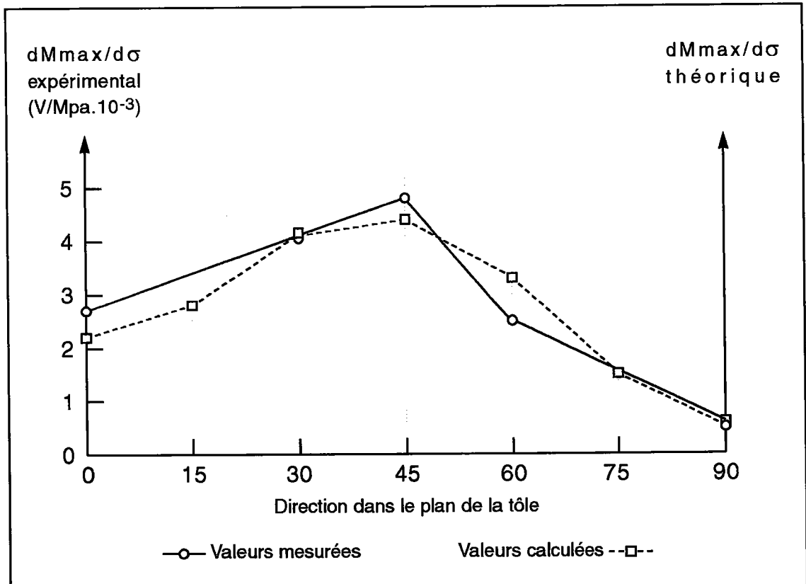
Fig. 6.4 : Tôle T2 / Susceptibilités magnétoélastiques mesurée et calculée de l'activité Barkhausen en fonction de la direction de mesure.
