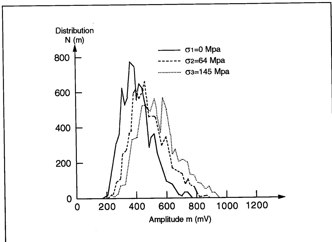
Fig. 5.7 : Distribution de l'amplitude des sauts Barkhausen m pour trois états de contrainte Réf.[5.9]
