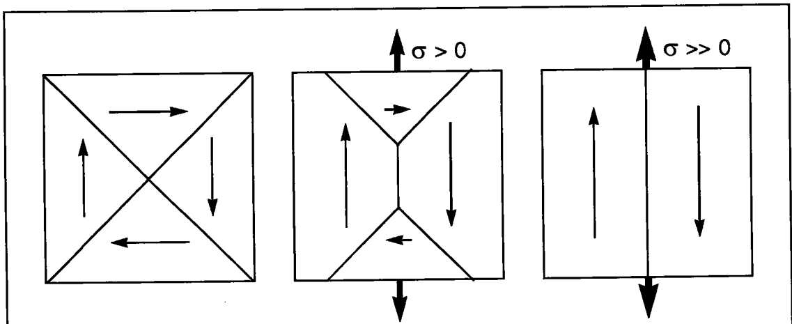
Fig. 4.8 : Effet de la contrainte de traction sur la distribution des domaines
