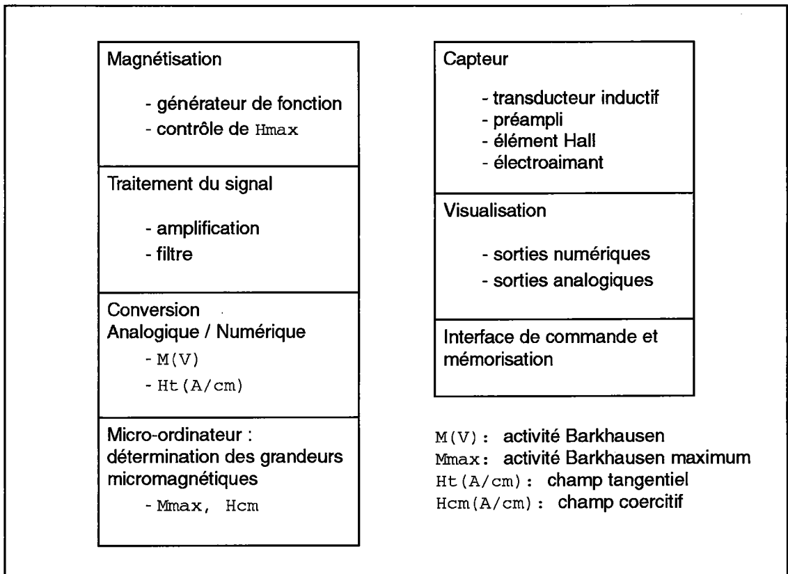
Fig. 3.1 : Principe de fonctionnement de l'appareil 3MA
