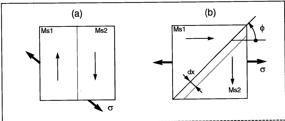
Fig. 4.7 : Domaines M_{s1} , M_{s2} aimantés orthogonalement et contrainte uniaxiale appliquée \sigma
