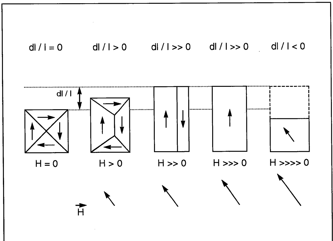
Fig. 2.11 : Magnétostriction en fonction des mécanismes de magnétisation
