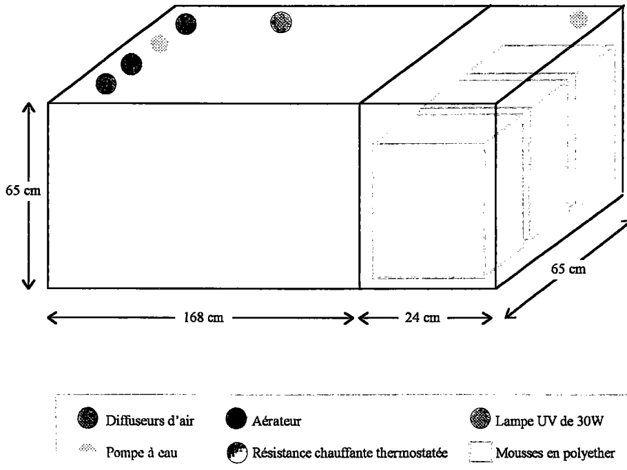
Figure 2. Dispositif d'élevage II : aquarium de 600 litres.
