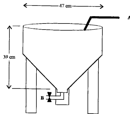
A : arrivée d'air B : vanne de vidange
