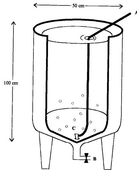
A : arrivée d'air B : vanne de vidange C : diffuseur d'oxygène
