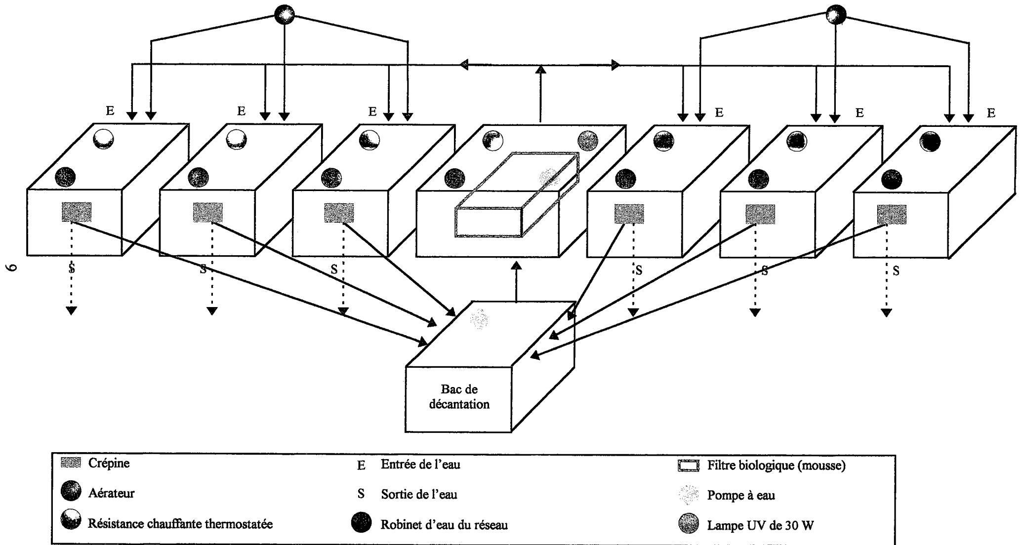
Figure 1 : Dispositif d'élevage I : bacs à fond rectangulaire de 40 litres.
