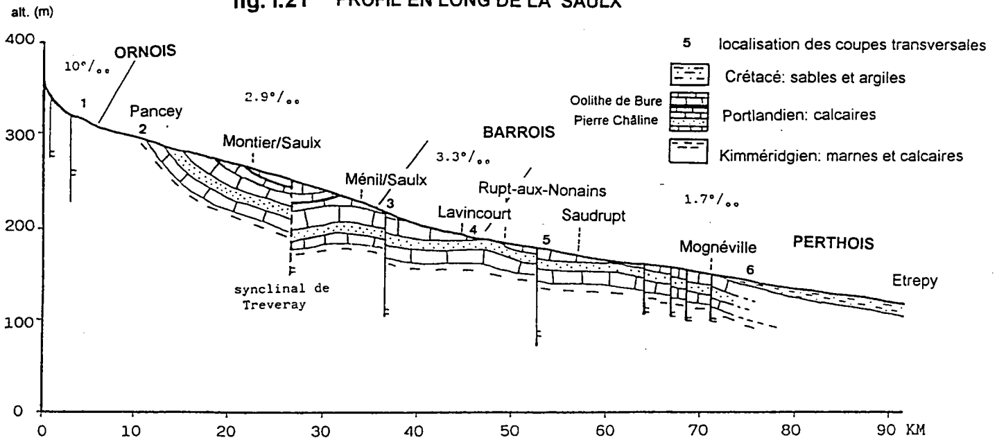
fig. I.21 PROFIL EN LONG DE LA SAULX
