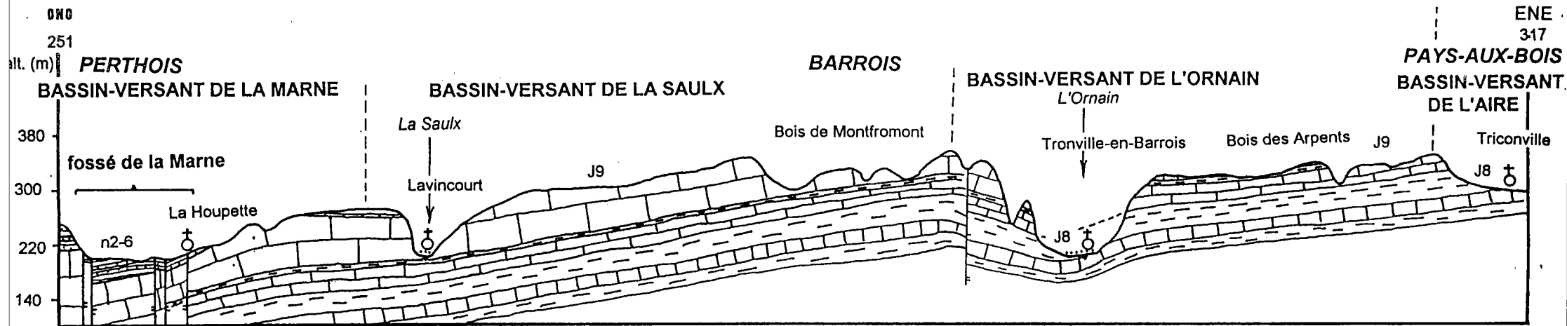
fig. I.12 COUPE GEOLOGIQUE DANS LE BARROIS
