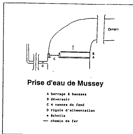
Section rectiligne avec prise statique
