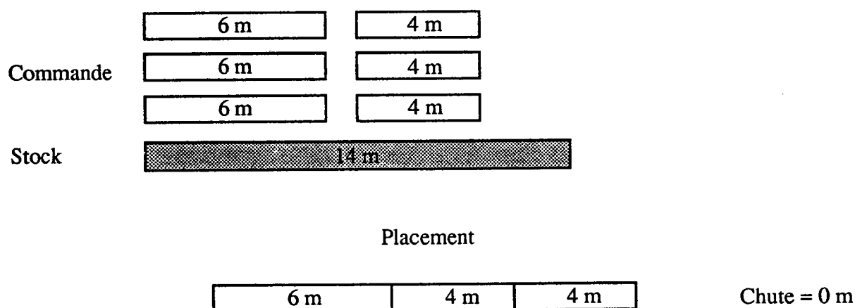
Figure IV.4 : Résultat du placement par l'algorithme de l'arborescence limitée
