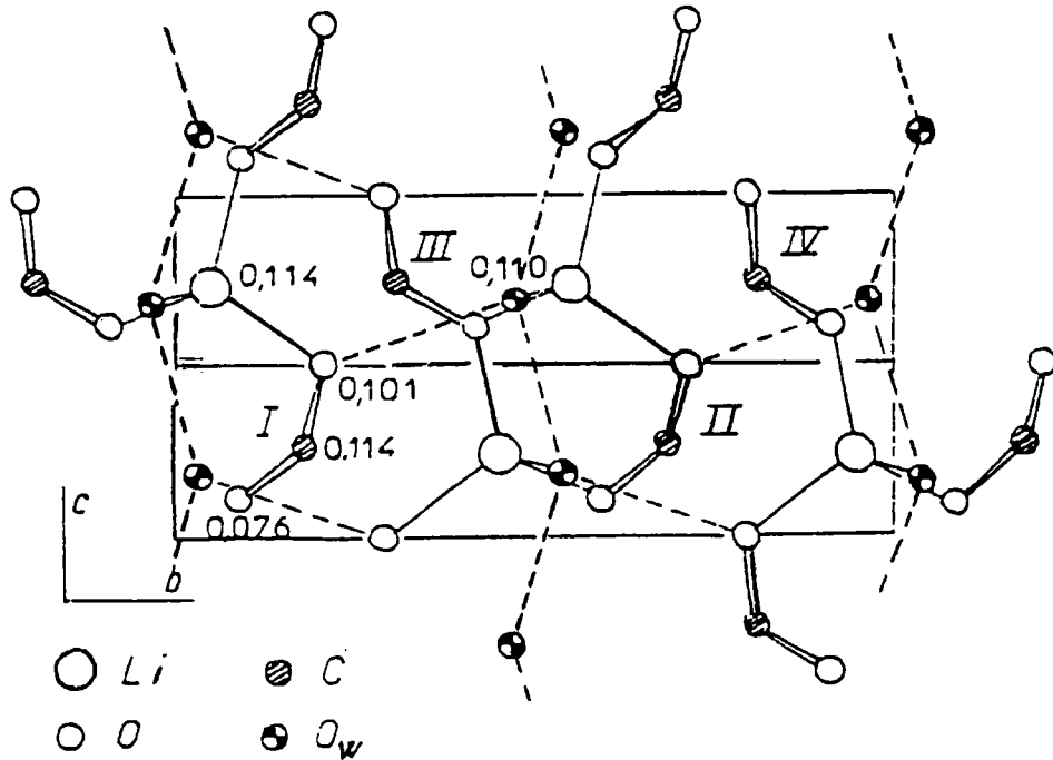
Figure I.4: Structure cristallographique du LiHCOO.H 2 O vue le long de l'axe a.
