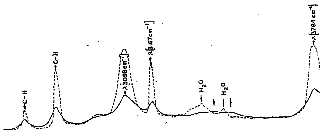
Figure I.10: Spectre Raman polarisé dans la région 2200-3700 cm -1 [---, rétrodiffusion (b → b); —, diffusion à angle droit (b → c)].
