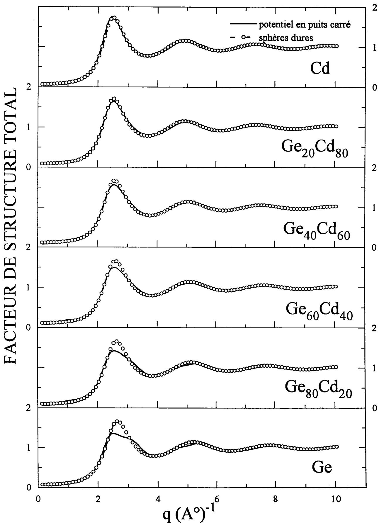
Figure (5-20) : facteur de structure total théorique de l'alliage liquide Cd-Ge à 950°C
