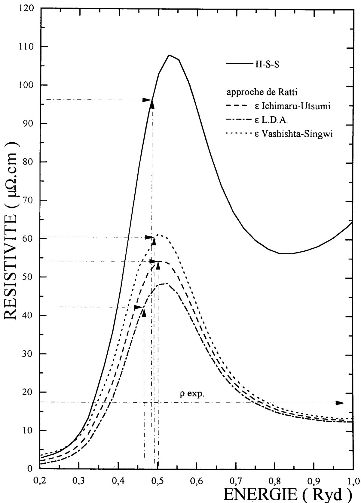
Figure (4-14) : résistivité de l'Argent à 1000^\circ\text{C} : cas de l'atome neutre (H.S.S) ; et du potentiel ionique écranté suivant la méthode de Ratti.
