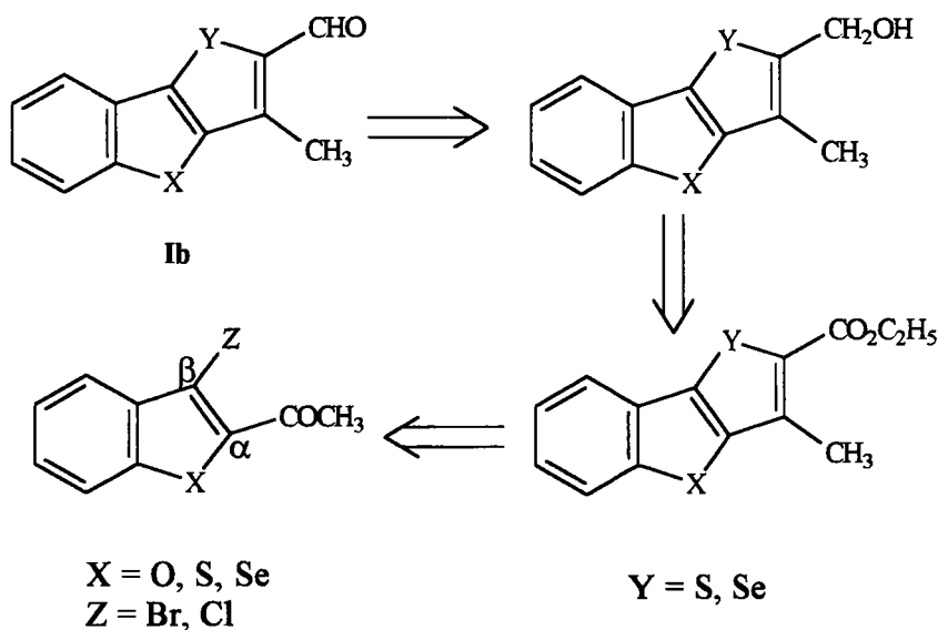
Schéma 110
