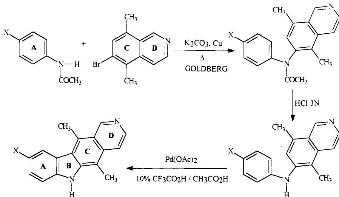
Schéma 86
