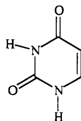
Uracile
