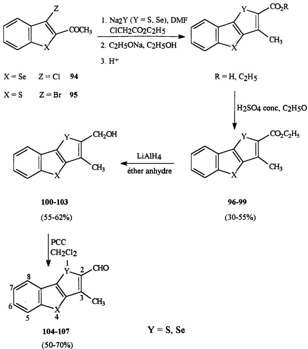
Schéma 112
