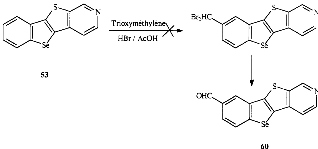
Schéma 77
