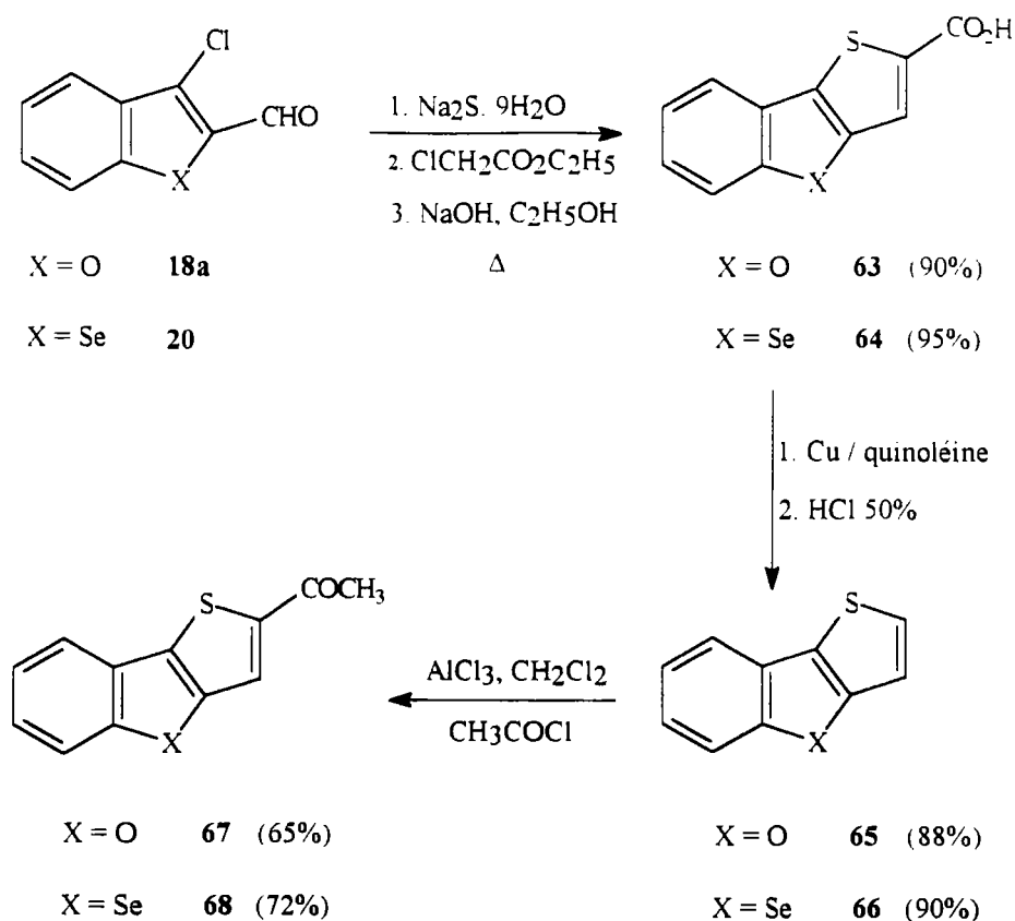
Schéma 82
