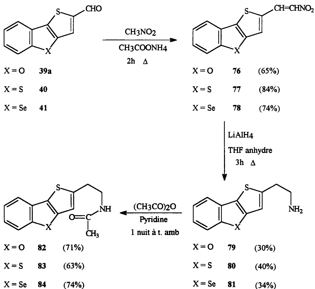
Schéma 99
