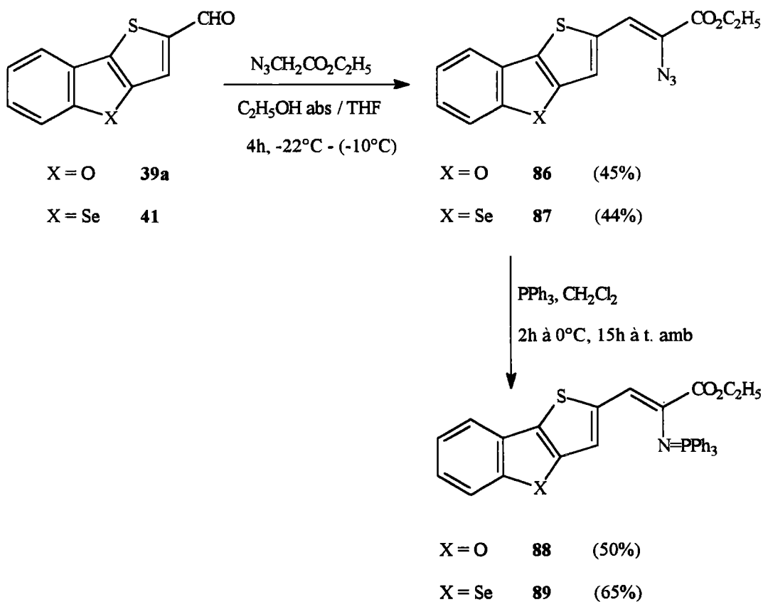
Schéma 105
