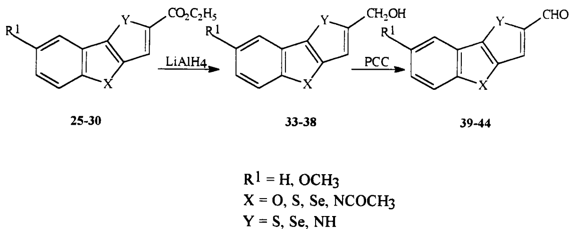
Schéma 54
