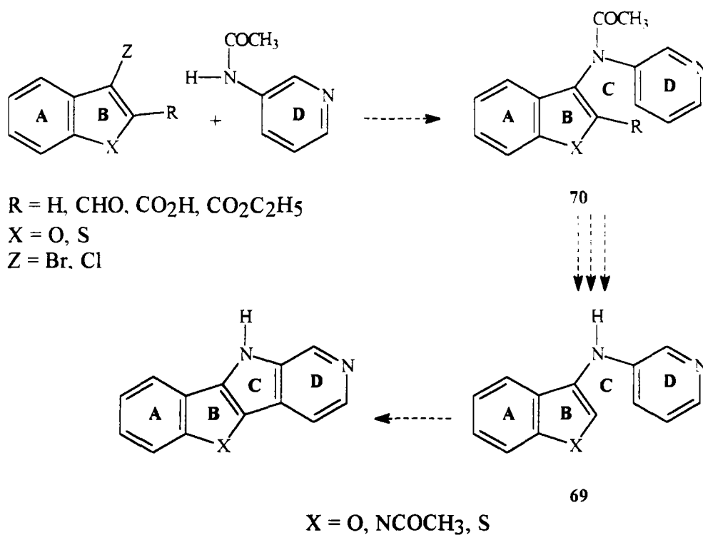
Schéma 87
