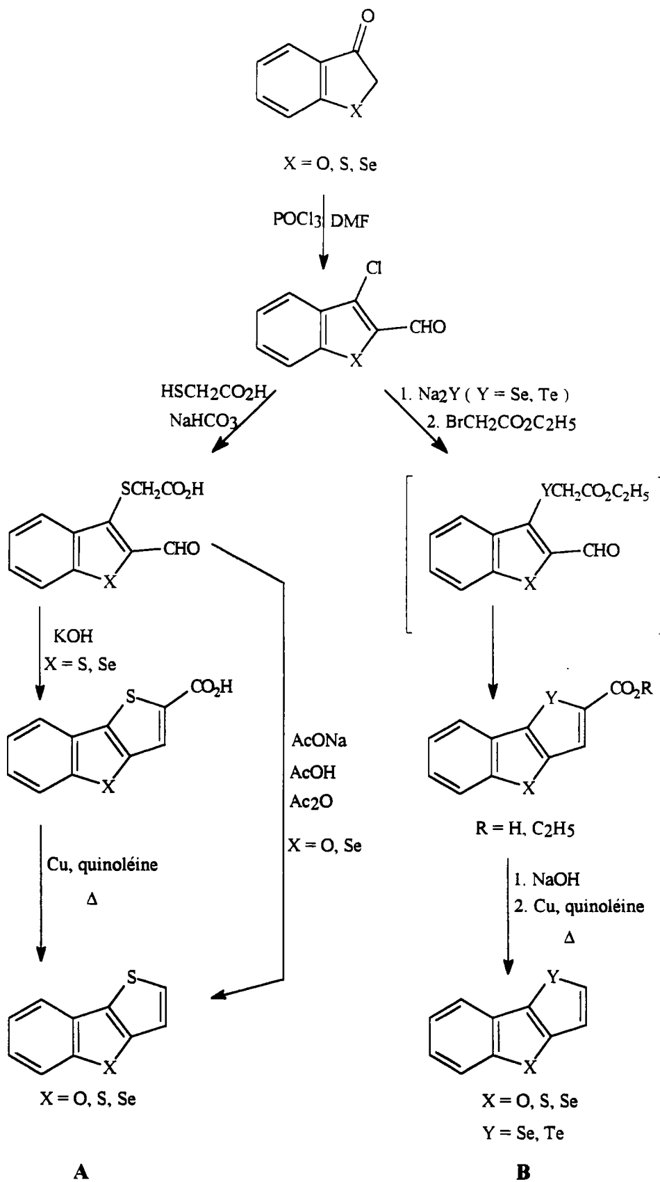
Schéma 48
