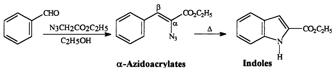
Schéma 107
