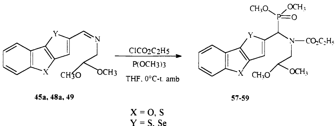
Schéma 70
