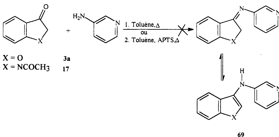
Schéma 85
