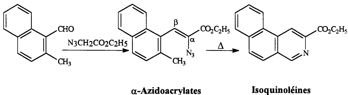
Schéma 108
