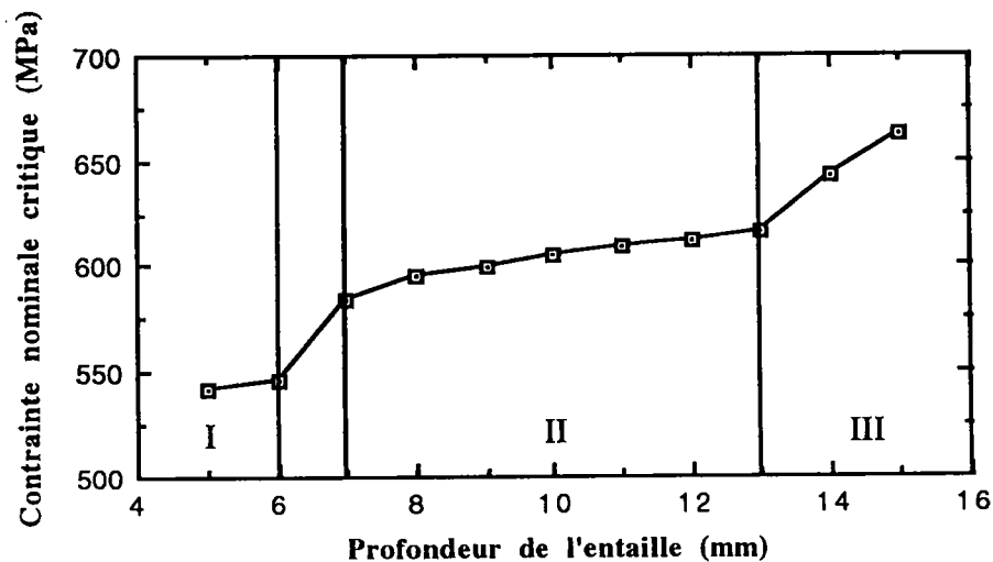
Figure 4.14 : Variation de \sigma_{\max}^c en fonction de a pour \rho = 0 mm
