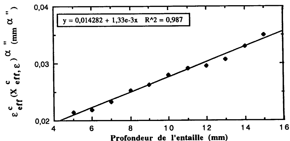
Figure 4.38 : Variation de \epsilon^c_{\text{eff}}(X^c_{\text{eff},\epsilon})^{\alpha''} en fonction de a .
