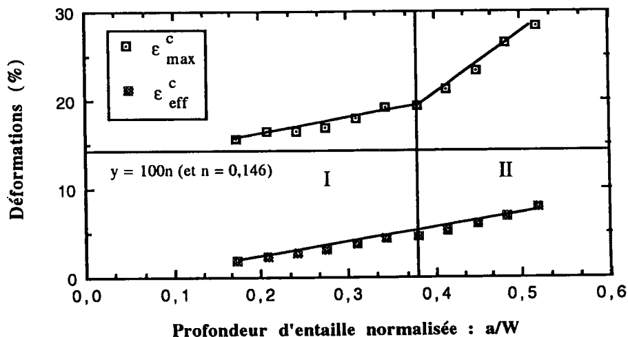
figure 4.21 : Variation de \epsilon^c_{max} et de \epsilon^c_{eff} avec la profondeur d'entaille a/W .
