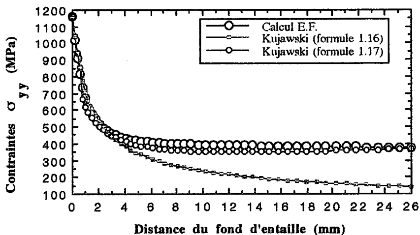
Figure 1.10 : Distribution des contraintes \sigma_{yy} élastiques selon KUJAWSKI.
