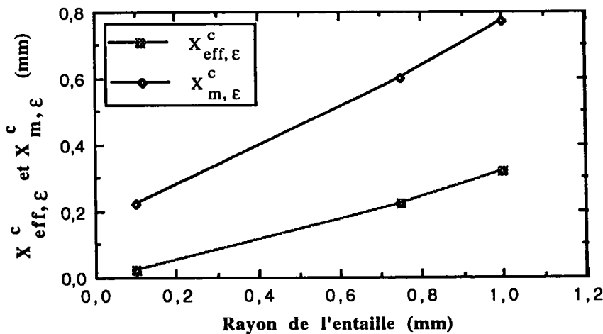
Figure 3.21 : Variation de X_{m,\varepsilon}^c et de X_{\text{eff},\varepsilon}^c en fonction de \rho . a = 44 mm.
