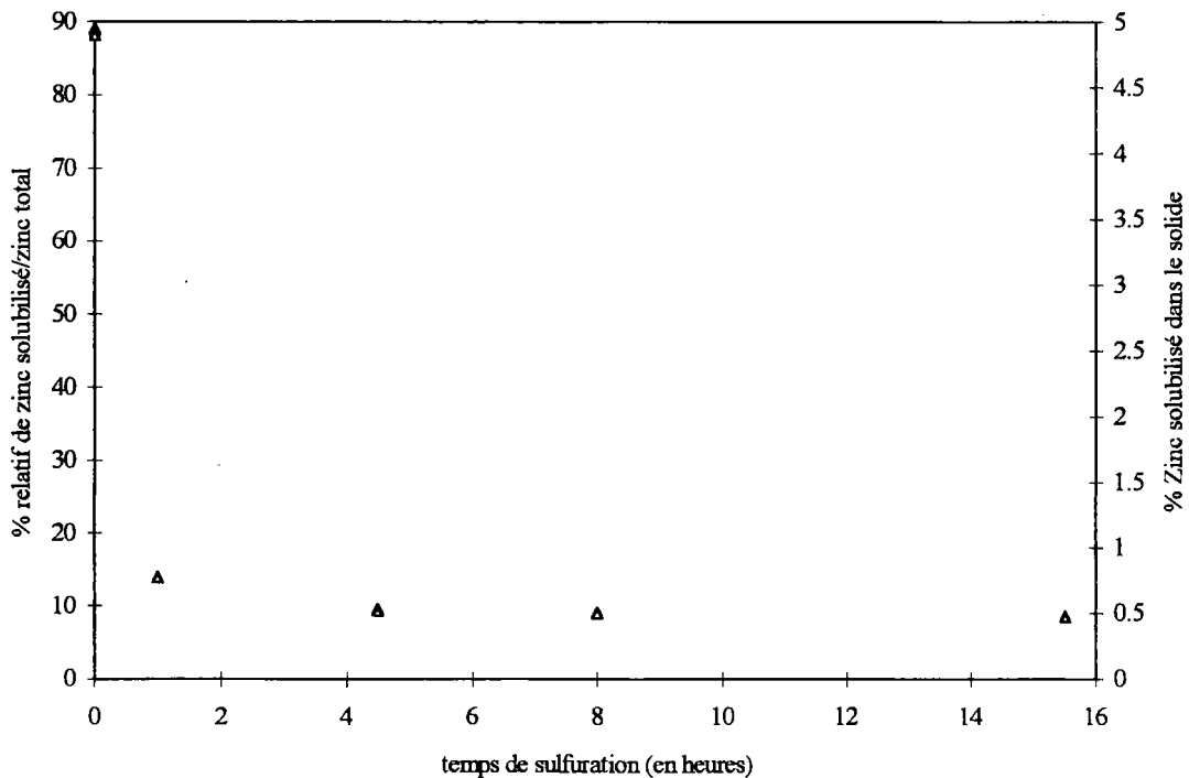
Figure 1.III.5 : Etude cinétique de l'inertage du gâteau d'hydroxydes métalliques issu de la coprécipitation d'un mélange fer-zinc. Taux de zinc mobilisable par l'acétate d'ammonium à 30 %. Etude à 70 °C.
