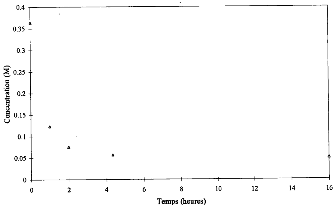
Figure 1.II.7 : Suivi de la concentration en polysulfures au cours de l'inertage
