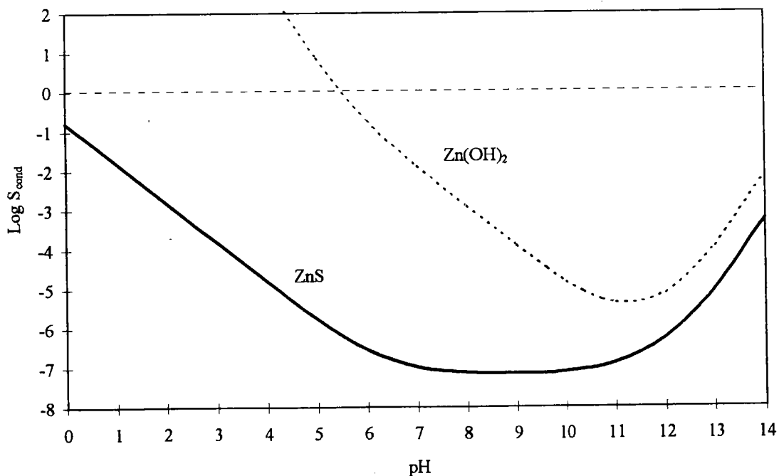
Figure 1.I.1 : Diagramme de solubilité de ZnS et ZnO en fonction de la variation de pH
