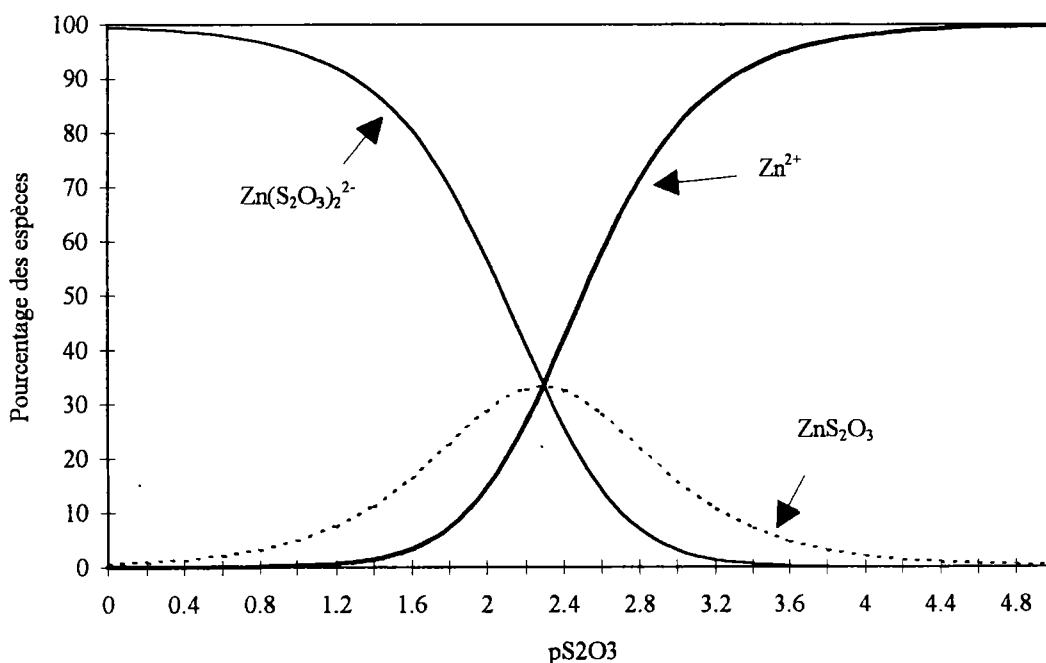
Figure 2.I.6 : Diagramme de répartition des complexes thiosulfates du zinc
