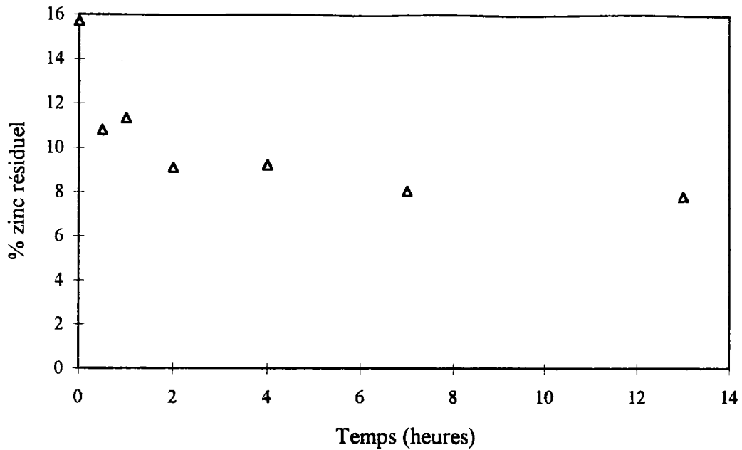
Figure 2.II.2 : Evolution de la teneur en zinc dans le résidu au cours du traitement par le thiosulfate d'ammonium à 4 M à 20 °C.
