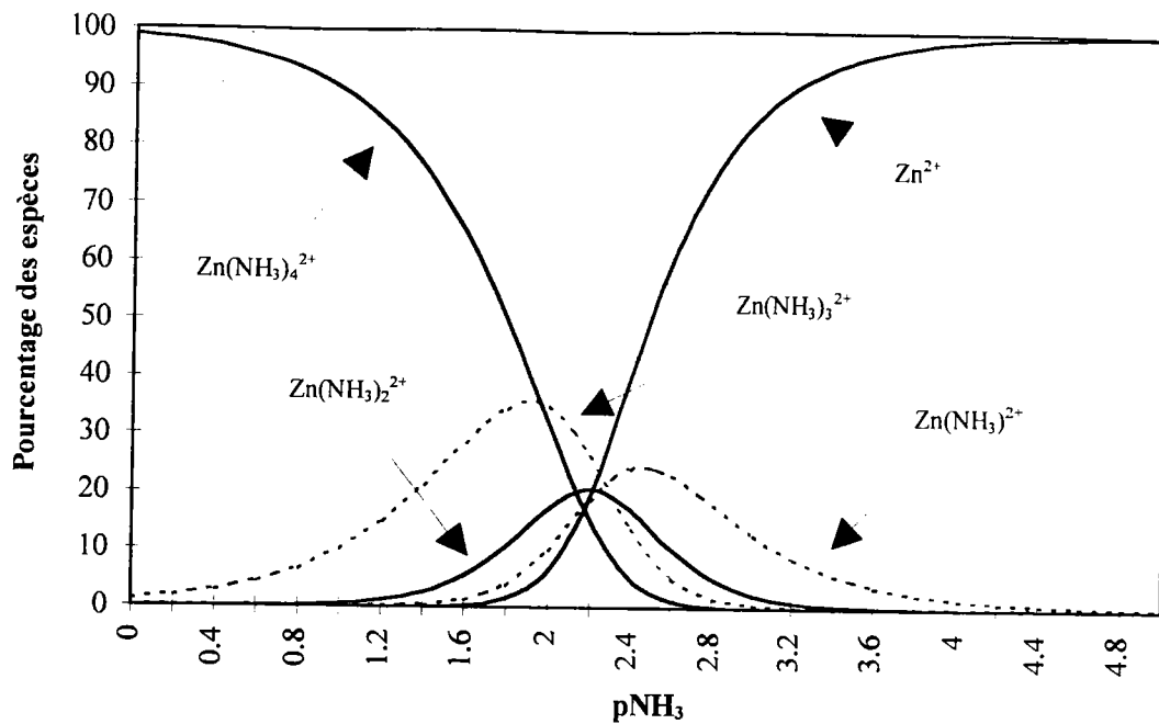
Figure 2.I.2 : Diagramme de prédominance des complexes ammines du zinc
