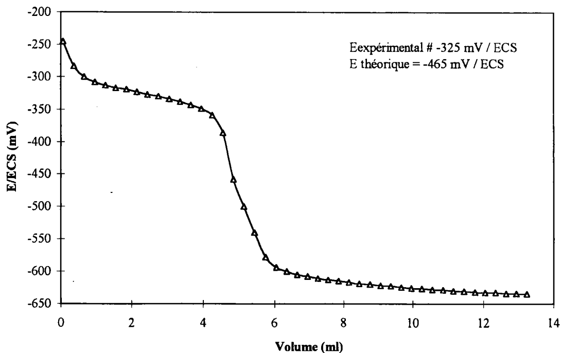
Figure 3.II.3 : Suivi du potentiel pris par une électrode d'argent plongeant dans 50 ml d'une solution de FeSO_4 à 5 \cdot 10^{-2} M au cours de l'ajout de polysulfures à 0,55 M.
