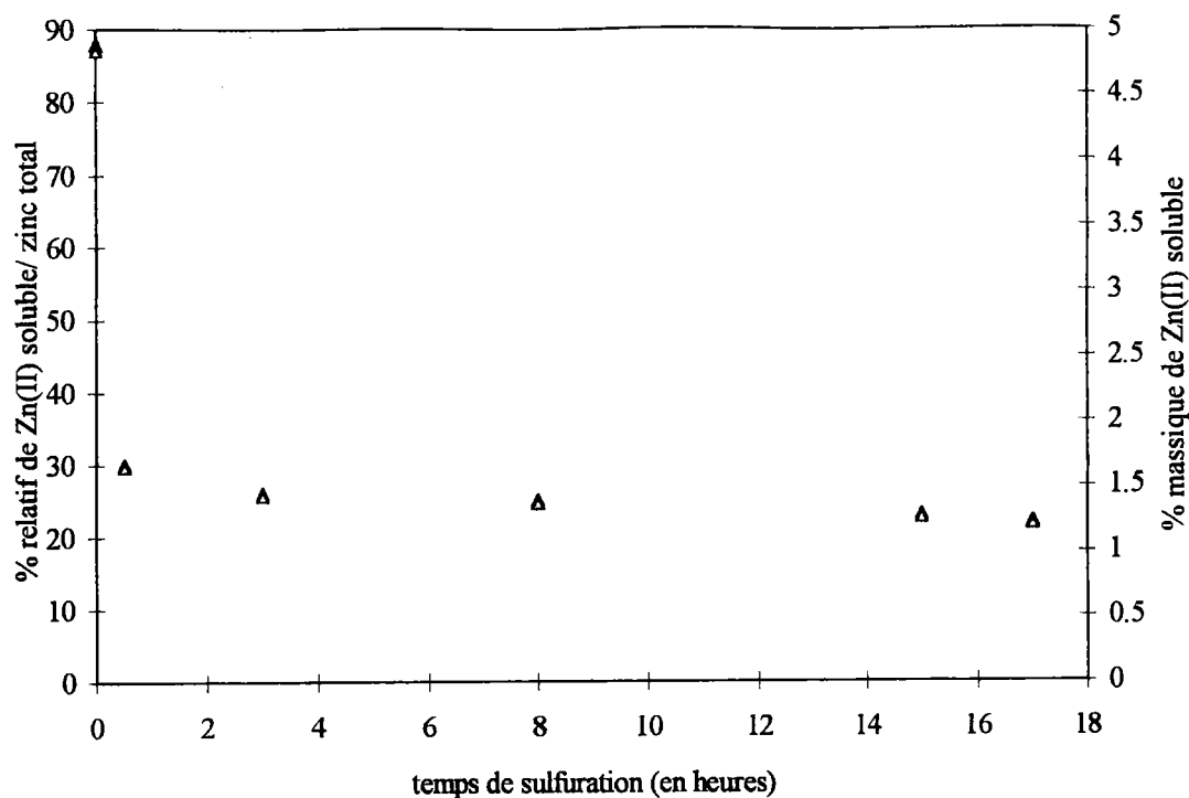
Figure 1.III.3 : Etude cinétique de l'inertage du gâteau d'hydroxydes métalliques issu de la coprécipitation d'un mélange fer-zinc. Taux de zinc mobilisable par l'acétate d'ammonium à 30 %.
