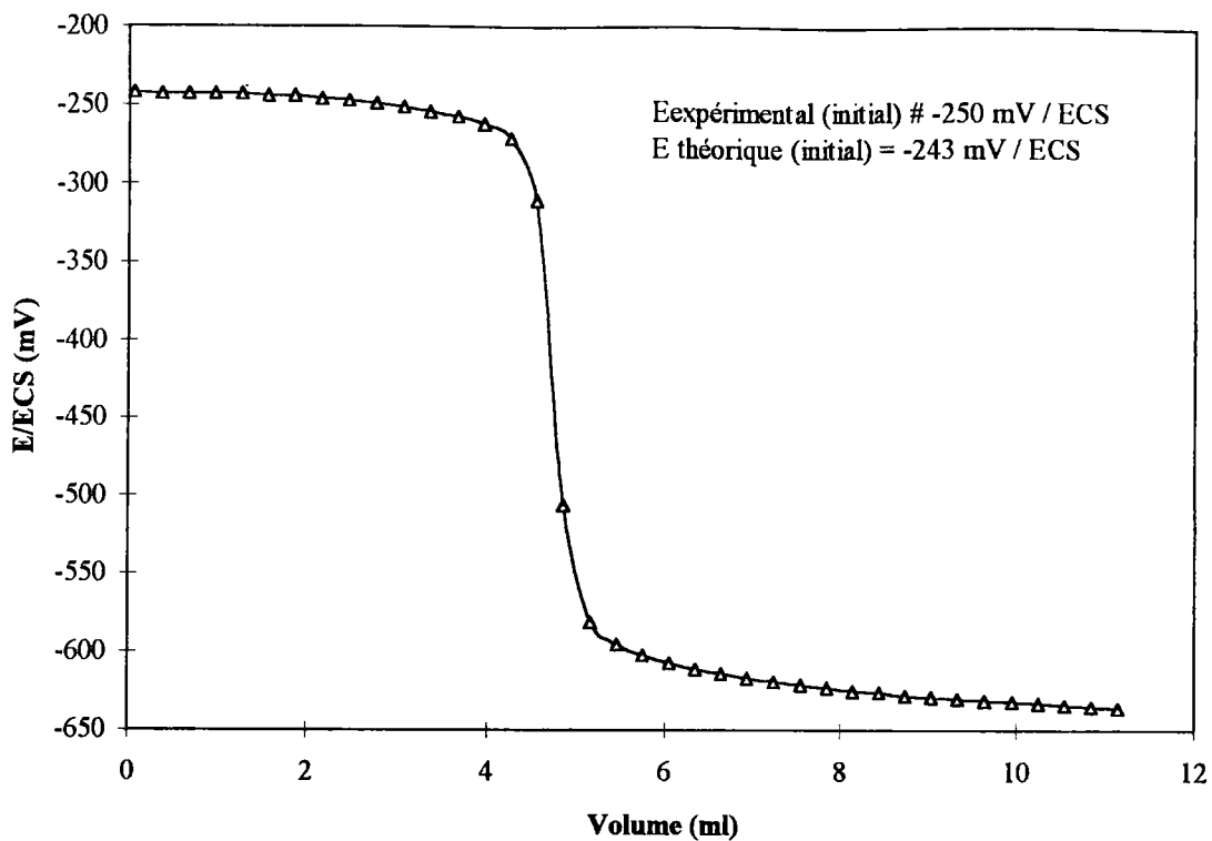
Figure 3.II.2 : Suivi du potentiel pris par une électrode d'argent plongeant dans 50 ml d'une solution de ZnSO_4 à 5 \cdot 10^{-2} M au cours de l'ajout de polysulfures à 0,55 M.
