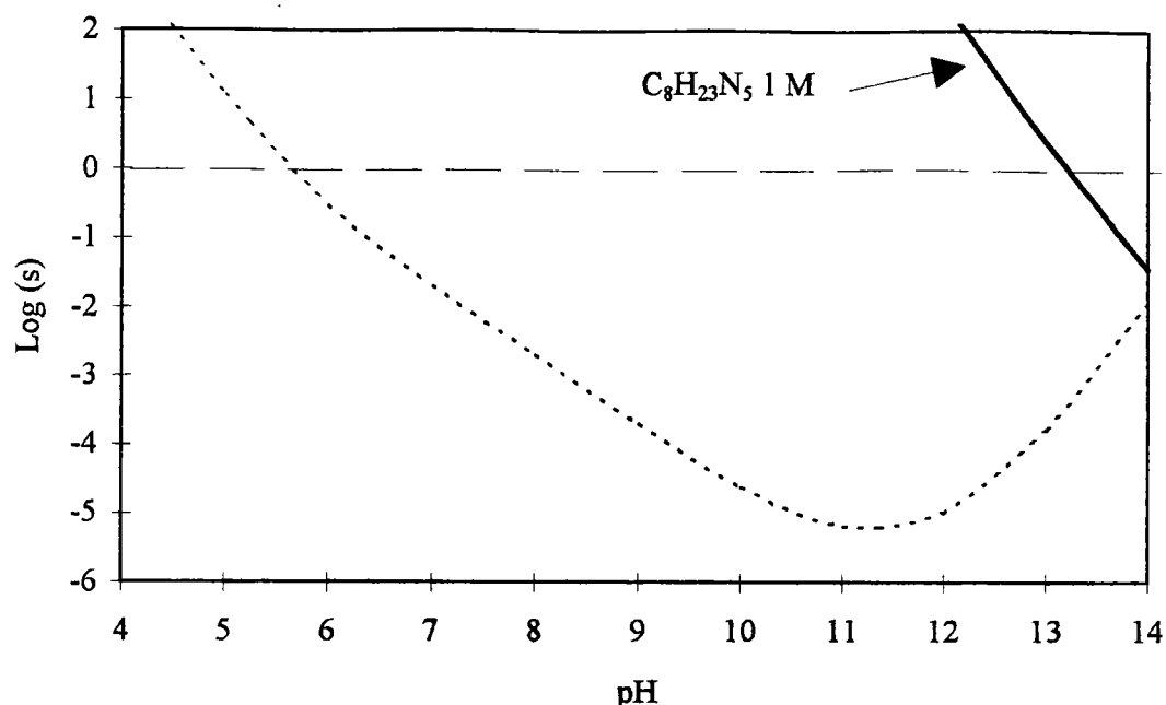
Figure 2.I.10 : Courbe de solubilité de Zn(OH)_2 en présence de tétraéthylènepentamine
