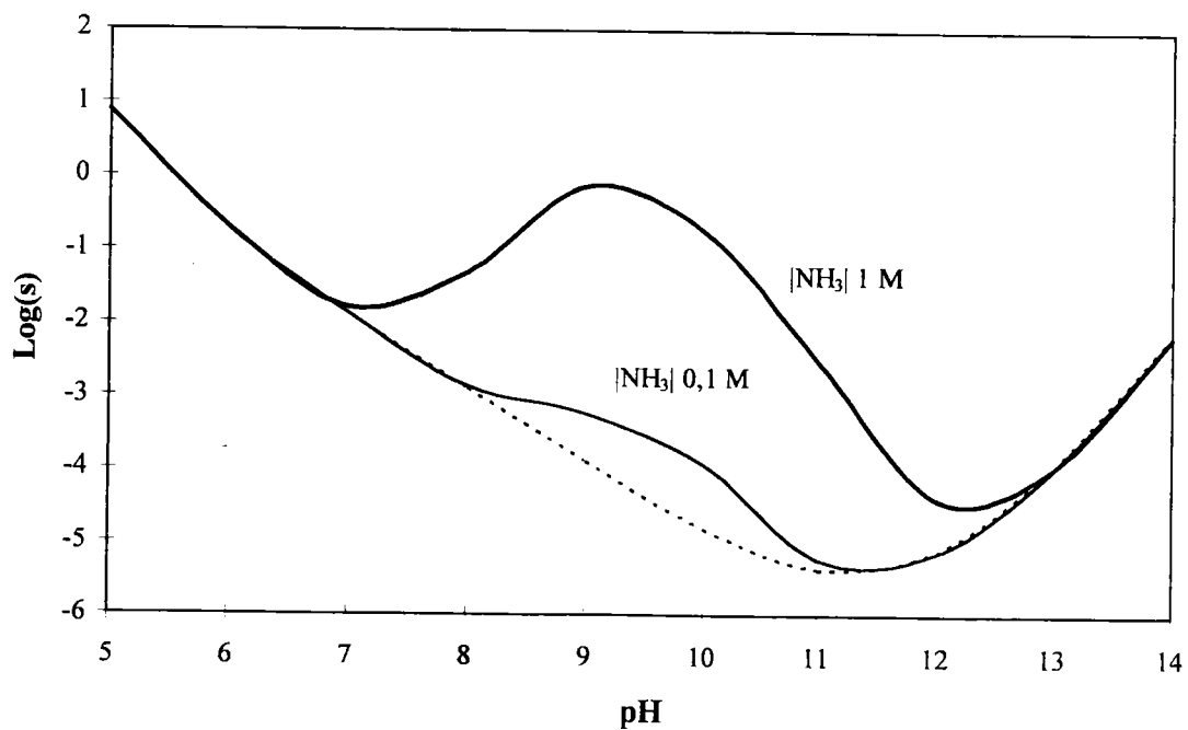
Figure 2.I.3 : Diagramme de solubilité en fonction du pH du zinc en milieu ammoniacal
