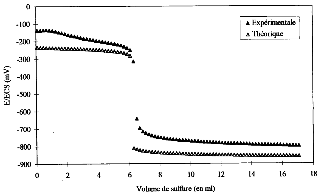
figure 3.I.5 : Suivi potentiométrique de la précipitation de ZnS.
