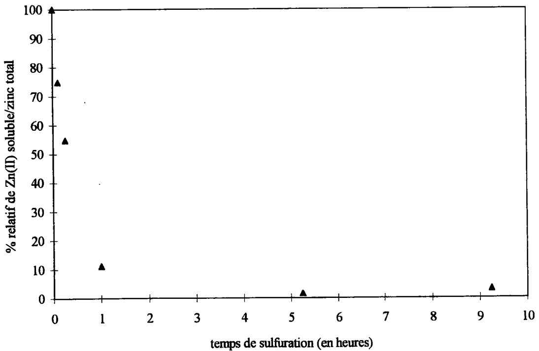
Figure 1.III.4 : Etude cinétique de l'inertage de l'hydroxyde de zinc. Taux de zinc mobilisable par l'acétate d'ammonium à 30 %.
