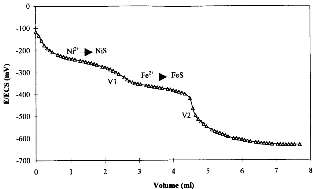
Figure 3.II.13 : Evolution du potentiel et du pH lors de l'ajout de polysulfures dans une solution contenant un mélange \text{Fe}^{3+} - \text{Zn}^{2+}
