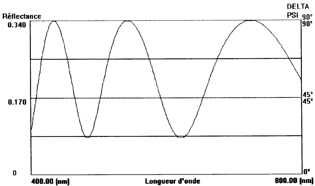
Fig.IIB.6.a : Représentation spectrale en longueur d'onde de la réflectance.
