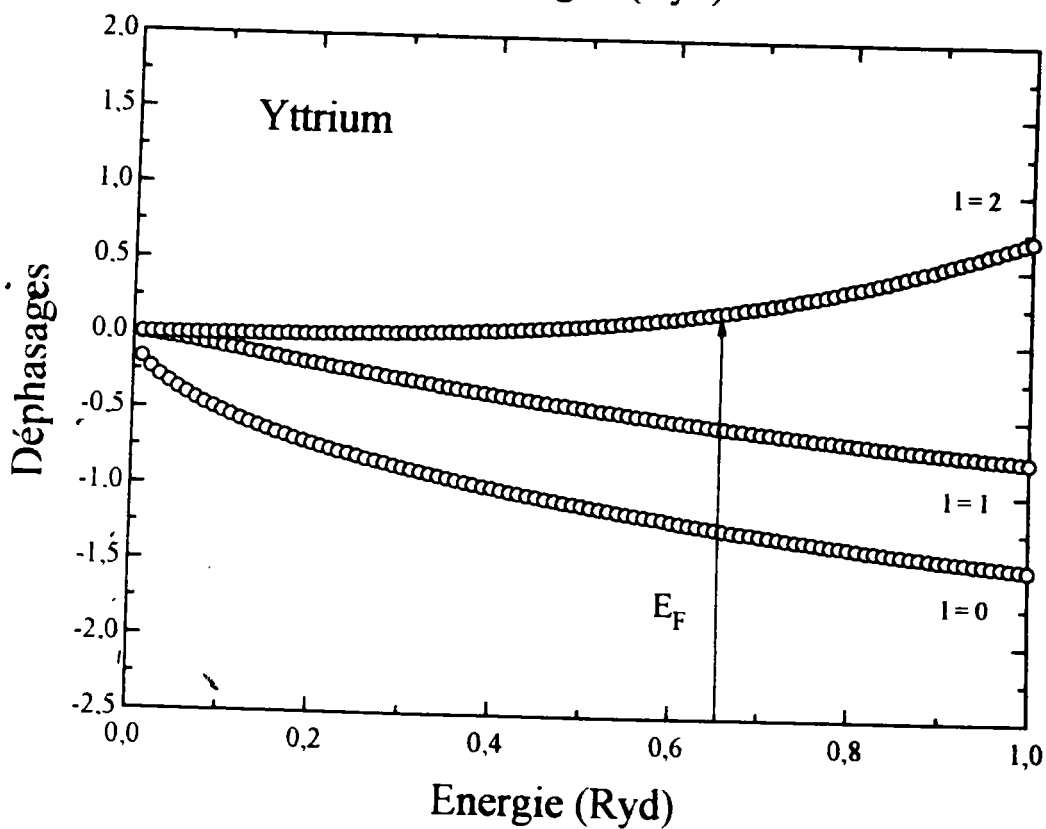
Figure F3. 2: Déphasages en fonction de l'énergie du nickel et de l'yttrium
