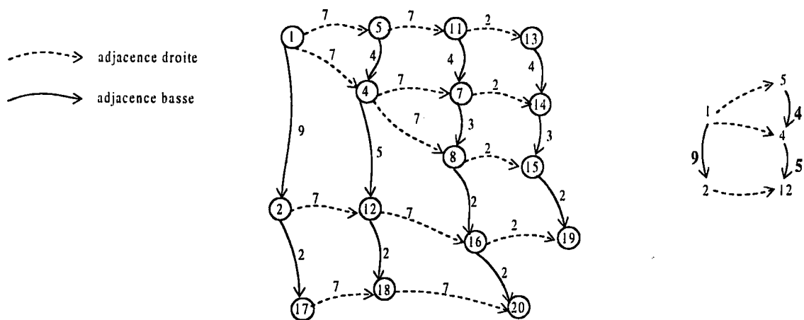
Figure 3.29. Conserver les longueurs des rectangles
