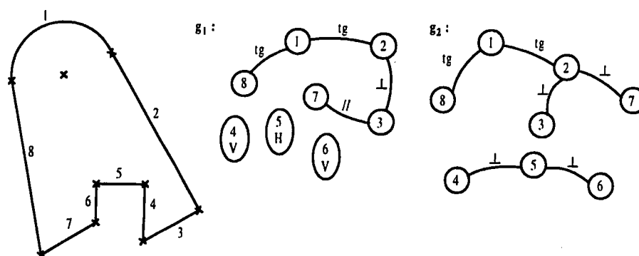
Figure 2.4. Deux graphes différents pour la même pièce
