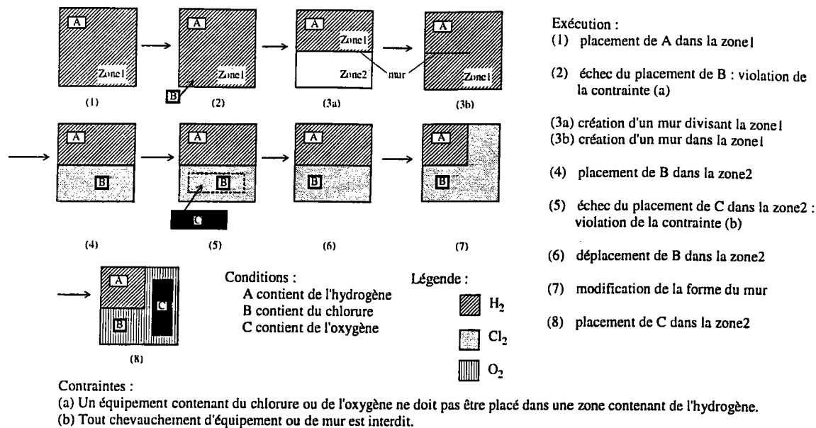
Figure 3.5. Exemple d'aménagement industriel
