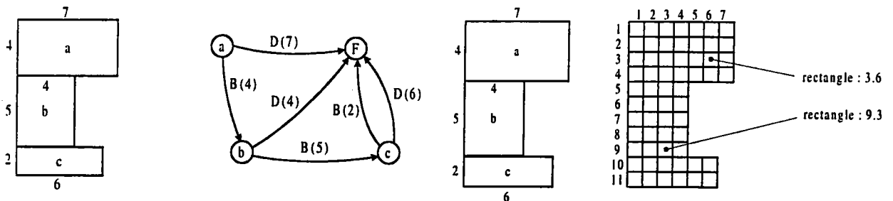
Figure 3.36. Modélisation d'un objet complexe Figure 3.37. Représentation unitaire de l'objet complexe
