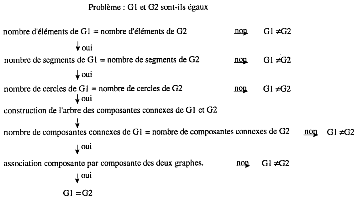
Figure 2.15. Algorithme d'égalité de deux graphes
