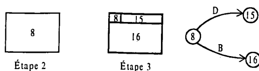
Figure 3.25. Déduction d'adjacence
