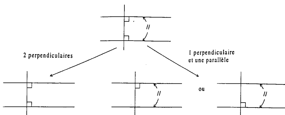
Figure 2.37. Redondance d'informations
