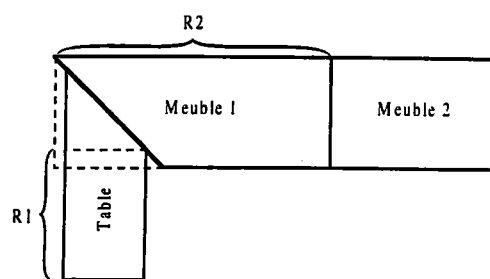
Figure 3.14. Configuration spéciale
