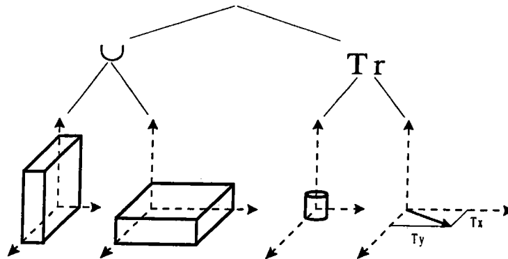
Figure A.2. Un arbre de construction CSG
