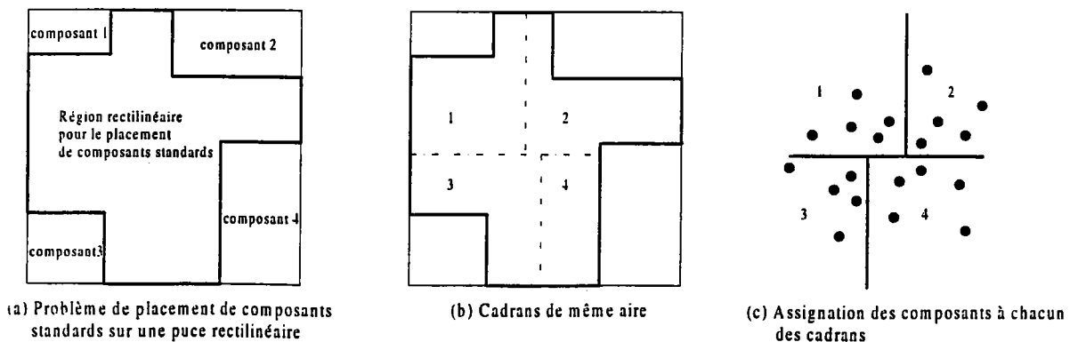
Figure 3.1. L'algorithme de croissance de groupe adaptatif
