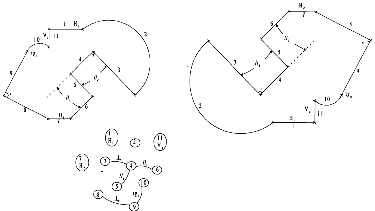
Figure 2.30. Pièces liées par des relations topologiques et géométriques
