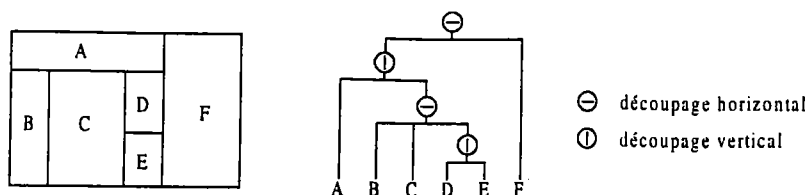
Figure 3.11. Arbre de partitionnement
