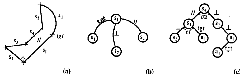
Figure 1.2. - (a) Représentation géométrique de l'objet- (b) Graphe de l'objet- (c) Arbre de construction-
