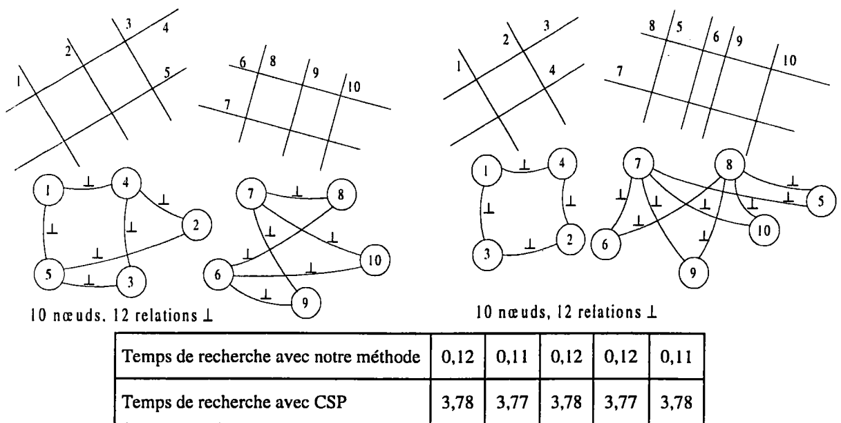
Figure 2.27. Comparaison CSP/méthode spécifique
