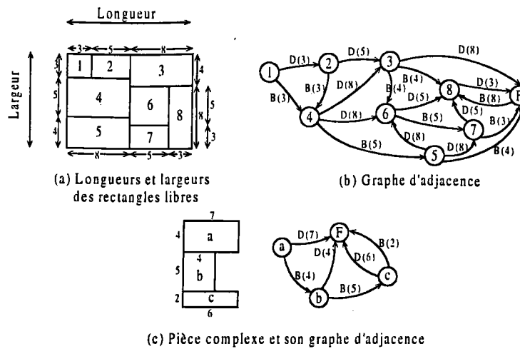
Figure 3.31. Modélisation de l'espace de placement et de l'objet à placer
