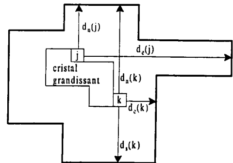
Figure 3.3. Directions d'accroissement
