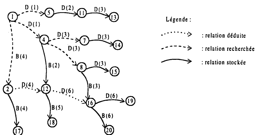
Figure 3.26. Graphe d'adjacence
