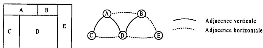
Figure 3.12. Graphe d'adjacence
