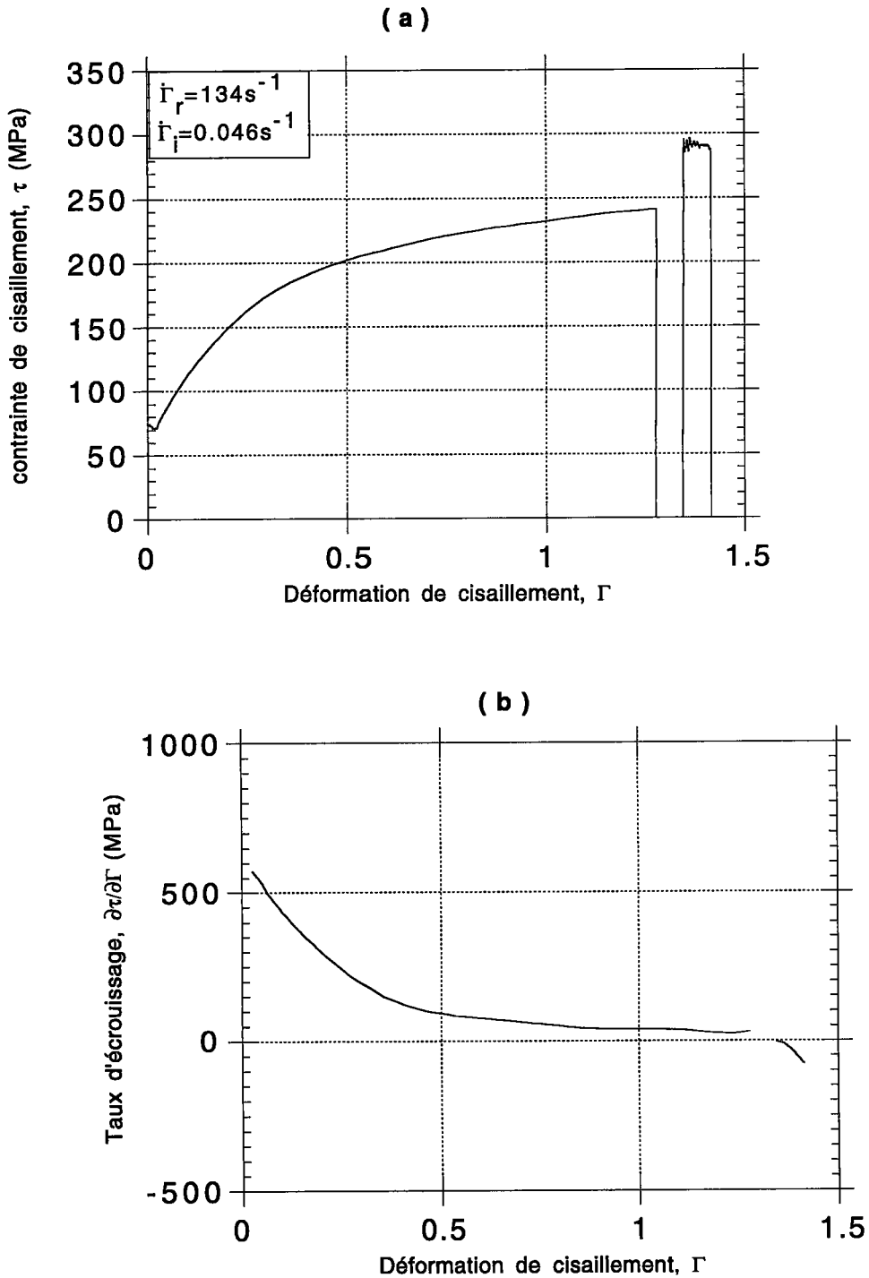
Figure (IV. 17): Résultats d'un essai de saut de vitesse de \dot{\Gamma}_i = 4.6 \times 10^{-2} s^{-1} à \dot{\Gamma}_r = 134 s^{-1} , sur éprouvette deux fois chargée à vitesse élevée après une pré-déformation \Gamma_i = 1.25 sur les barres de Kolsky, (a) courbe contrainte-déformation, (b) courbe taux d'écroissage-déformation.
