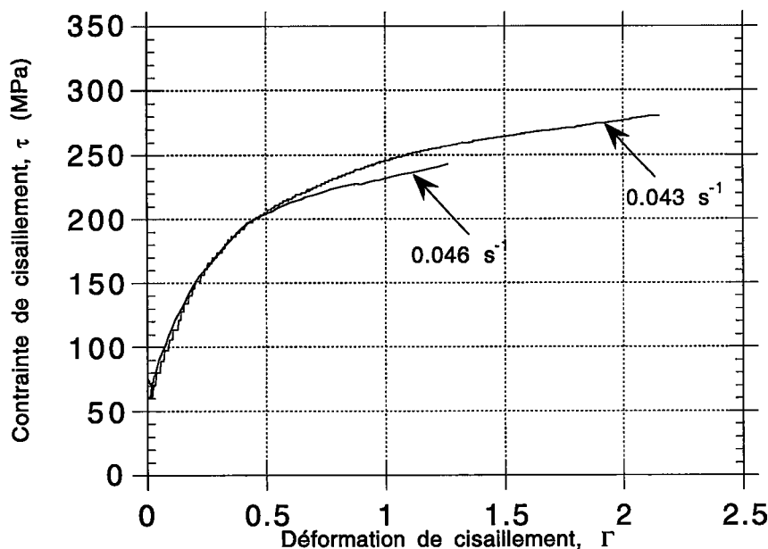
Figure (IV. 2): Courbes contrainte-déformation quasi-statiques sur machine de Zwick à la vitesse \dot{\Gamma} = 4,3 \times 10^{-2} \text{s}^{-1} et sur les barres de Kolsky à la vitesse \dot{\Gamma} = 4,6 \times 10^{-2} \text{s}^{-1} .
