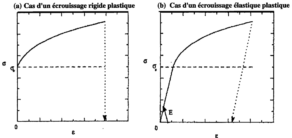
Figure(I. 2): Évolution de la contrainte en fonction de la déformation dans le cas d'un comportement unidimensionnel avec écoulement non linéaire.
