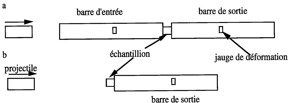
Figure (II. 2): Diagramme schématique du dispositif de Kolsky pour l'analyse des ondes de compression, (a) [64], (b) [75].
