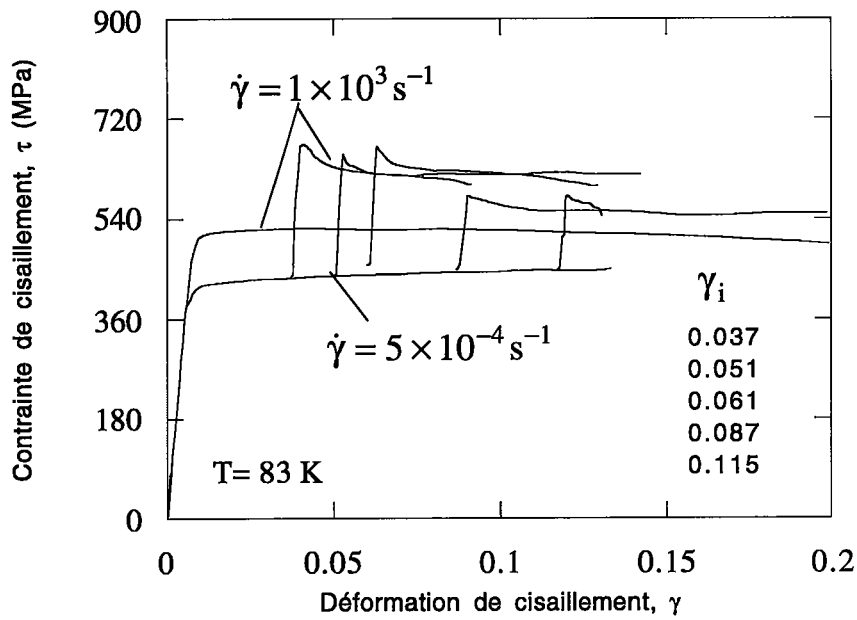
Figure(I. 7): Résultats des essais aux vitesses constantes et des sauts de vitesse de l'acier doux 1020 (HRS) à T=83K, Klepaczko et al.,[17].
