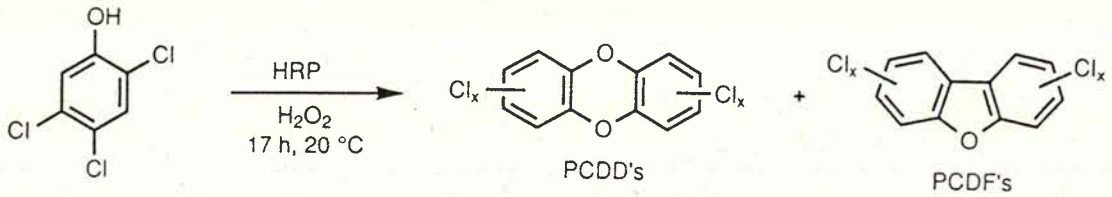
Figure 1.2 : Formation de PCDDs et PCDFs par biohalogénéation du 2,4,5 trichlorophénol (Svenson et al. , 1989).
