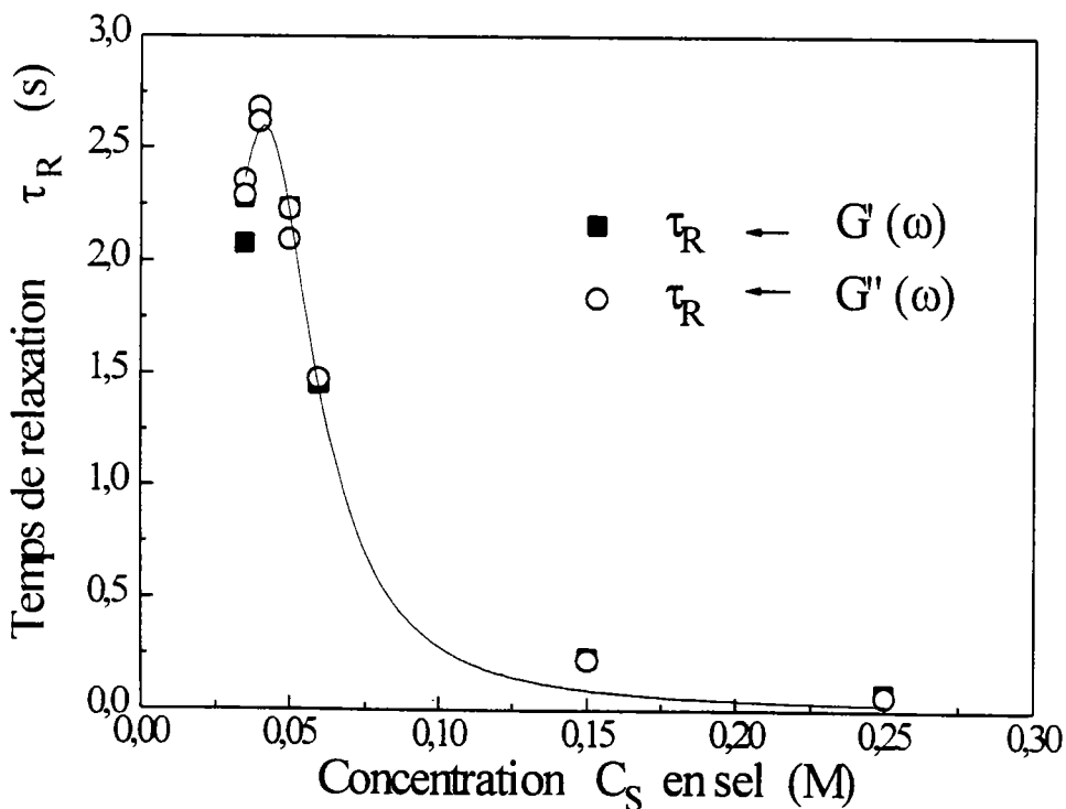
Figure IV.24 - Evolution du temps de relaxation \tau_R en fonction de la concentration en NaTos pour une solution de CTAB 0.05 M ( T = 24^\circ\text{C} ).
