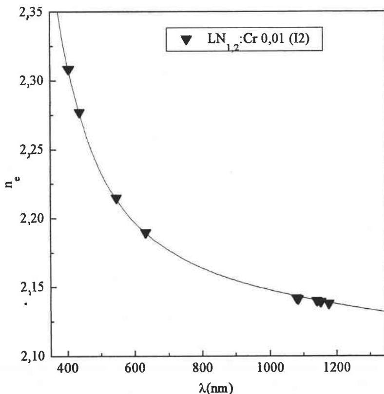
Figure II.12: Indice de réfraction extraordinaire n_e de l'échantillon LN 1,2 :Cr 0,01 en fonction de la longueur d'onde. La ligne représente la courbe d'ajustement de Sellmeier.
