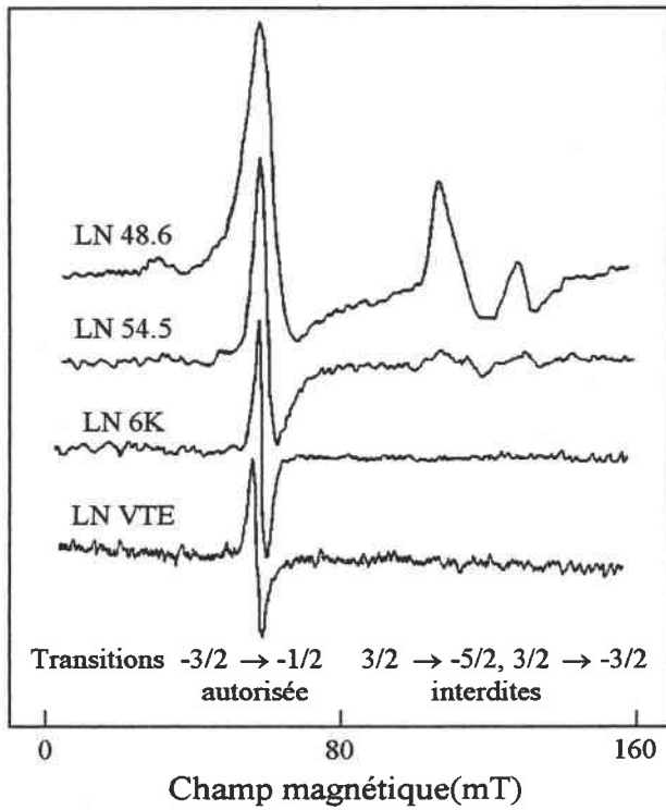
Figure II.2: Pics RPE des ions Fe^{3+} dans les cristaux de LiNbO_3 de plusieurs compositions pour un champ magnétique faible B//c et une fréquence micro-onde \nu = 9,018 GHz à température ambiante.
