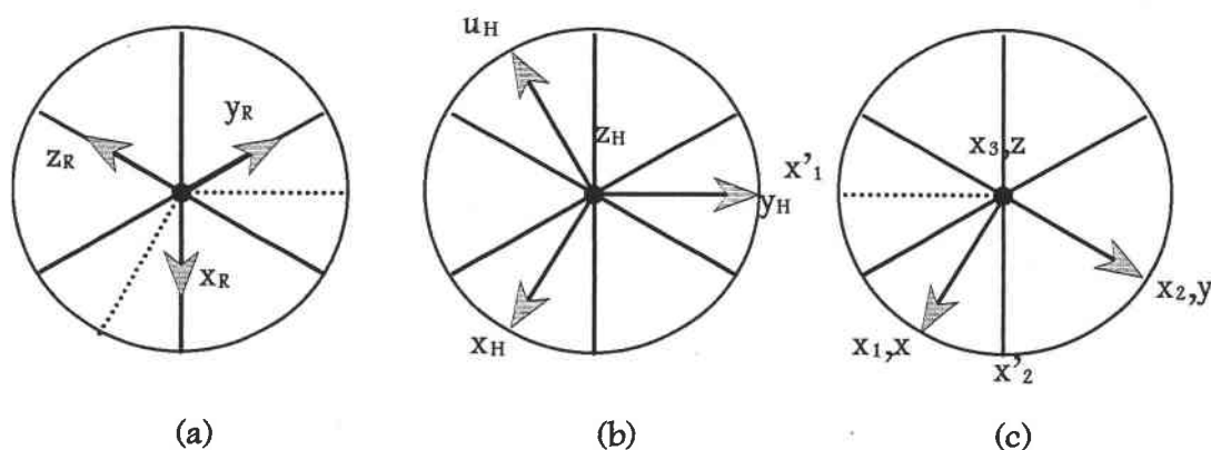
Figure I.6: Convention d'axes dans LiNbO_3 .
