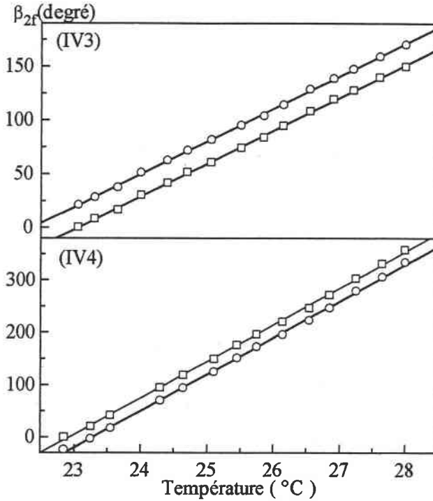
Figure III.9: Evolution de l'angle de \beta_{2f} en fonction de la température pour les échantillons LN_{1,15}:Cr\ 0,02 (IV3) et LN_{1,5}:Cr\ 0,02 (IV4).
