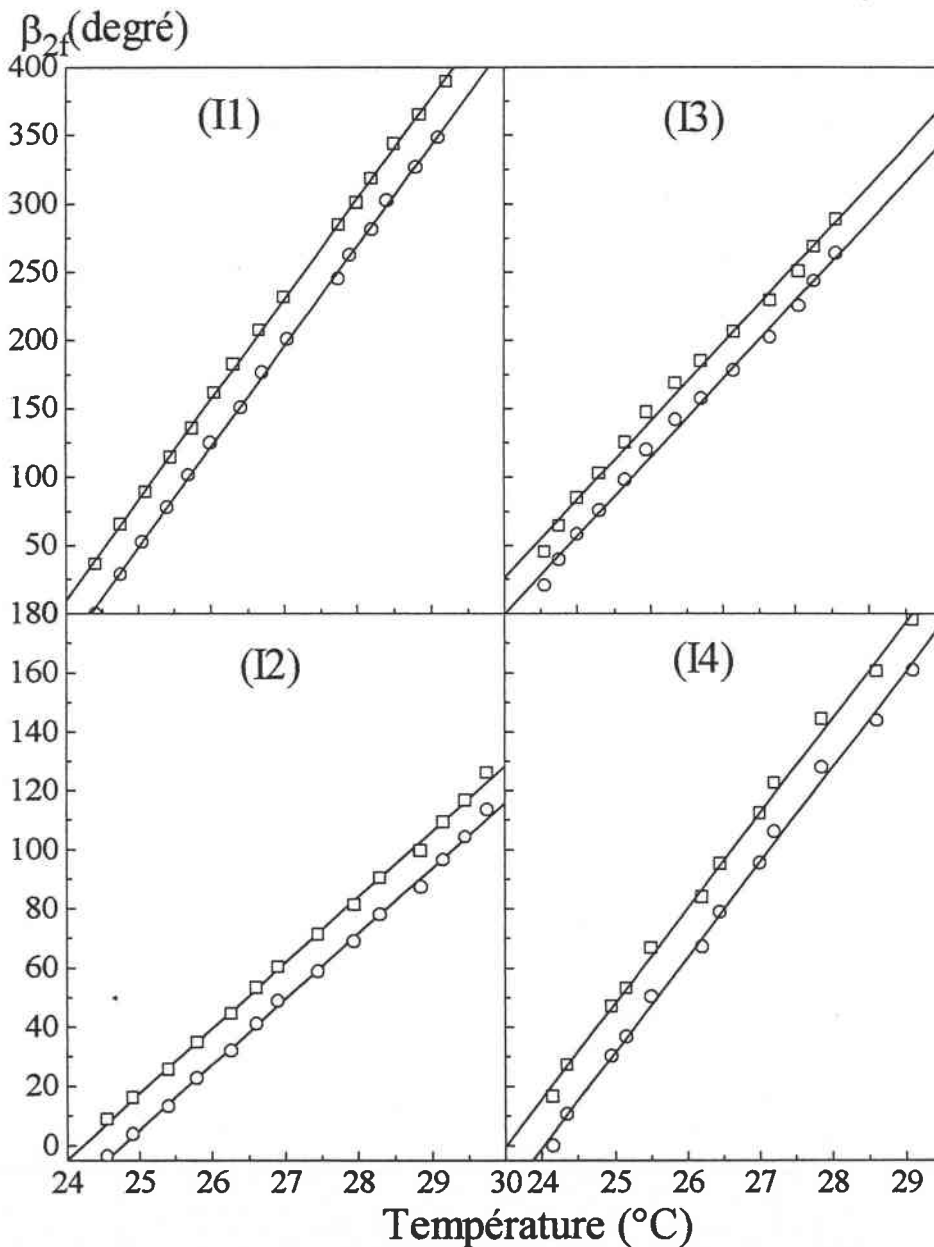
Figure III.3: Variation de l'angle \beta_{2f} en fonction de la température, (O) 0 V et ( \square ) 428V de tension dc appliquée, pour les échantillons \text{LN}_{1,2}:\text{Cr} 0 (I1), \text{LN}_{1,2}:\text{Cr} 0,01 (I2), \text{LN}_{1,2}:\text{Cr} 0,05 (I3) et \text{LN}_{1,2}:\text{Cr} 0,275 (I4). Les lignes correspondent aux droites d'ajustement des points expérimentaux.
