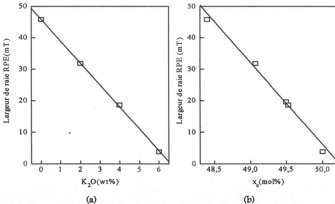
Figure II.3: Dépendance de la largeur des raies RPE de Fe^{3+} en fonction de: (a) la concentration du potassium introduite dans le bain, (b) la composition x_c des échantillons. Pour un champ magnétique B \perp c et une fréquence micro-onde \nu = 9,018 GHz à 14K de la raie à 300 mT.
