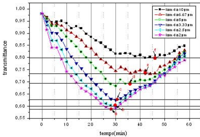
Figure IV-14 : Evolution temporelle de transmittance et minima aux différentes longueurs d’onde
