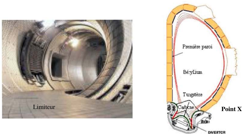
Figure I-4 : Photographie du limiteur dans Tore Supra [1] Figure I-5 : Schéma du divertor dans ITER [1]
