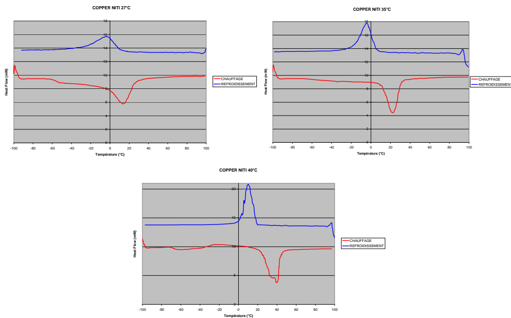
Figure 18 : Courbes de DSC des fils Copper NiTi 27°C (en haut à gauche), Copper NiTi 35°C (en haut à droite), Copper NiTi 40°C (en bas)
