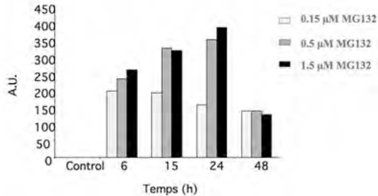
Figure 53 : A : Cinétique d'induction d'Hsp27 dans les chondrocytes de rat par le MG132. Les chondrocytes ont été exposés à différentes concentrations de MG132 (0,15 ; 0,5 et 1,5 μM). Différents temps après la mise en contact, les protéines totales ont été extraites et dosées par la méthode de Bradford. La protéine Hsp27 a été détectée par western-blot avec un anticorps spécifique d'Hsp27 (n = 3 expériences indépendantes). B : Le niveau d'expression de la protéine Hsp27 a été évalué par analyse densitométrique de chaque bande obtenue en western blot et les résultats ont été exprimés en unités arbitraires.
