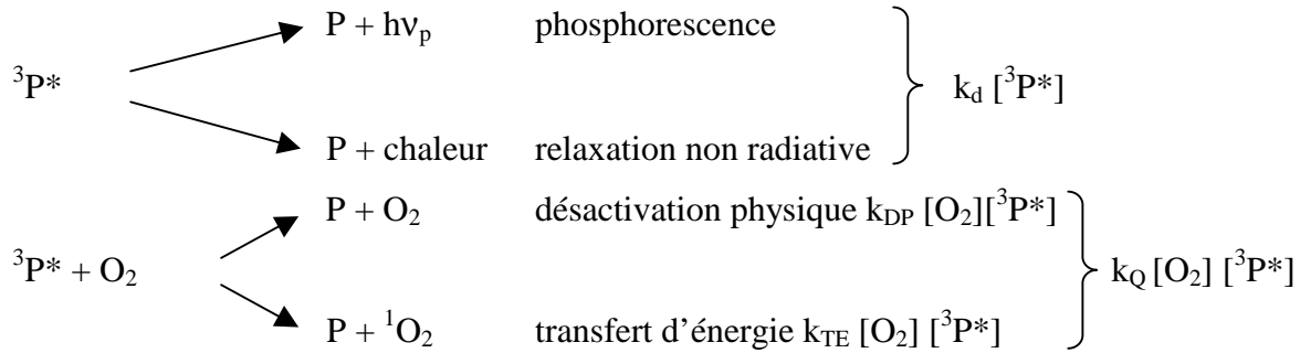
Figure 2: Processus physiques et chimiques impliquant le photosensibilisateur à l'état triplet excité ^3\text{P}^* , avec leurs constantes respectives : k_d constante de désactivation de ^3\text{P}^* , k_{\text{DP}} constante de désactivation physique, k_{\text{TE}} constante de transfert d'énergie, k_Q constante d'interaction de ^3\text{P}^* avec \text{O}_2 , k_Q = k_{\text{DP}} + k_{\text{TE}} .
