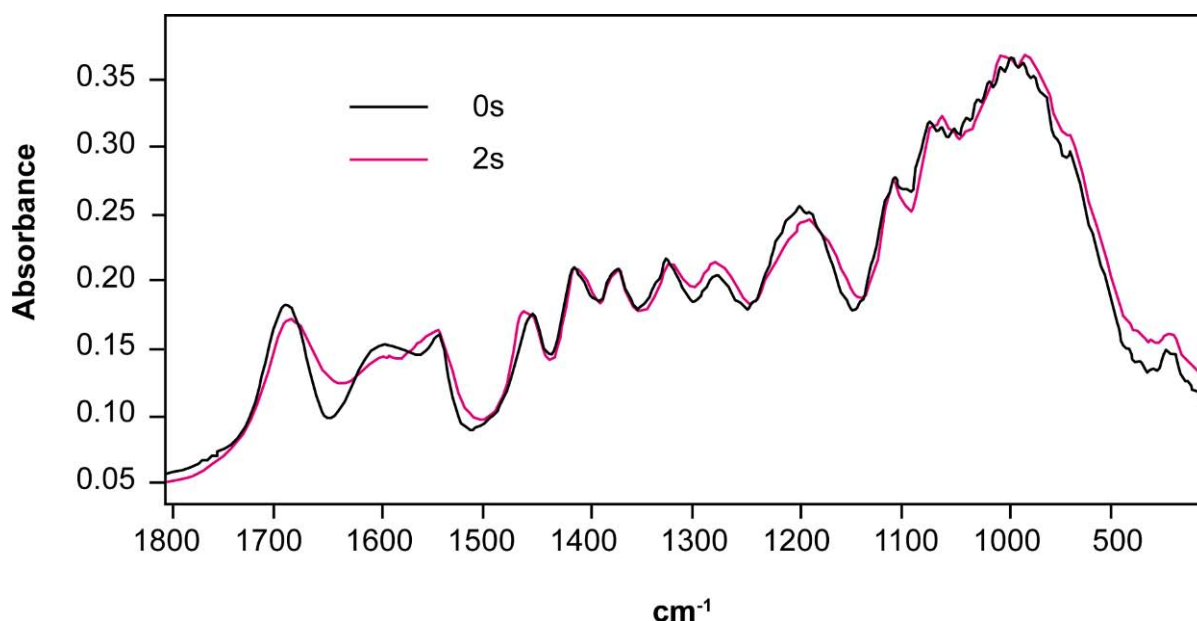
Figure 80: Variations des bandes FT-IR de l'interface soudée dans le domaine 2600\text{-}850\text{ cm}^{-1} en fonction du temps de soudage (0 s et 2 s).
