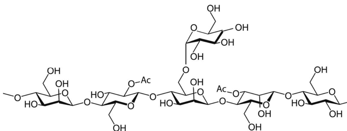
Figure 7: Structure chimique partielle d'un mannane de résineux (O-acetyl-galactoglucomannane).
