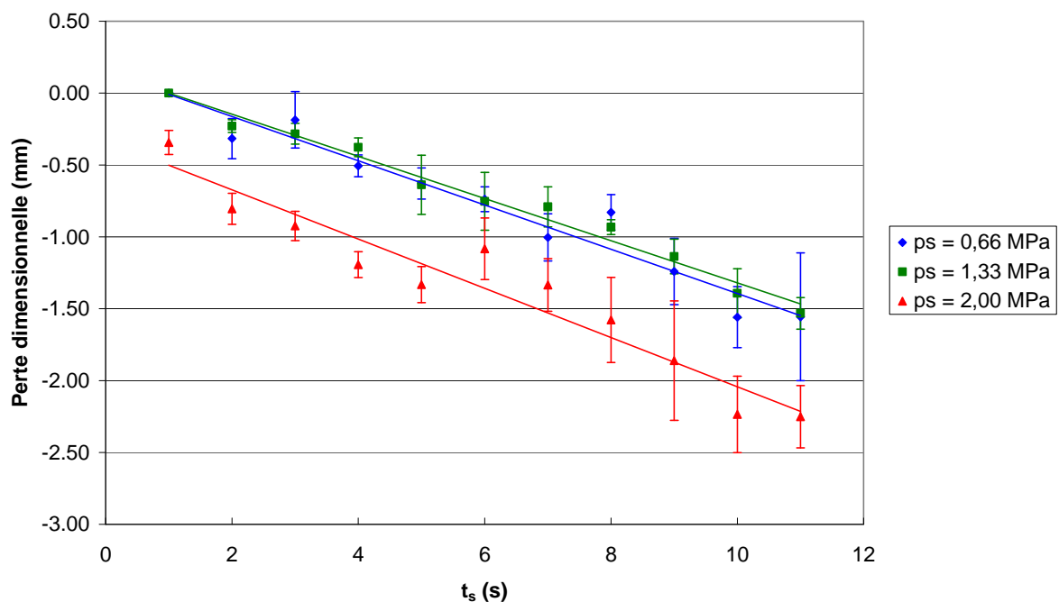
Figure 66: Evolution moyenne de la perte dimensionnelle en fonction du temps de soudage ( t_s ) et de la pression de soudage ( p_s ). Les indicateurs correspondent aux écarts-types de chacune des moyennes.
