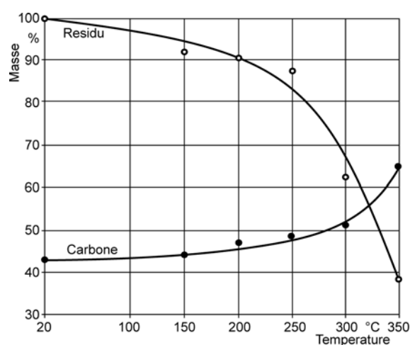
Figure 13: Perte de masse et teneur en carbone de Fagus sylvatica après un traitement thermique progressant de 5^\circ\text{C} par minute (selon Košík et al. 1969).
