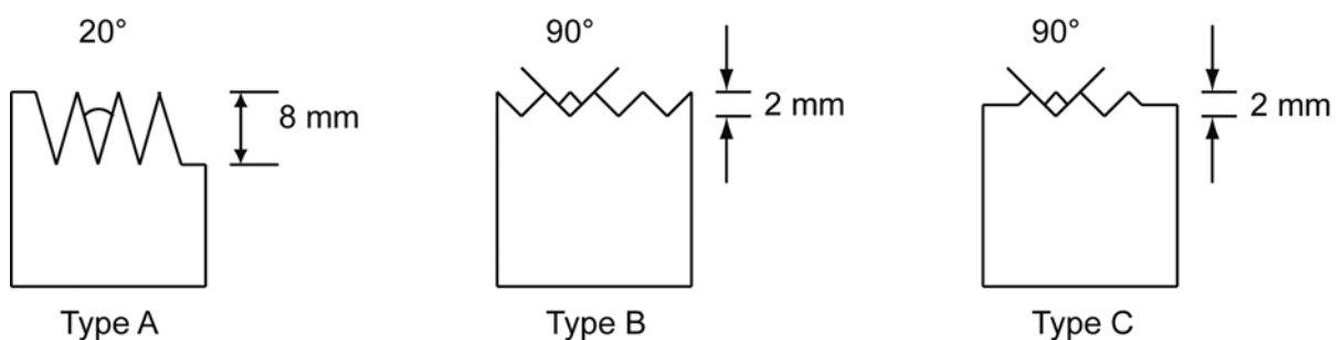
Figure 29: Schéma des types A, B et C de profils testés pour le soudage par friction linéaire.
