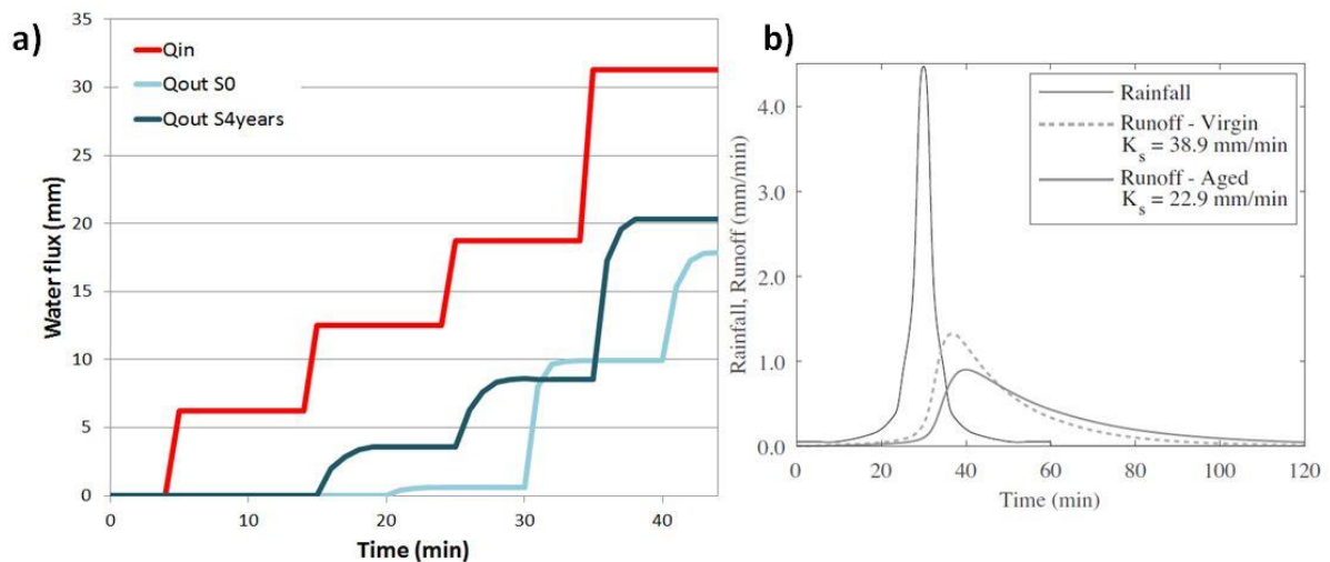
Figure 61. a) Courbes cumulées des précipitations ( Q_{in} ) et flux d'eau sortant d'un substrat neuf ( Q_{out\ S0} ) et d'un substrat évolué ( Q_{out\ S4years} ) ; b) Courbes instantanées des flux de précipitations (Rainfall), d'eau sortant d'un substrat neuf (Runoff - Virgin) et d'un substrat évolué (Runoff - Aged) (De Ville et al., 2017)
