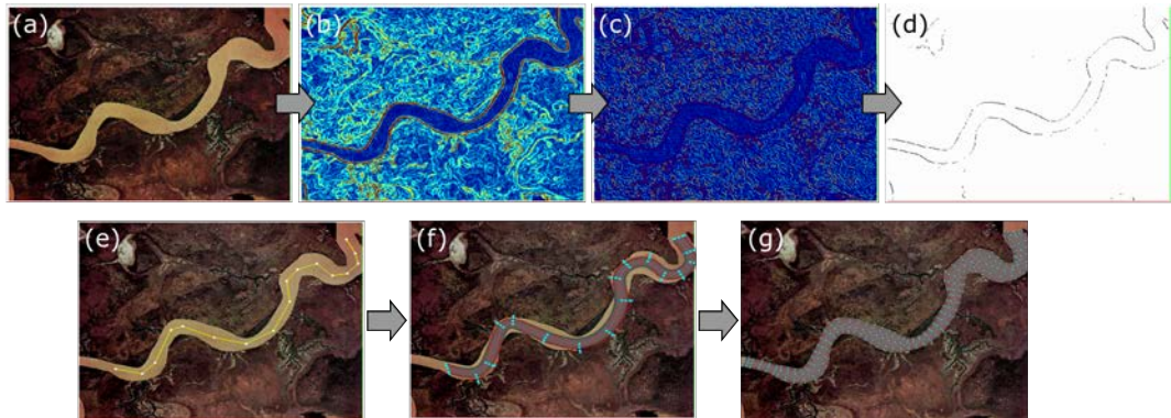
Figure 7 Détection automatique de formes géologiques par application de divers filtres d'analyse d'images et déformation d'objets NURBS. a Image satellite b Détection de bords c Affinement des bords d Seuillage des bords e Interprétation manuelle de la ligne centrale du chenal f Création d'un volume NURBS g Déformation du volume pour atteindre les bords détectés. Modifié d'après [Ruiu, 2015] South Alligator river, Australia [Google Earth, 2012]
