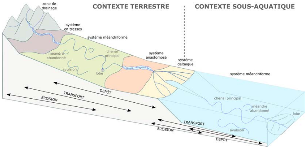
FIGURE 1 Schéma général des contextes de dépôts alluviaux depuis la zone de drainage jusqu'à la mer. De nombreux systèmes chenalisés s'y succèdent. Parmi eux les systèmes méandriformes se rencontrent en contexte fluvial et sous-marin. Les mêmes structures s'y retrouvent (p. ex. chenal principal, méandres abandonnés, avulsion, lobe, levée, barre d'accrétion latérale)
