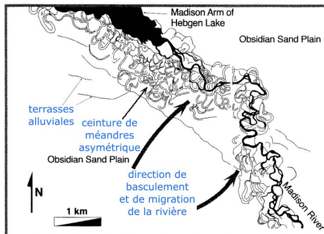
Figure 6 La migration d'un chenal est influencée par la tectonique régionale. Modifié d'après [Burbank and Anderson, 2000].
