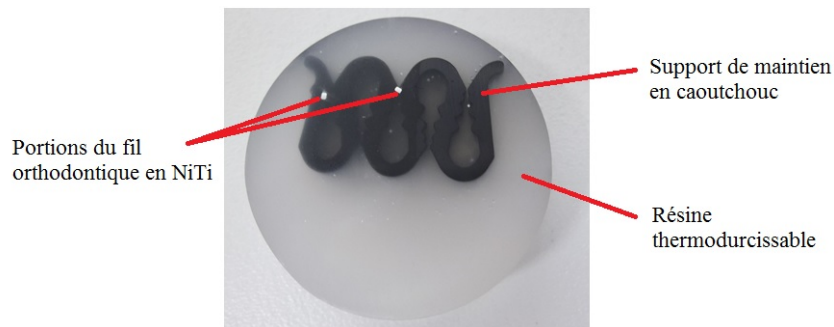
FIGURE 2.13 – Échantillon en NiTi superélastique enrobé en résine thermosable Mécaprex.
