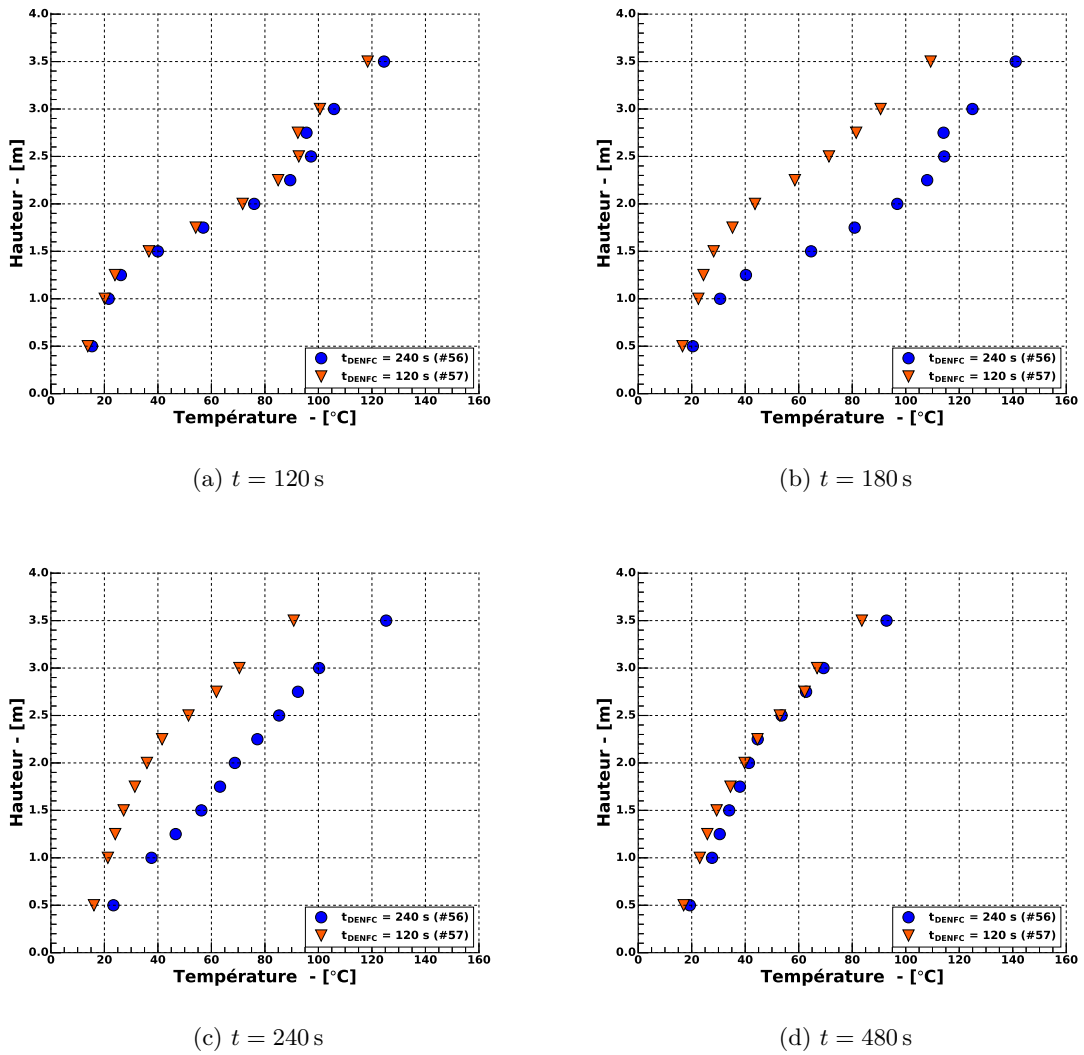
FIGURE 2.18 – Profils de température à différents instants pour 2 scénarios différents (foyer de 800 kW). En bleu : ouverture de l'exutoire 60 s après aspersion. En orange : ouverture de l'exutoire 60 s avant aspersion.
