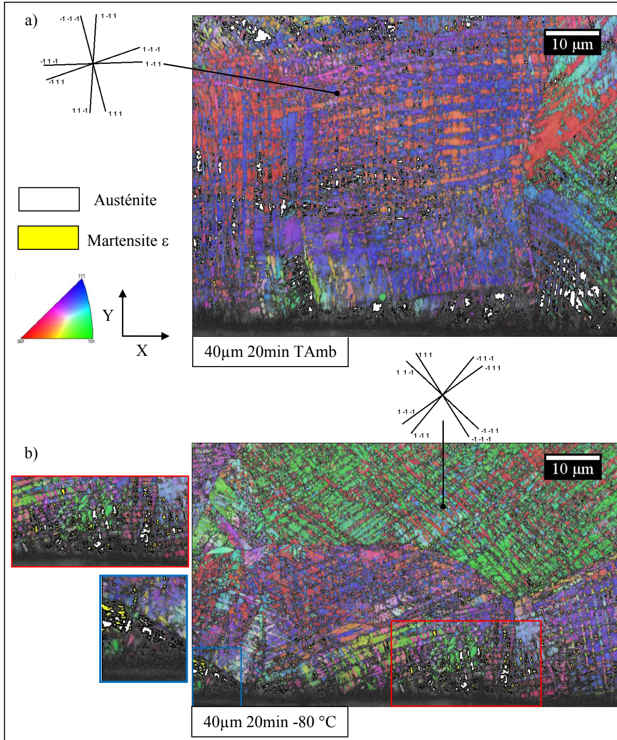
Figure 4.12 Cartographie d'orientation acquises en extrême surface des échantillons 304L a) 40µm 20min T Amb et b) 40µm 20min -80 °C. L'austénite est représentée en blanc la martensite \epsilon en jaune et la martensite \alpha' en coloration de figure de pôle inverse selon l'axe Y. Les vues de détail à gauche de la Figure 4.12b sont des zones où l'austénite résiduelle et la martensite \epsilon sont particulièrement visibles en extrême surface. Les deux surfaces présentent
