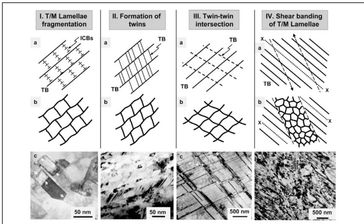
Figure 1.25 Schéma de l'affinement structural par maclage pour les matériaux de faibles EFE avec une schématisation a) des processus d'affinement, b) des structures affinées obtenues ainsi que c) les images électroniques associées. La colonne I correspond à un cuivre pur traité par SMAT, la II à un cuivre déformé par galetage, la III à un alliage 304 traité par SMAT et la IV à un cuivre pur déformé dynamiquement à température cryogénique [Tao et Lu - 2009]
