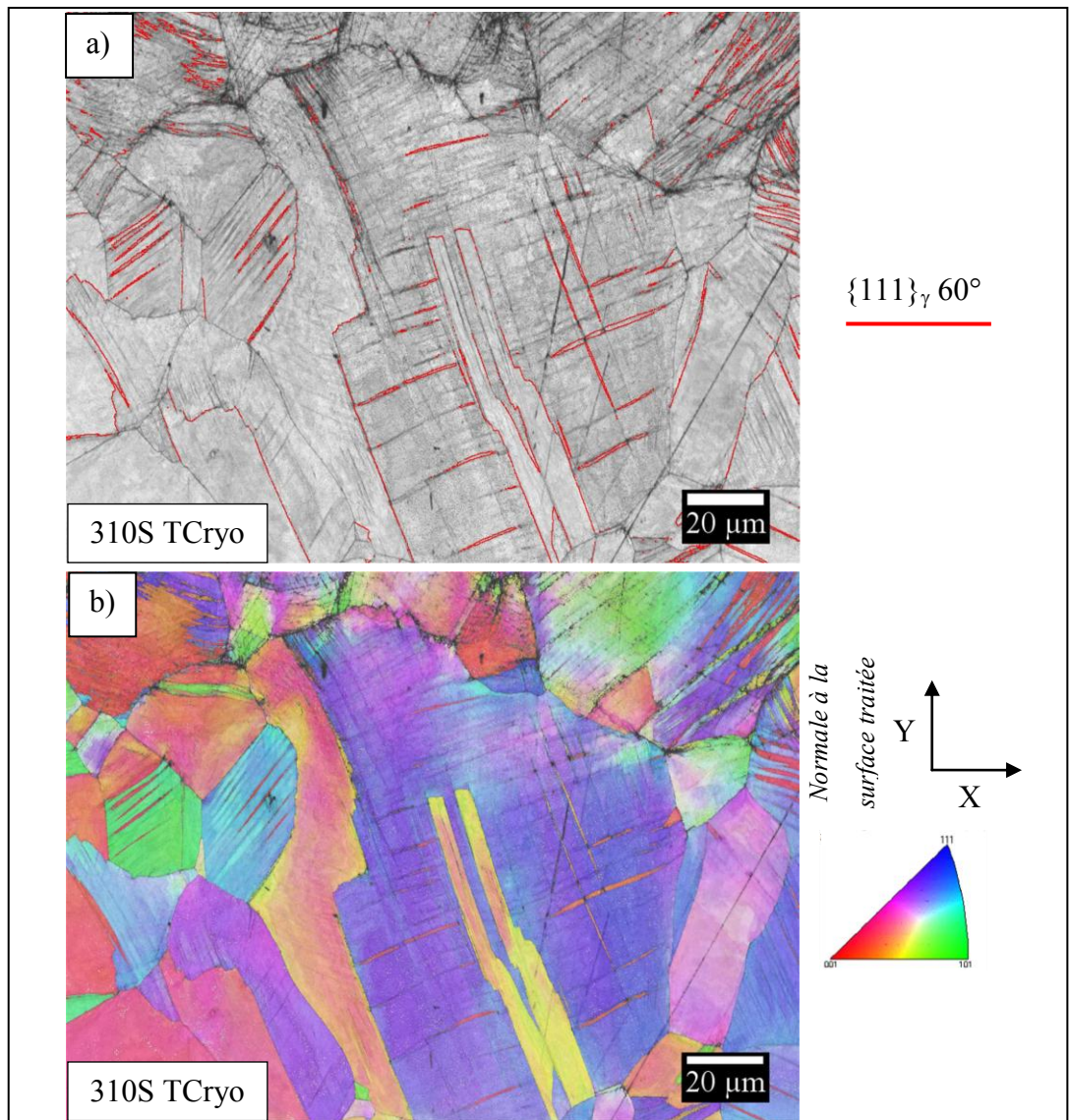
Figure 3.3 Cartographies d'orientation EBSD obtenues à une profondeur de 230 \mu\text{m} pour l'alliage 310Straité sous condition cryogénique avec a) l'austénite représentée en contraste de bande et la relation d'orientation de macle 60^\circ \langle 111 \rangle en rouge et b) l'austénite en coloration de figure de pôle inverse selon l'axe Y
