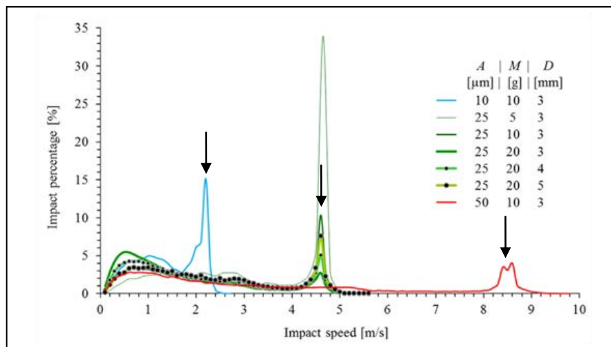
Figure 1.26 Distribution des vitesses des billes en fonction des paramètres de grenailage ultrasonique avec A l'amplitude de vibration, M la masse de billes insérée et D le diamètre des billes [Badreddine et al. - 2014]
