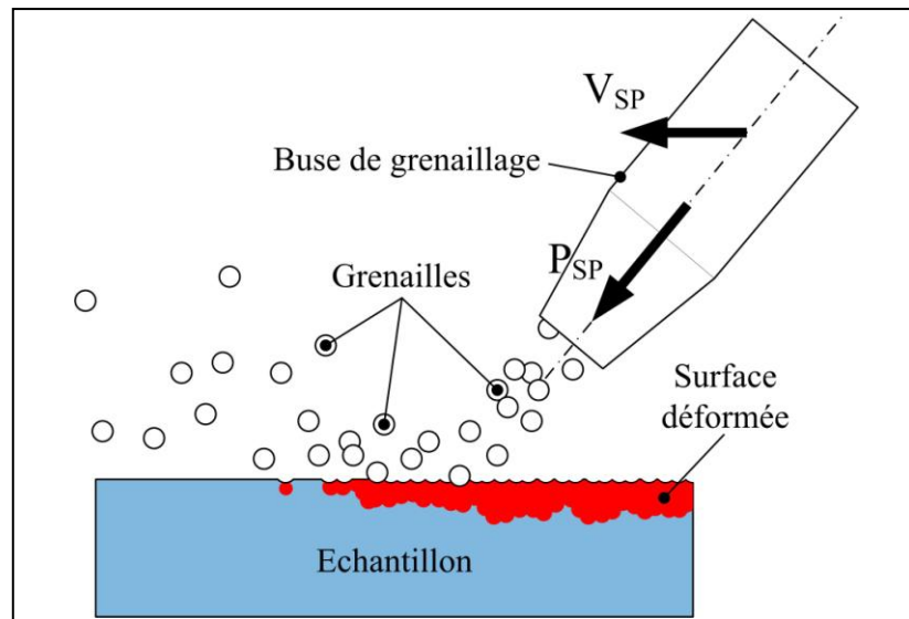
Figure 1.21 Schéma du traitement de grenailage de précontrainte traditionnel.
