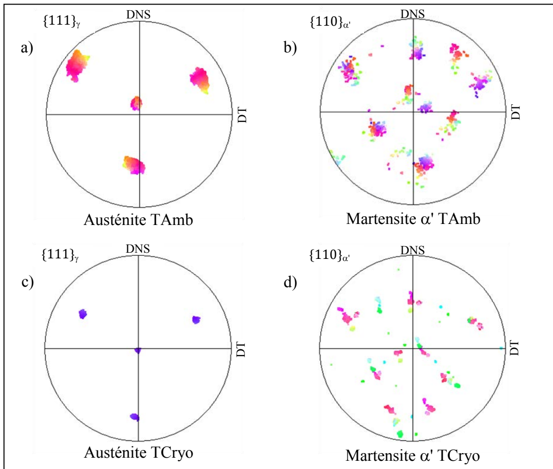
Figure 3.15 Comparaison entre des FDPs \{111\} de l'austénite et \{110\} martensite \alpha' obtenues en sous-couche des échantillons de 304L traités à température ambiante et sous condition cryogénique pour des orientations cristallines comparables. Les axes sur les FDPs représentent la Direction Normale à la Surface traitée (DNS) et la Direction Transverse (DT)
