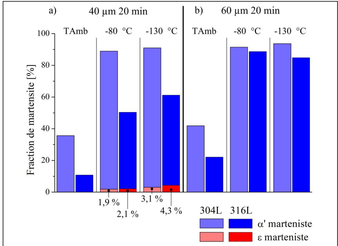
Figure 4.18 Fractions de martensites en surface obtenues par DRX pour les alliages 304L et 316L a) pour amplitude de 40 \mu\text{m} et b) pour une amplitude de 60 \mu\text{m} . L'erreur globale estimée pour ces mesures est de \pm 2\%
