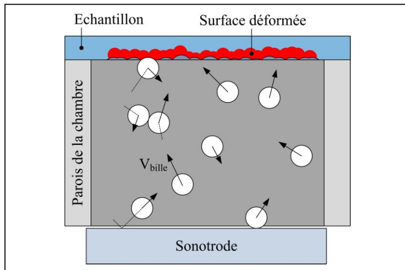
Figure 1.23 Schéma du traitement de grenailage ultrasonique
