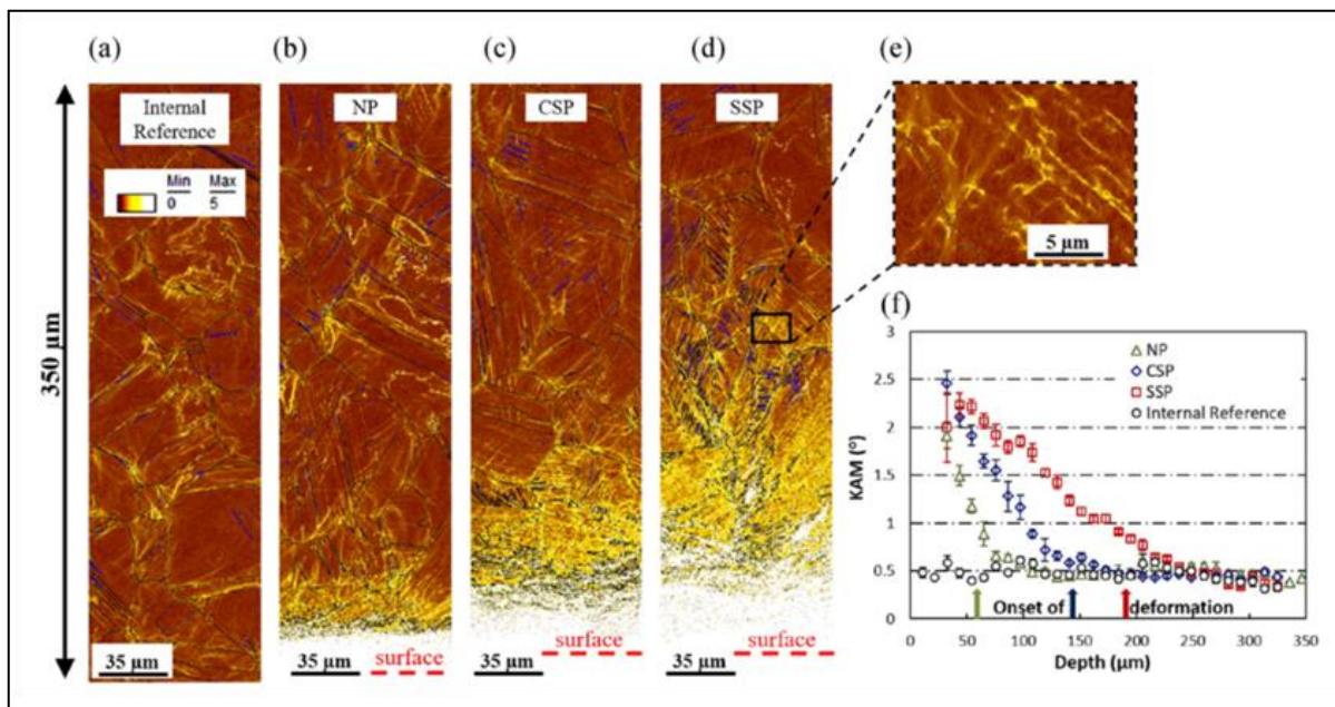
Figure 1.22 Comparaison des microstructures de sous-couche obtenues avant (NP) et après traitement de grenailage conventionnel (CSP) et de grenailage sévère (SSP) sur un alliage 316L. Une cartographie de référence à cœur est donnée en Figure 1.22a et les distributions des désorientations locales (KAM) associées aux différentes cartographies d'orientation sont données par les auteurs en Figure 1.22f [Bagherifard et al. - 2016]
