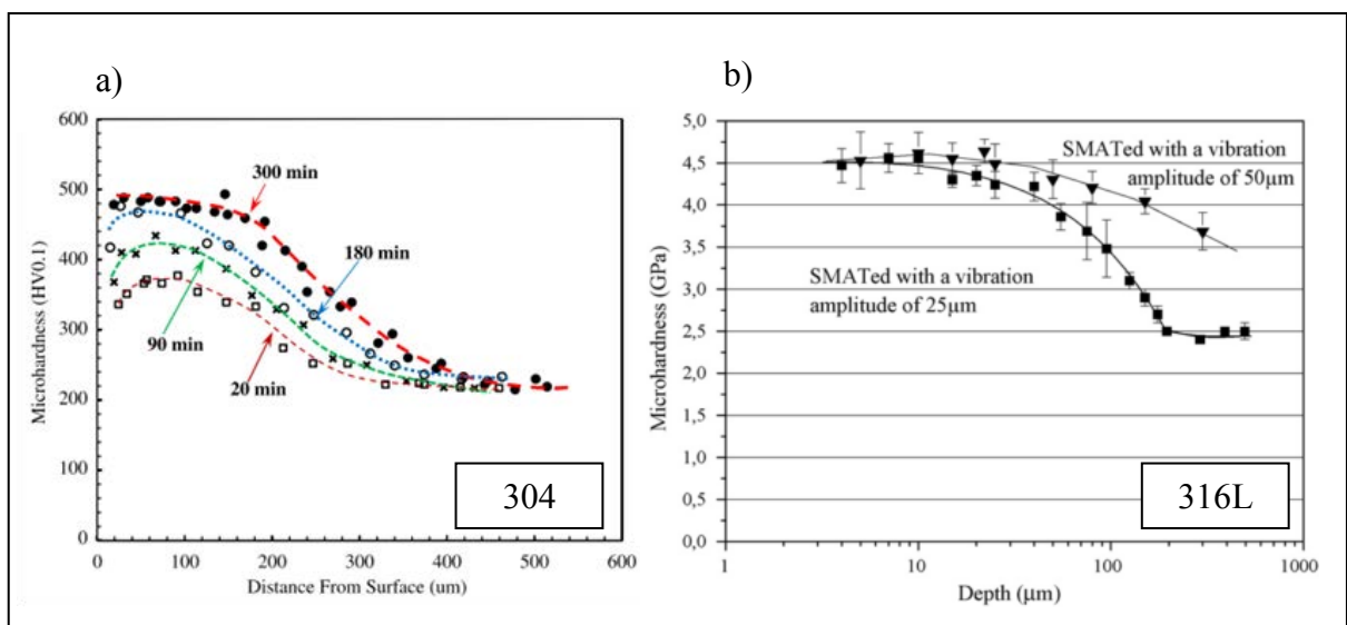
Figure 1.29 Profils de dureté obtenus après traitement de grenailage ultrasonique en fonction de a) la durée de traitement sur un alliage 304 [Sun - 2013] et b) de l'amplitude de traitement sur un alliage 316L [Roland et al. - 2007]
