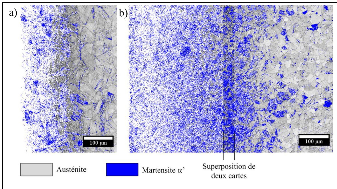
Figure 4.7 Distributions des phases en sous-couches des échantillons 304L a) 60 \mu m 20min T Amb et b) 60 \mu m 20min -130 °C observées par cartographie d'orientation
