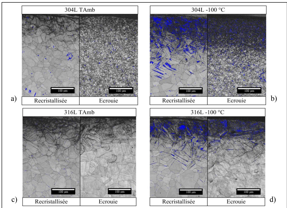
Figure 5.2 Cartographies d'orientation EBSD réalisées sur les sections transverses des alliages 304L et 316L grenailés a-c) à température ambiante et b-d) sous condition cryogénique. L'austénite est représentée en contraste de bande et la martensite \alpha' en bleu
