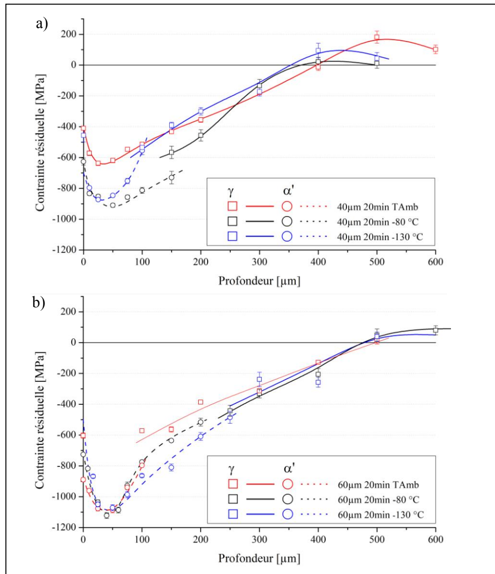
Figure 4.21 Profils des contraintes résiduelles obtenus sur l'alliage 316L pour les trois températures (TAmb, -80\text{ }^\circ\text{C} et -130\text{ }^\circ\text{C} ) sous une amplitude de a) 40 \mu\text{m} et b) 60 \mu\text{m}
