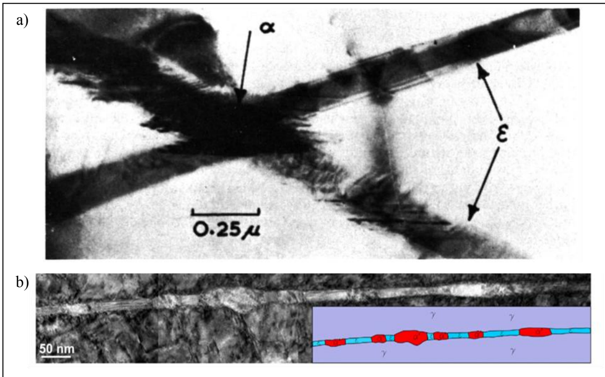
Figure 1.9 Exemple de la germination de martensite \alpha a) à l'intersection de deux bandes de martensite \epsilon [Venables - 1961] et b) à l'intérieur d'une bande unique de martensite \epsilon [Yang, Sun et Zhang - 2015]. L'austénite \gamma est ici représentée en gris, la martensite \epsilon en bleu et la martensite \alpha' en rouge sur le schéma inséré
