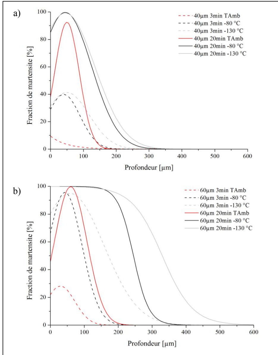
Figure 4.10 Distribution de martensite pour les différentes conditions de traitement réalisées sur l'alliage 304L avec a) une amplitude de 40 μm et b) une amplitude de 60 μm
