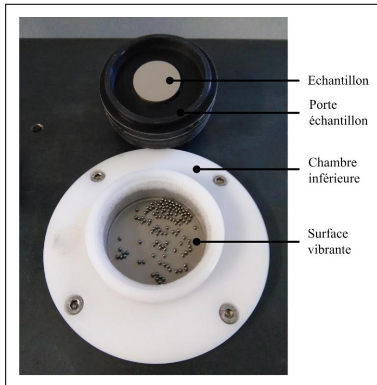
Figure 2.2 Photographie d'une vue globale du dispositif de grenailage ultrasonique destiné au traitement d'échantillons plats
