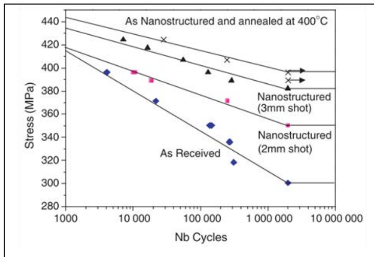
Figure 1.35 Courbe de Wöhler d'un alliage 316L traité par grenailage ultrasonique [Roland et al. - 2006]
