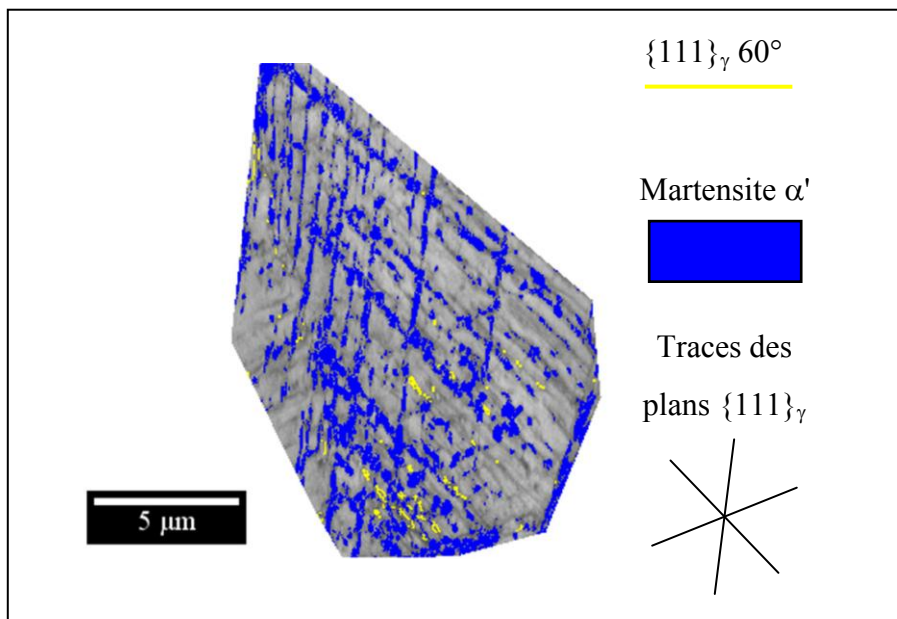
Figure 3.11 Cartographie d'orientation EBSD à fort grandissement d'un grain sélectionné sur la carte présentée en Figure 3.10 L'austénite est représentée en contraste de bande, les relations d'orientation de macle \{111\}_\gamma 60^\circ en jaune et la martensite \alpha' en bleu.
