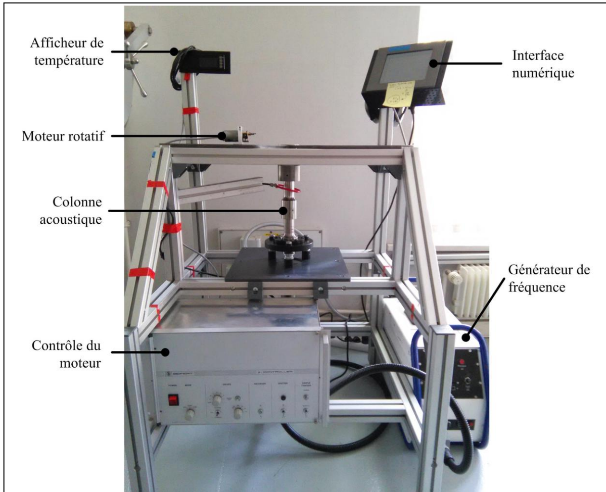
Figure 2.1 Photographie d'une vue d'ensemble du dispositif de grenailage ultrasonique
