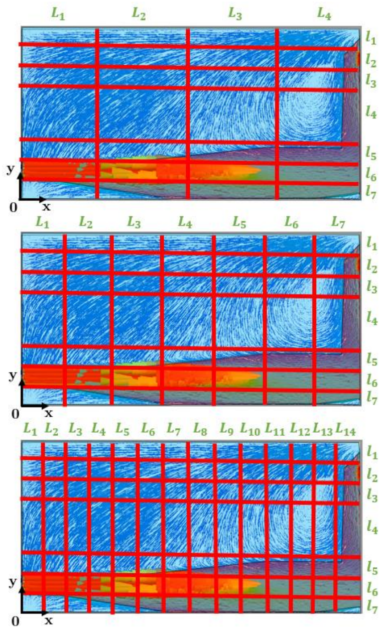
Figure III-20 : Champ de vitesse dans le plan horizontal ( Oxy ) à la surface libre en z = 47 cm. Surlignage rouge : fortes vitesses. Surlignage bleu : faibles vitesses. Traits rouges : découpage des compartiments. EN HAUT : N_L = 4 . AU MILLIEU : N_L = 7 . EN BAS : N_L = 14 .
