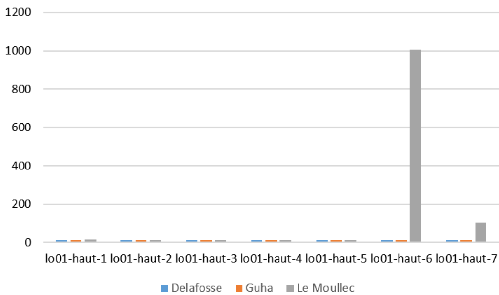
Figure III-45 : Débits turbulents exprimés en pourcentage du débit convectif dans le plan lo01 sur les compartiments de la couche de surface (haut) sur chacune des subdivisions dans la largeur (1 à 7).
