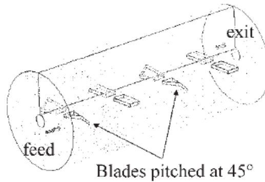
Figure I-25 : Schéma d'un réacteur de production de polyéthylène basse densité, (Wells and Ray, 2005).
