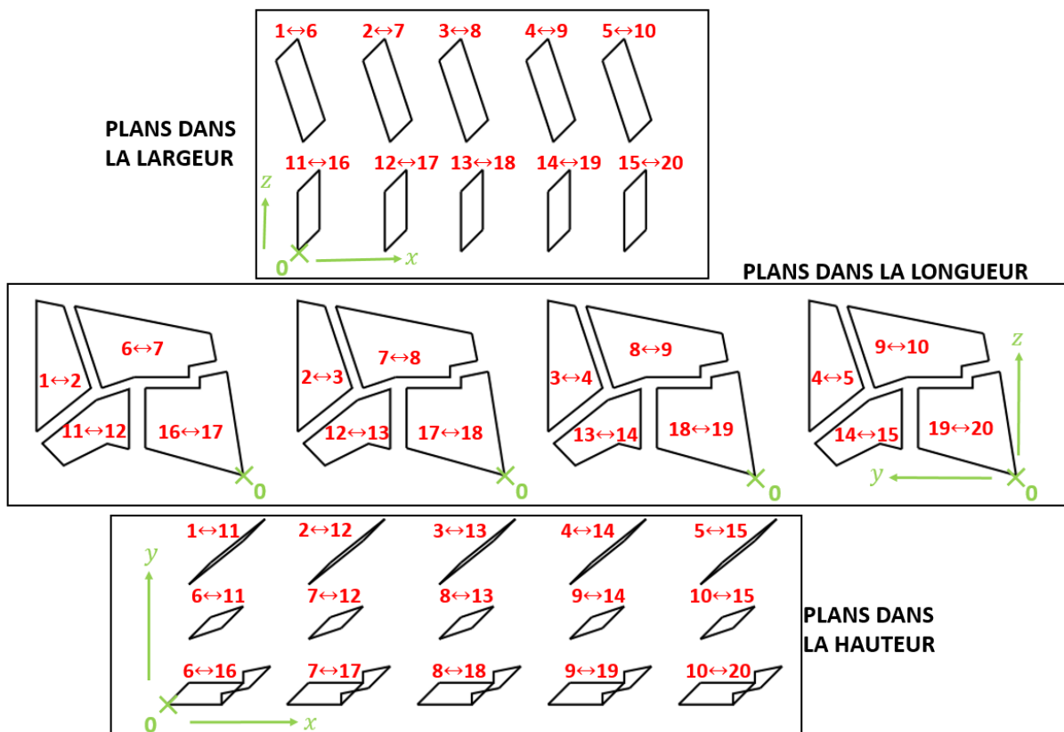
Figure II-25 : Classement des surfaces d'échanges selon des plans dans la largeur, longueur et hauteur d'après le modèle de la Figure II-24.
