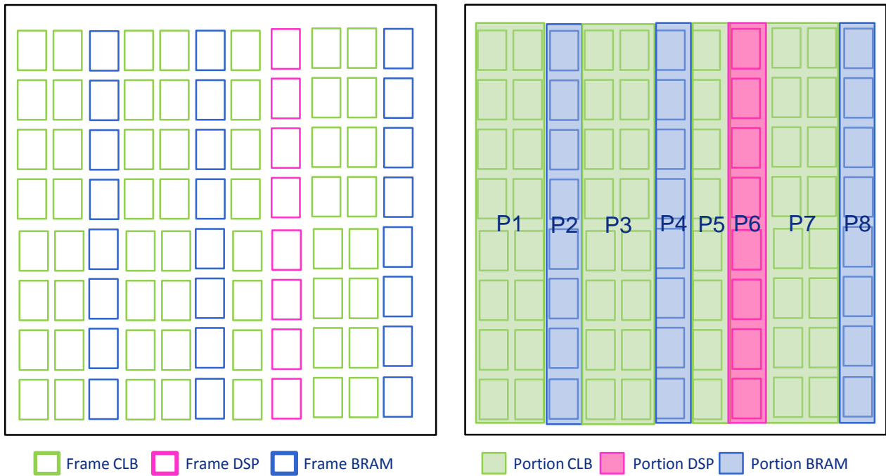
FIGURE 3.5 – Une architecture hétérogène simplifiée
