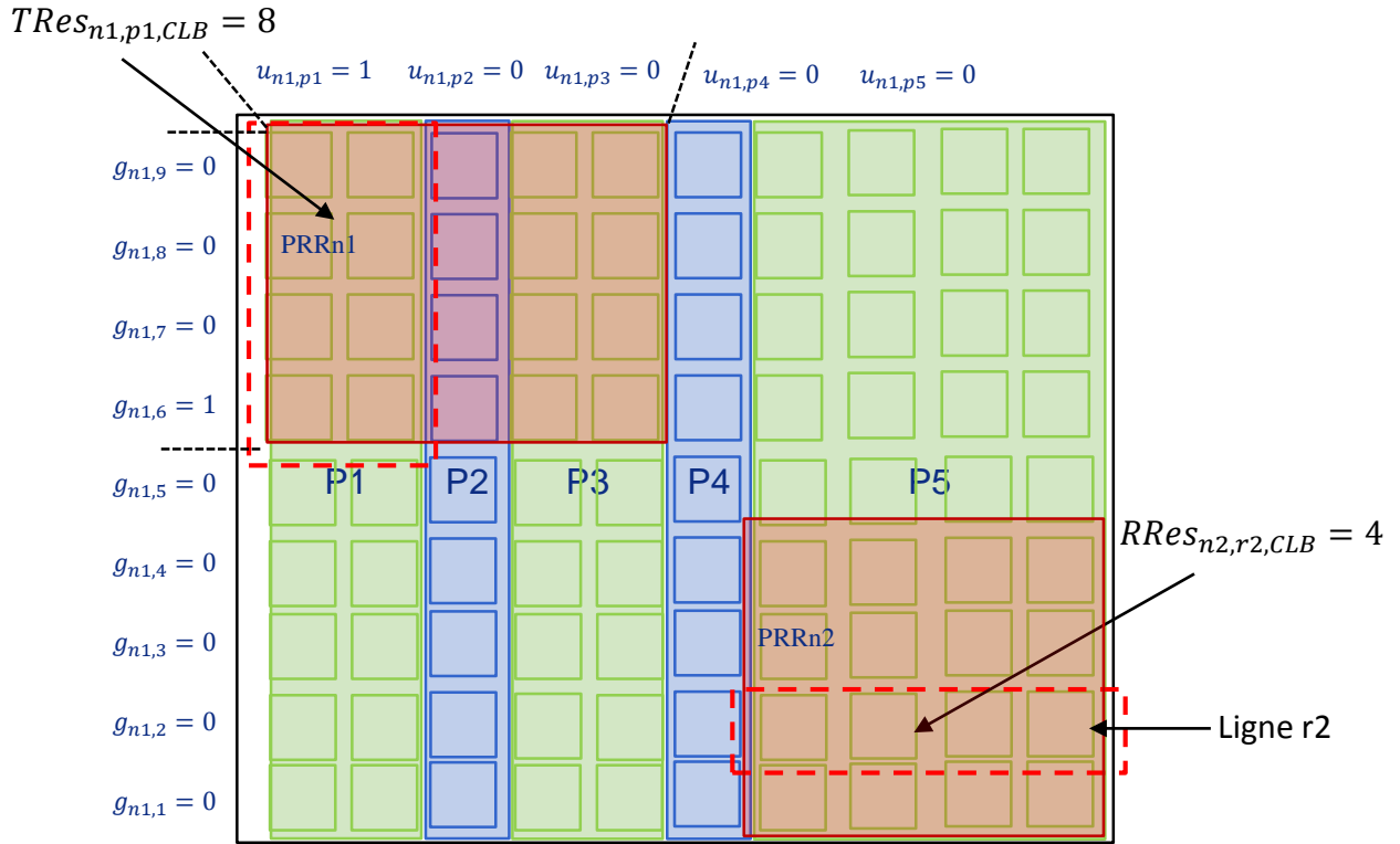
FIGURE 4.2 – Calcul des ressources couvertes : TRes_{n,p,t} et RRes_{n,r,t}
