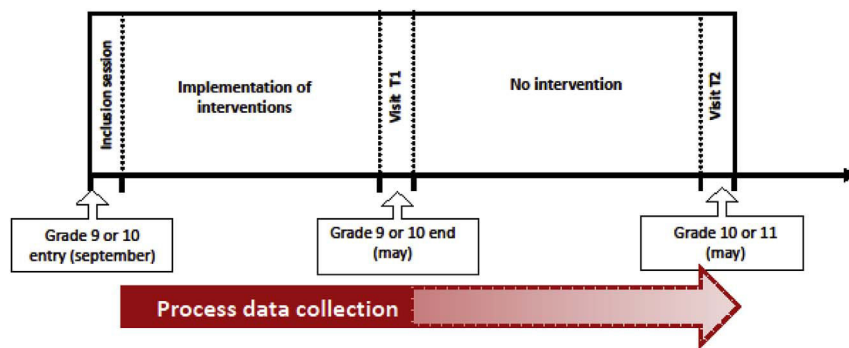
Fig. 1. PRALIMAP-INÈS implementation.
