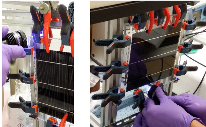
Figure 4-4 - A gauche, scellement du haut de l'assemblage, à l'aide d'une lampe UV portable. A droite, scellement de l'entrée de l'encapsulant au niveau de l'aiguille de remplissage.
