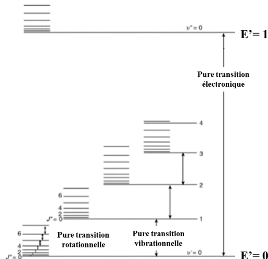
Figure 2-1 - Niveau d'énergie d'une molécule diatomique (l'échelle énergétique est purement schématique, l'espace relatif entre chaque transition est théoriquement bien plus grand) [59].
