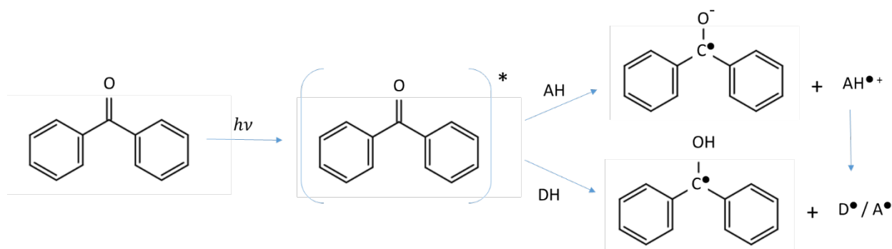
Figure 1-28 - Formations de radicaux libres d'un photoamorceur radicalaire de type II : exemple de la benzophénone [57].
