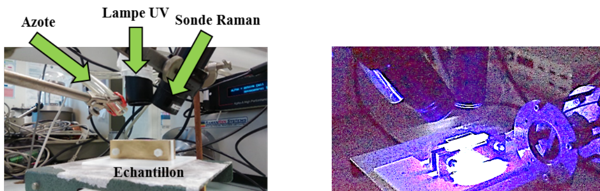
Figure 4-17 - A gauche, montage expérimental pour le suivi cinétique de photopolymérisation par couplage in situ de la spectroscopie Raman et de l'analyse diélectrique. A droite, le système en cours de mesure sous irradiation UV.
