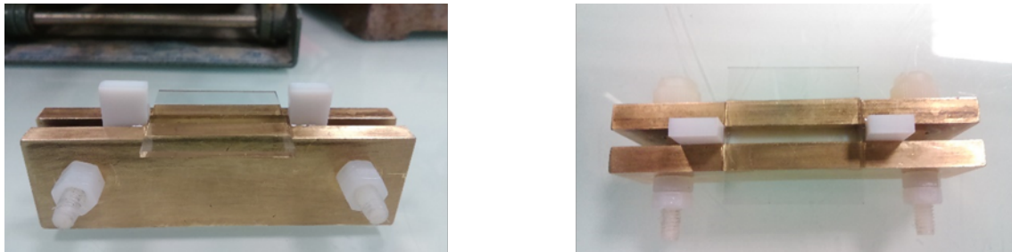
Figure 4-16 - Cellule de mesure pour le suivi cinétique de photopolymérisation par spectroscopie Raman couplée aux analyses diélectriques.
