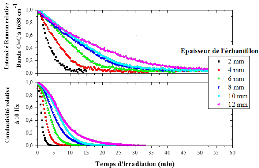
Figure 4-20 - Suivi cinétique de la photopolymérisation de la formulation F15 par diminution de l'intensité de la bande spectrale Raman C=C à 1638 cm -1 (en haut) et par diminution de la conductivité à 10 Hz (en bas).
