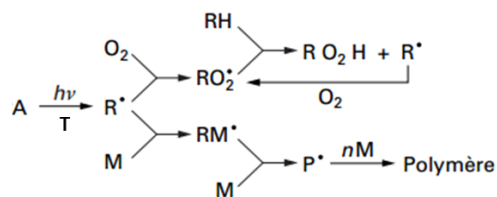
Figure 1-15 – Effet inhibiteur de l’oxygène lors de la polymérisation radicalaire [23]. A est l’amorceur, et M le monomère.
