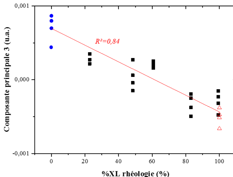
Figure 3-42 – Variations des scores de la CP-3 de chacun des échantillons en fonction de leur degré de réticulation évalué par rhéologie.
