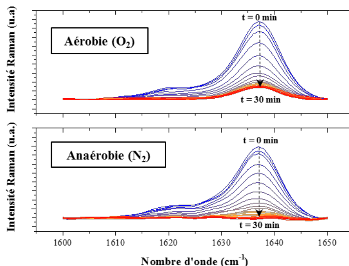
Figure 4-13 – Evolution de la bande spectrale Raman liée à la liaison C=C du monomère pour la formulation F5 à 1638\text{ cm}^{-1} en fonction du temps d'irradiation UV (du bleu t = 0\text{ min} au rouge t = 30\text{ min} ). En haut, système en présence d' \text{O}_2 . En bas, système en absence d' \text{O}_2 .
